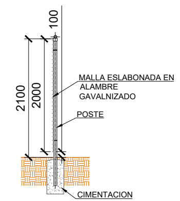
VALLADO MALLA ESLABONADA EN ALAMBRE PERFIL TIPO ESCALA 1: 75
