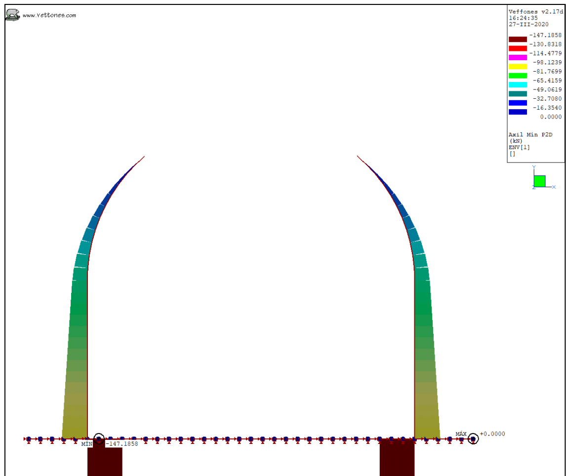
Ilustración 15. Envolvente ELS, K30 = 100 kgf/cm3. Sección Pico Flauta. Nominal mínimo.
