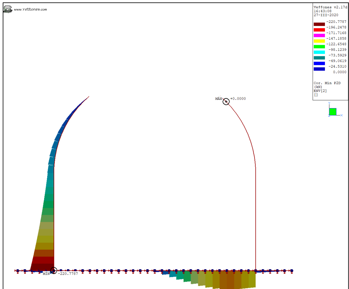
Ilustración 20. Envolvente ELU, K30 = 100 kgf/cm 3 . Sección Pico Flauta. Cortante mínimo.
