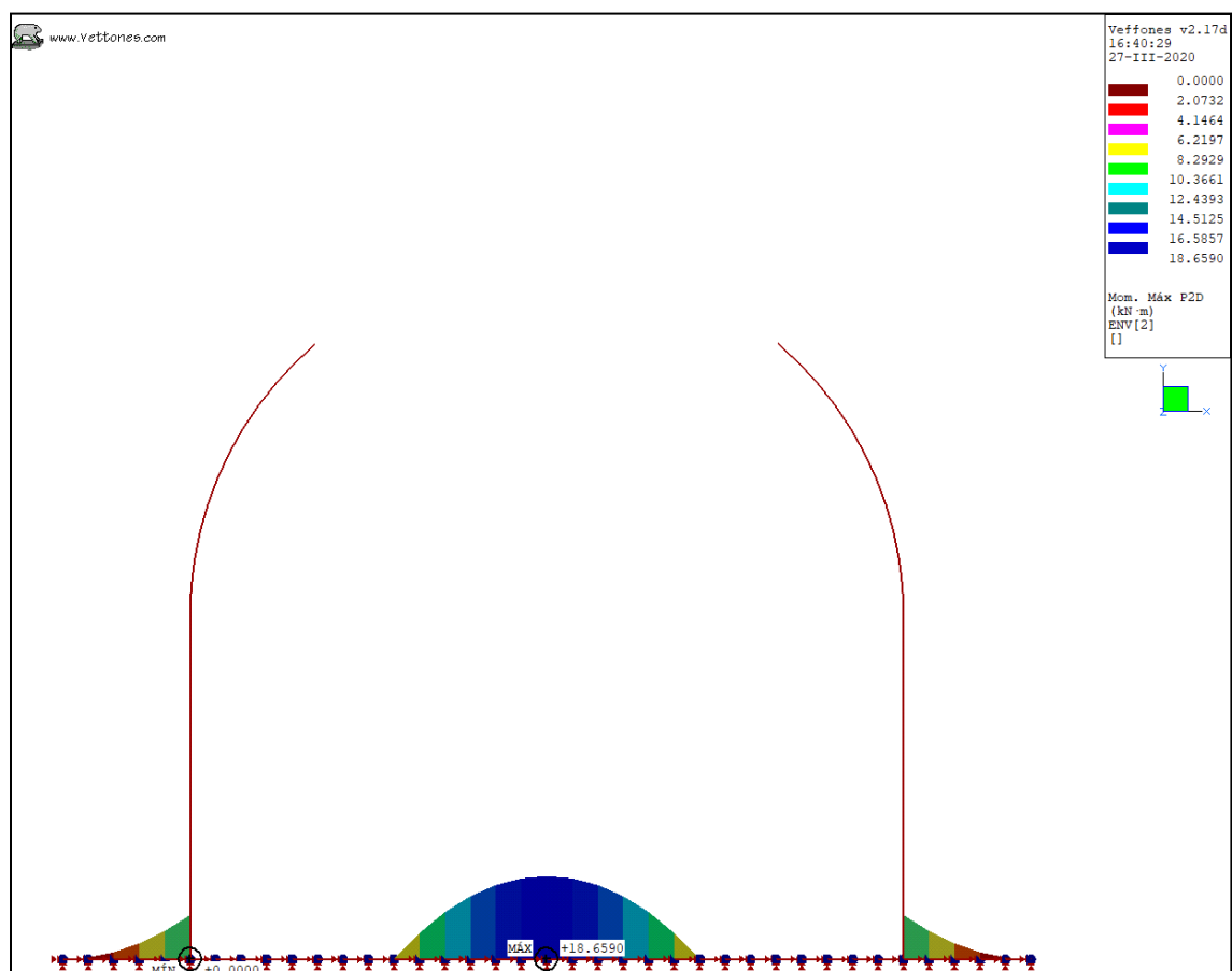
Ilustración 16. Envoltura ELU, K30 = 100 kgf/cm 3 . Sección Pico Flauta. Momento máximo.
