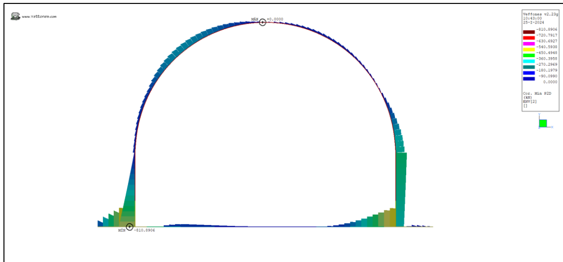
Ilustración 39. Cortante Min (kN)
