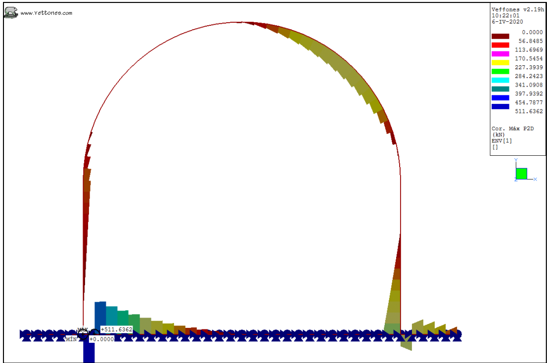
Ilustración 13. Envolvente ELS, K30 = 100 kgf/cm 3 . Cortante máximo.
