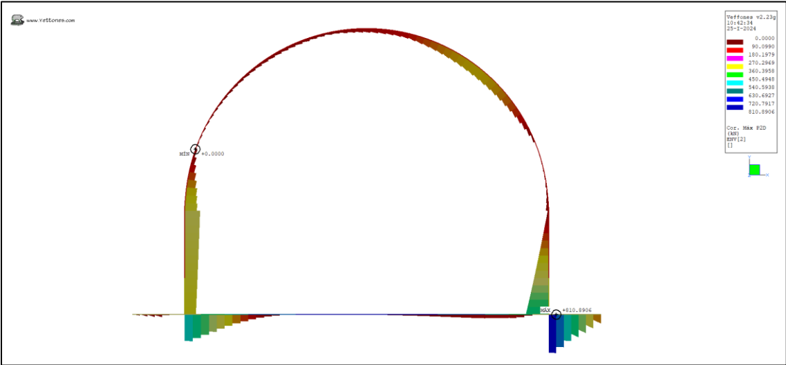
Ilustración 36. Cortante Max (kN)
