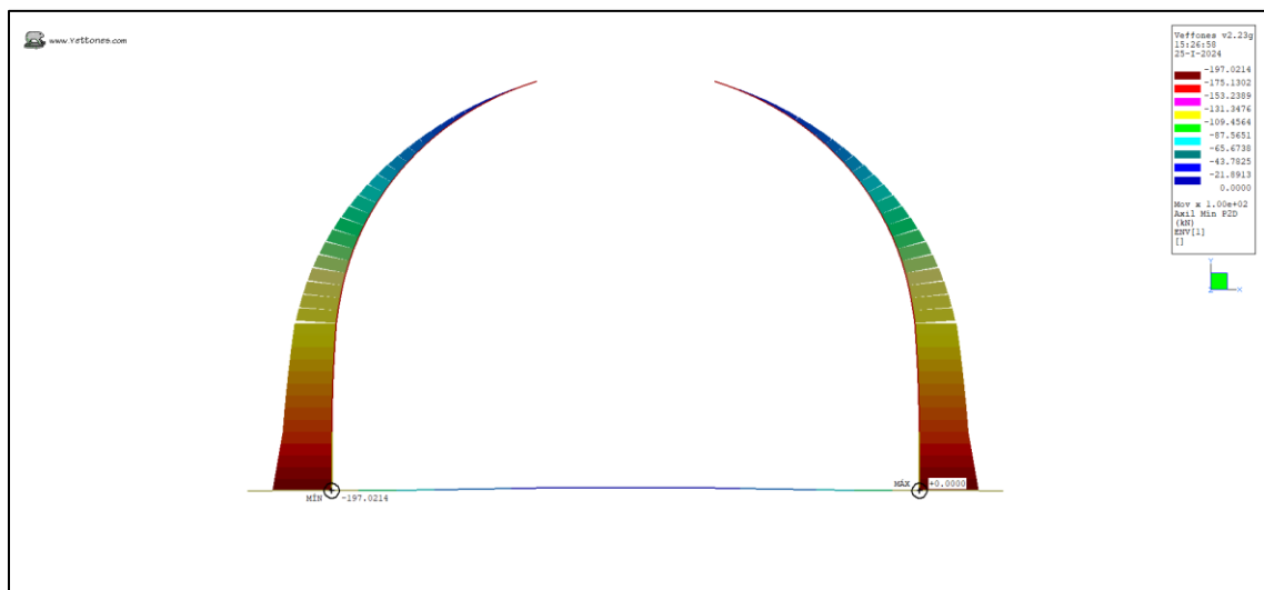
Ilustración 20. Axil Min (kN)
