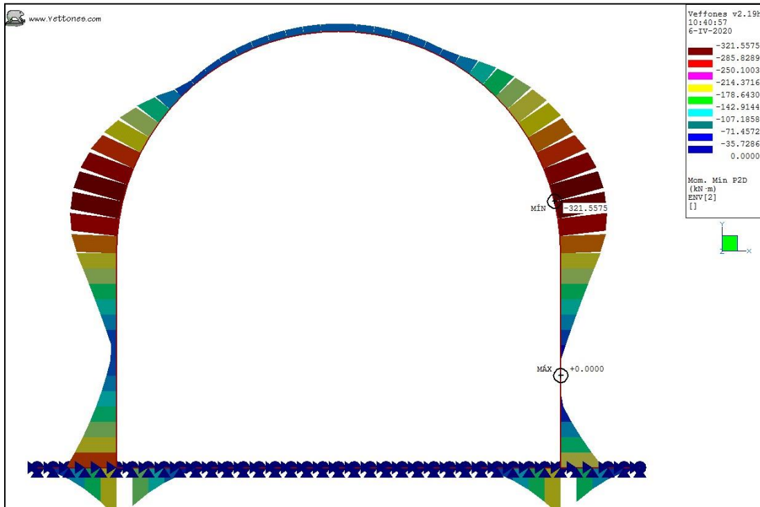
Ilustración 33. Envolvente ELU, K30 = 800 kgf/cm3. Momento mínimo.
