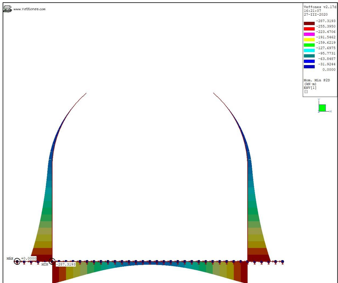
Ilustración 13. Envolvente ELS, K30 = 100 \text{ kgf/cm}^3 . Sección Pico Flauta. Momento mínimo.
