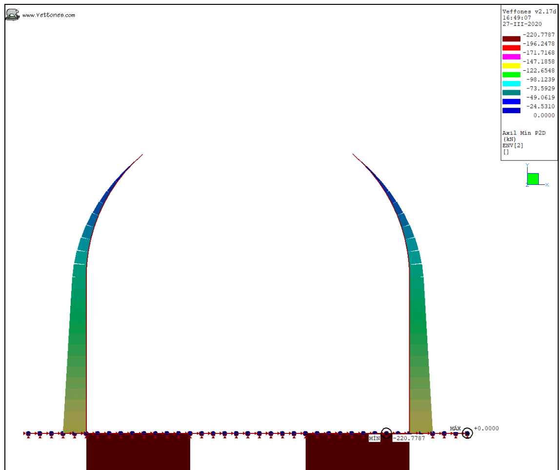
Ilustración 33. Envolvente ELU, K30 = 800 kgf/cm 3 . Sección Pico Flauta. Normal mínimo.
