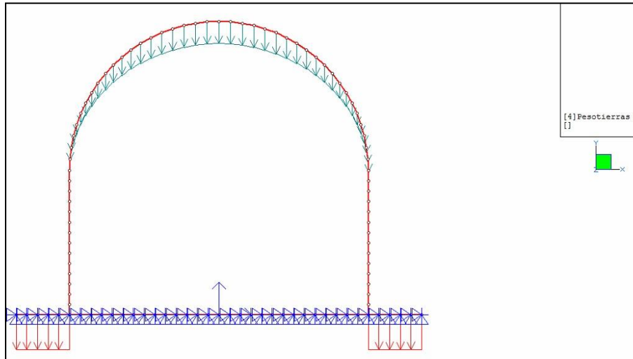
Ilustración 6 Carga vertical de tierras
