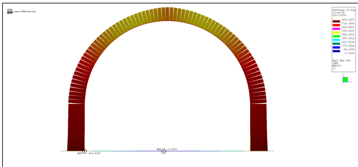
Ilustración 34. Axil Min (kN)
