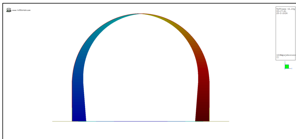
Ilustración 9. Acción -2 Empuje de tierras K_{a/2}
