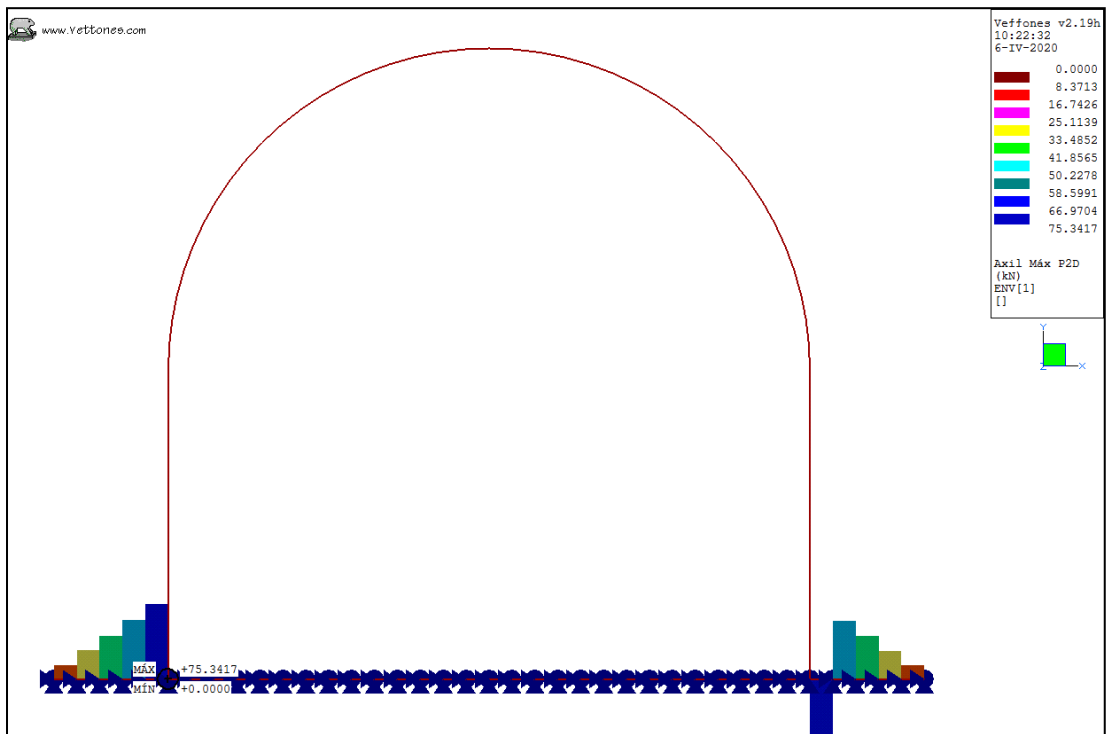
Ilustración 14. Envolvente ELS, K30 = 100 kgf/cm 3 . Normal máximo
