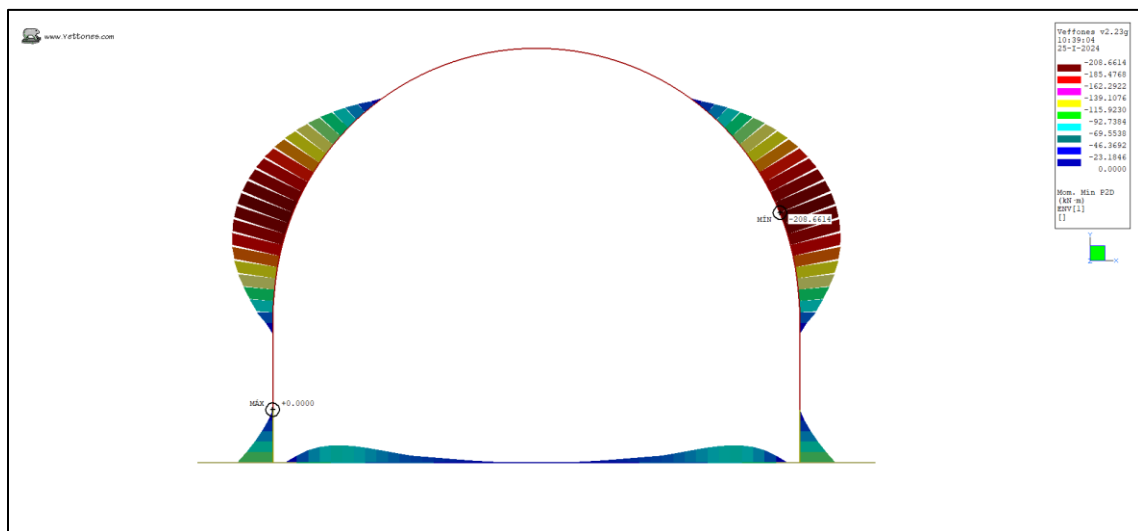
Ilustración 32. Momento Min (kN*m)
