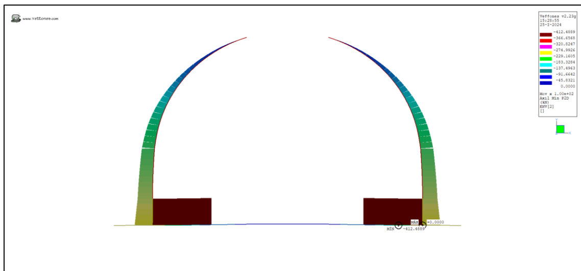
Ilustración 26. Axil Min (kN)
