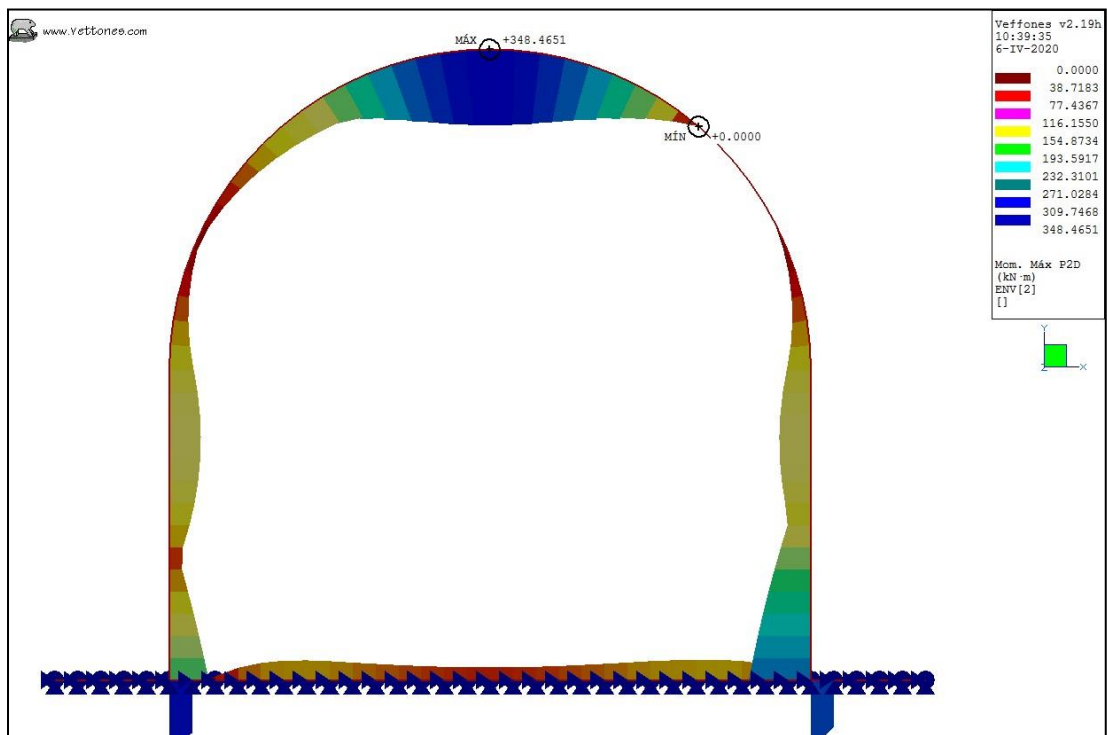
Ilustración 30. Envolvente ELU, K30 = 800 kgf/cm3. Momento máximo.
