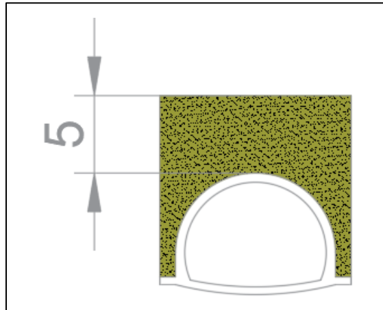
Ilustración 5. Esquema-Área del peso de tierras
