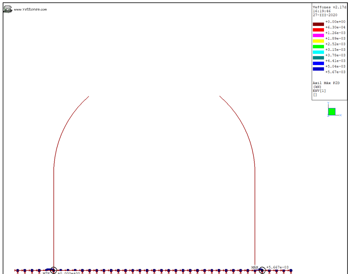
Ilustración 12. Envolvente ELS, K30 = 100 kgf/cm 3 . Sección Pico Flauta. Normal máximo
