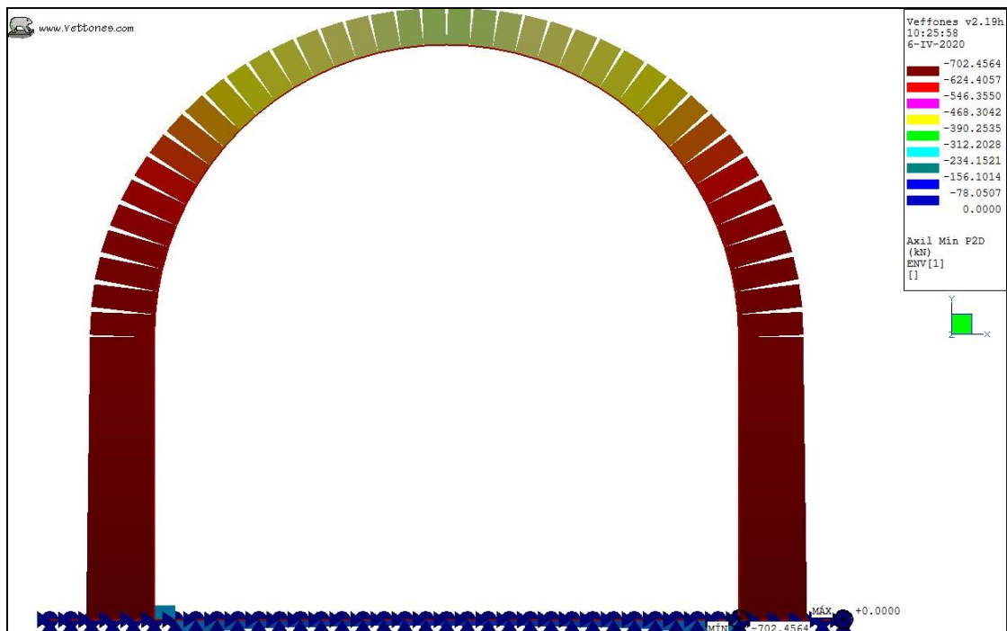
Ilustración 17. Envolvente ELS, K30 = 100 kgf/cm3. Nominal mínimo.
