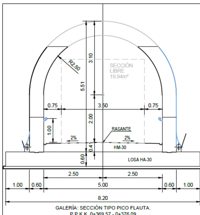
Ilustración 2 Falso túnel de galería. Pico Flauta
