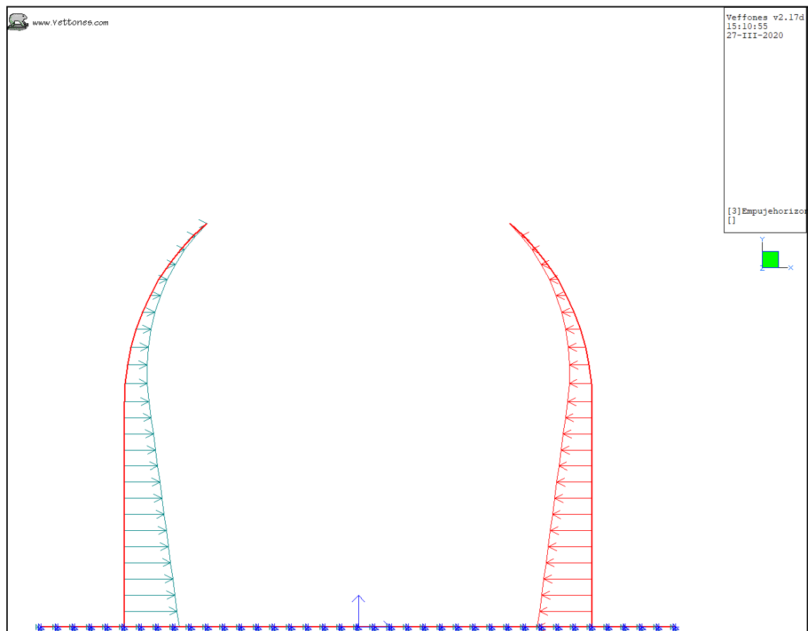
Ilustración 5. Empuje de tierras – Activo/2
