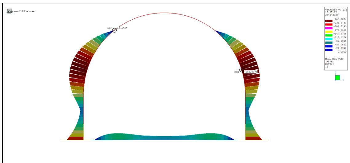
Ilustración 20. Momento Min (kN*m)
