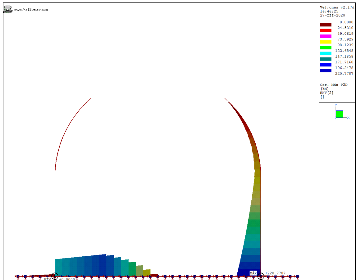
Ilustración 29. Envoltente ELU, K30 = 800 kgf/cm3. Sección Pico Flauta. Cortante máximo
