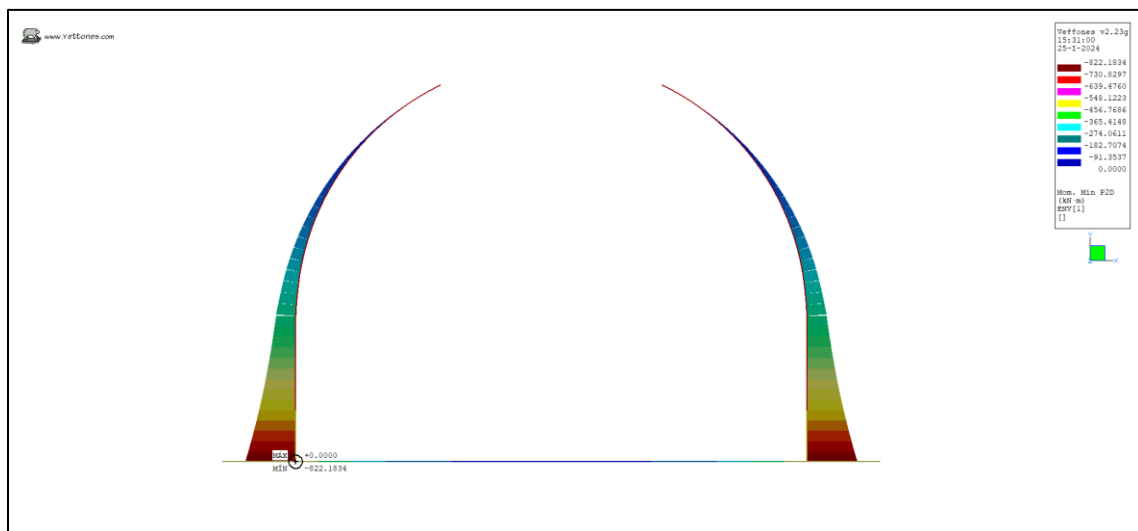
Ilustración 30. Momento Min (kN*m)
