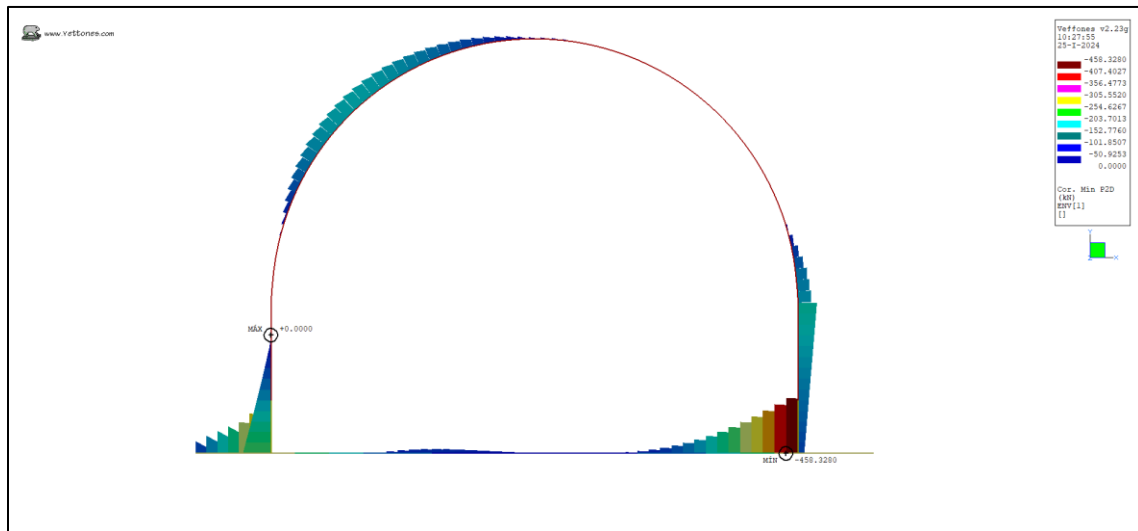
Ilustración 21. Cortante Min (kN)
