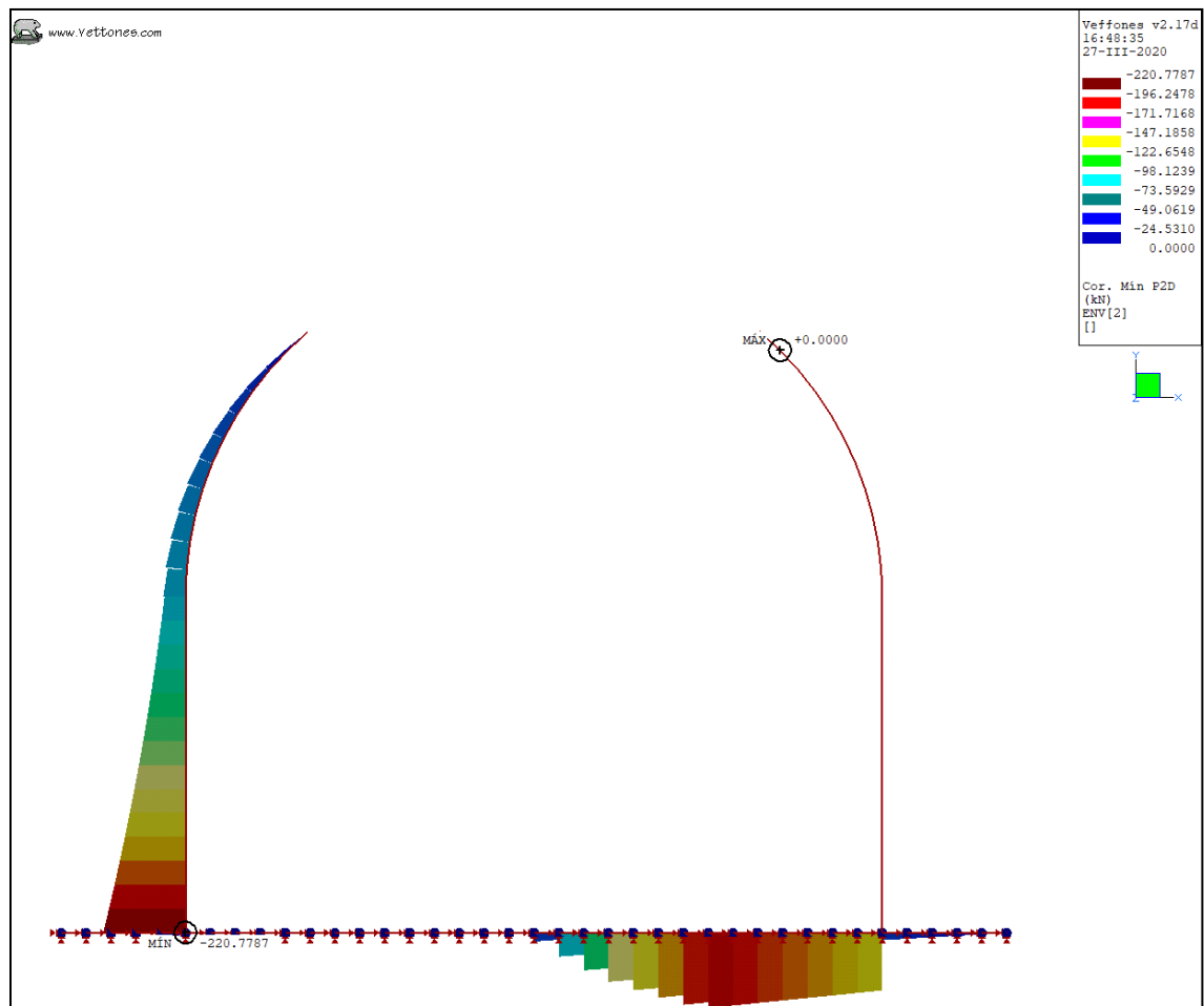
Ilustración 32. Envolvente ELU, K30 = 800 kgf/cm 3 . Sección Pico Flauta. Cortante mínimo.
