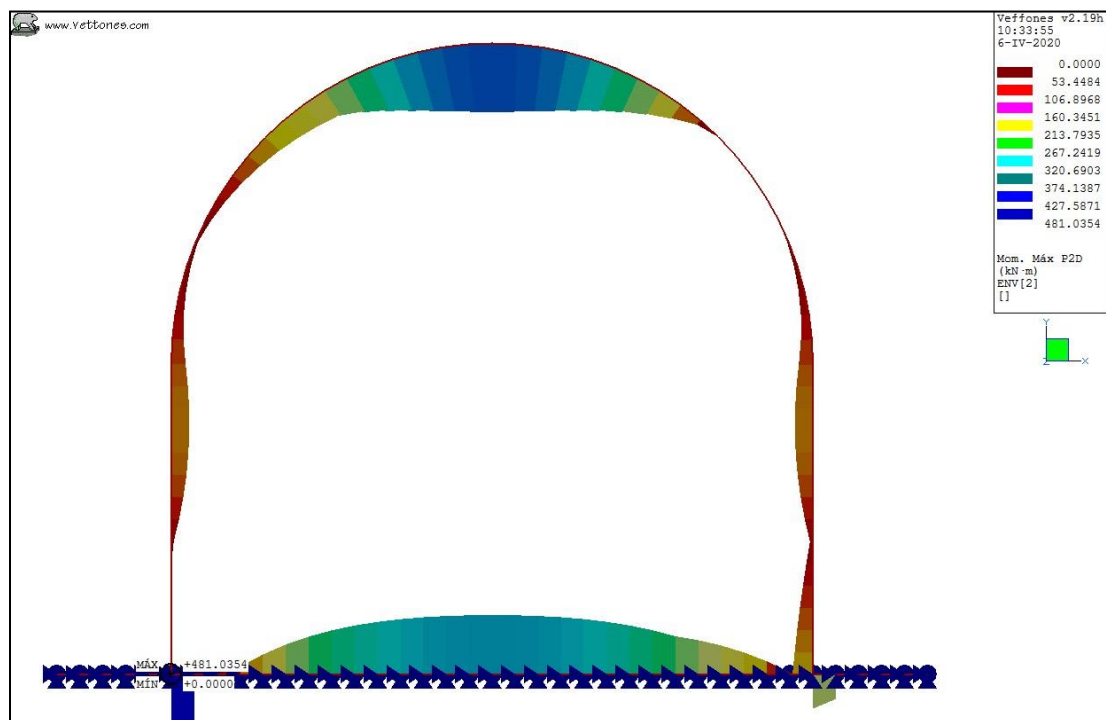
Ilustración 18. Envolvente ELU, K30 = 100 kgf/cm3. Momento máximo.
