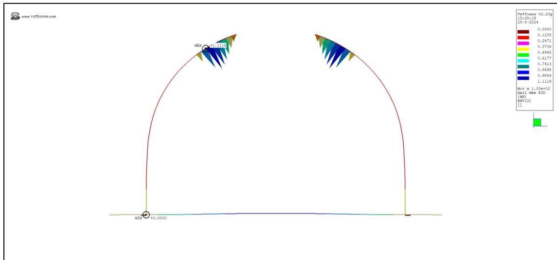
Ilustración 23. Axil Max (kN)
