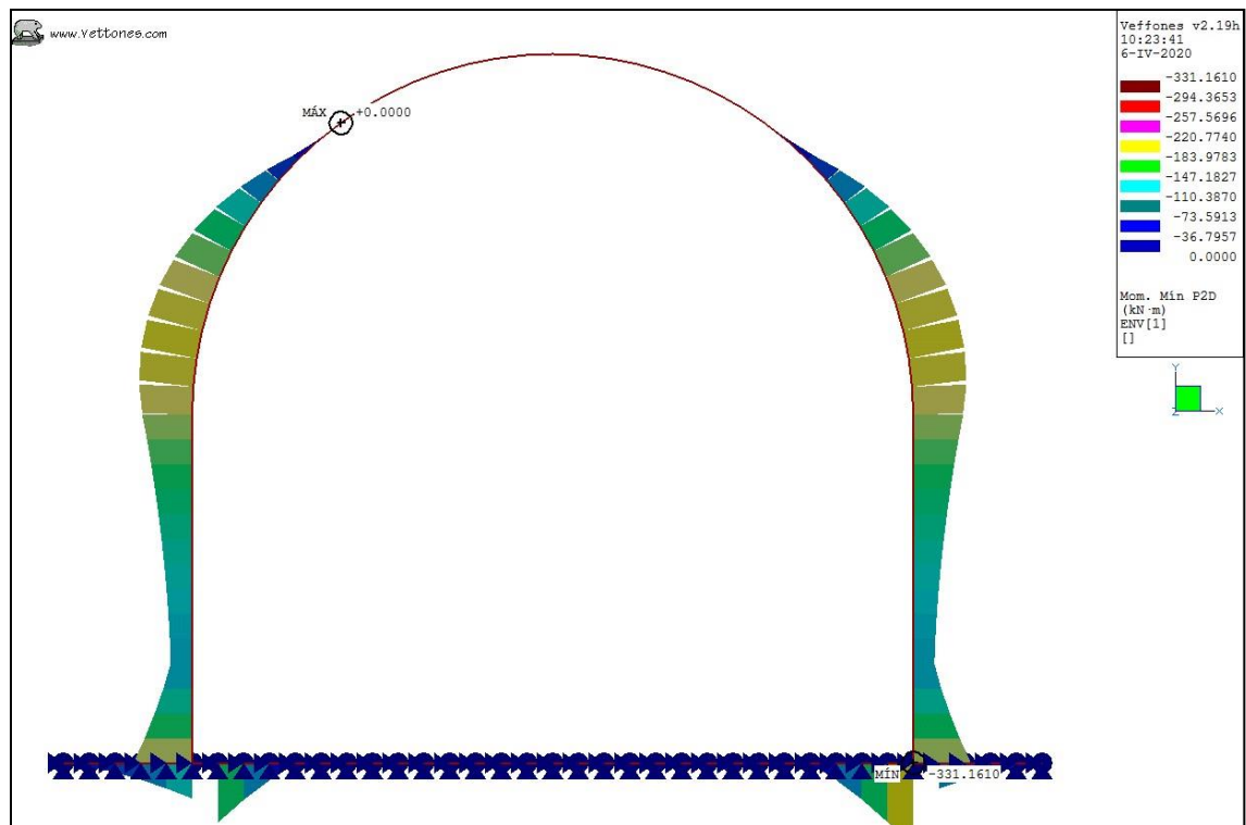
Ilustración 15. Envolvente ELS, K30 = 100 kgf/cm 3 . Momento mínimo.
