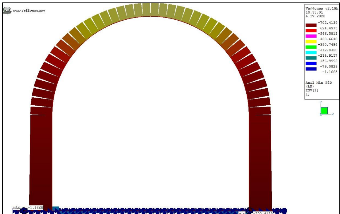
Ilustración 29. Envolvente ELS, K30 = 800 kgf/cm3. Normal mínimo.
