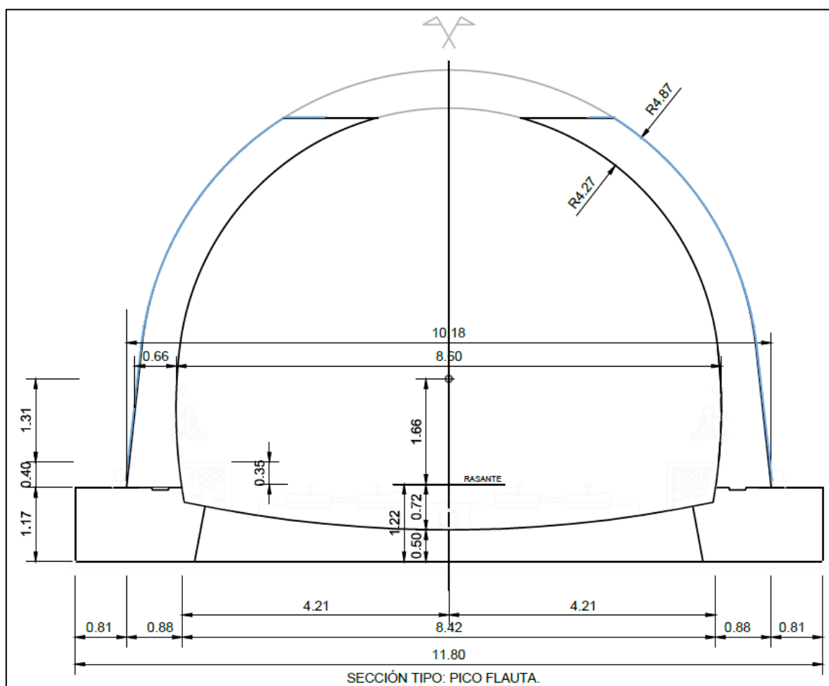
Ilustración 2 Pico de flauta
