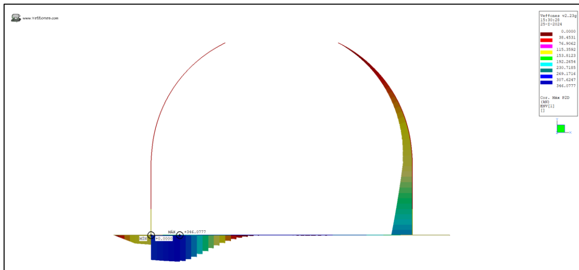
Ilustración 28. Cortante Max (kN)
