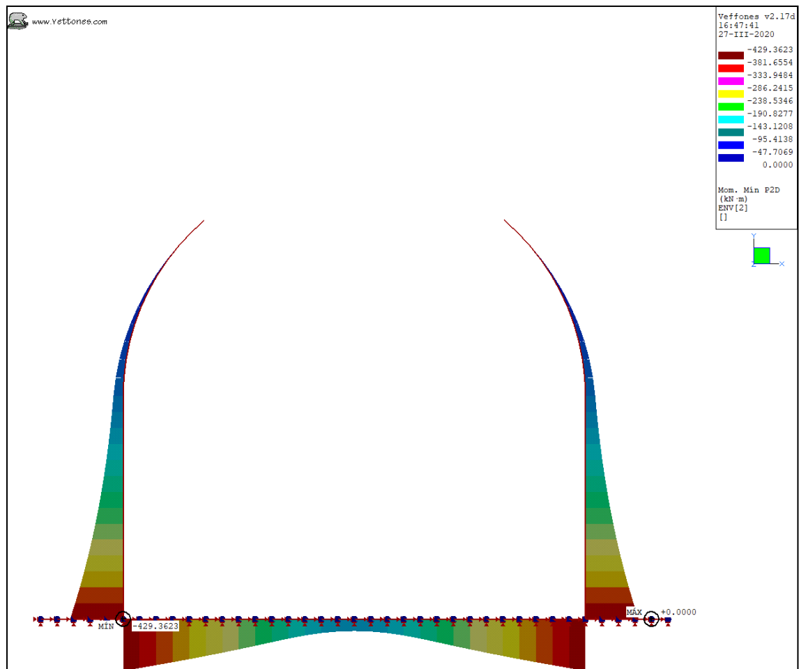
Ilustración 31. Envoltente ELU, K30 = 800 kgf/cm 3 . Sección Pico Flauta. Momento mínimo.
