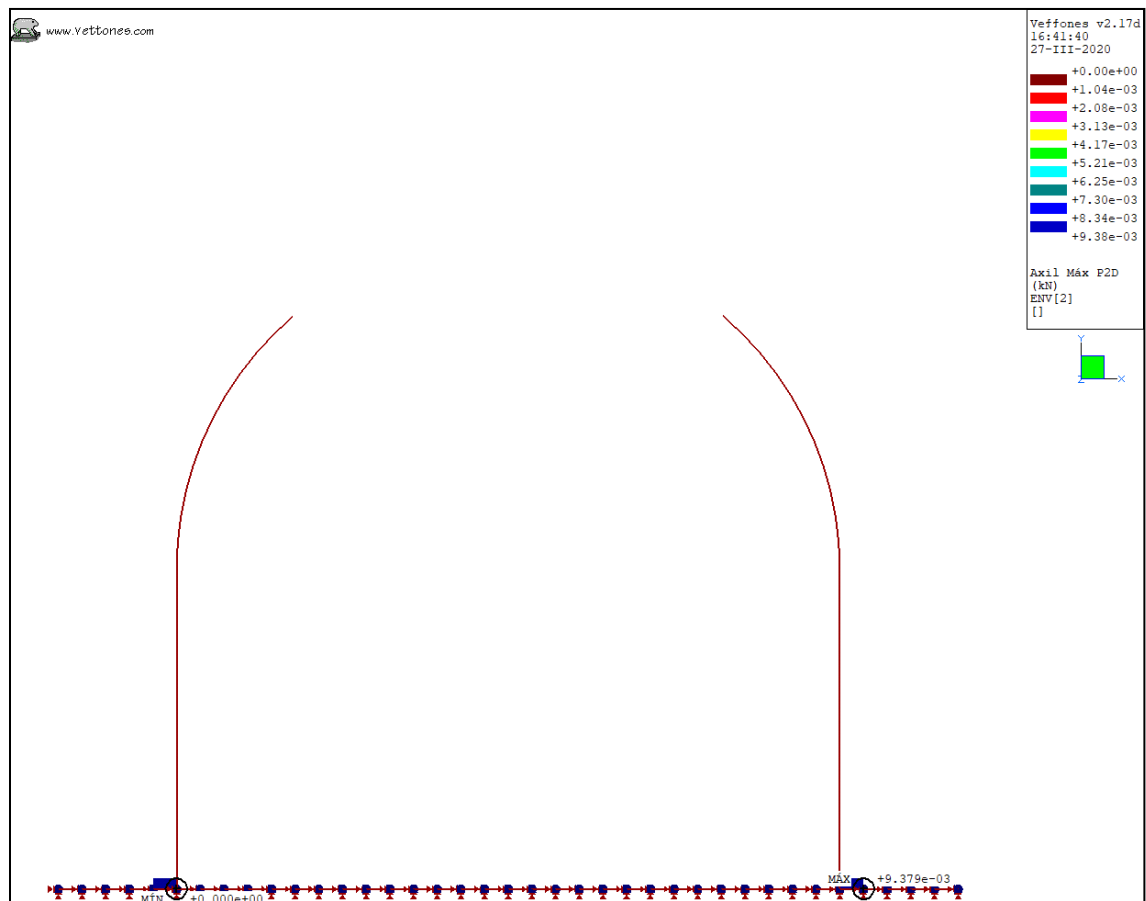
Ilustración 18. Envolvente ELU, K30 =100 kgf/cm 3 . Sección Pico Flauta. Normal máximo.
