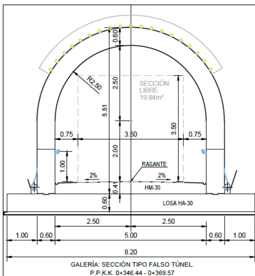
Ilustración 2 Falso túnel de galería
