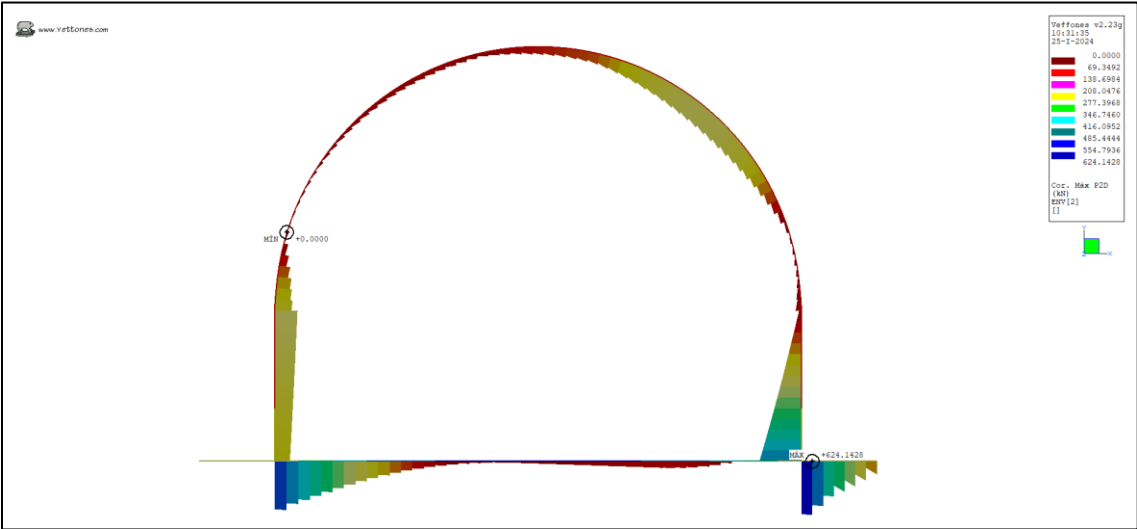
Ilustración 24. Cortante Max (kN)
