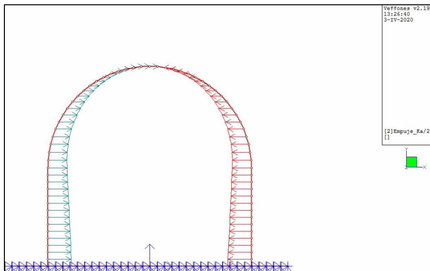
Ilustración 5. Empuje de tierras – Activo/2
