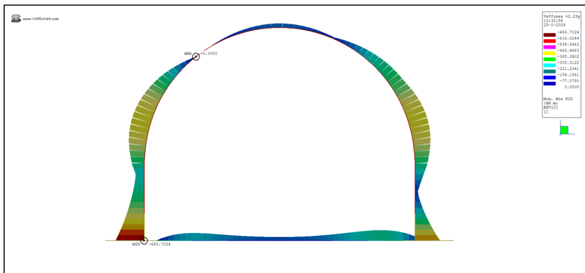
Ilustración 26. Momento Min (kN*m)
