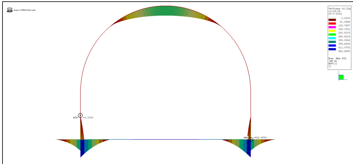
Ilustración 17. Momento Max (kN*m)
