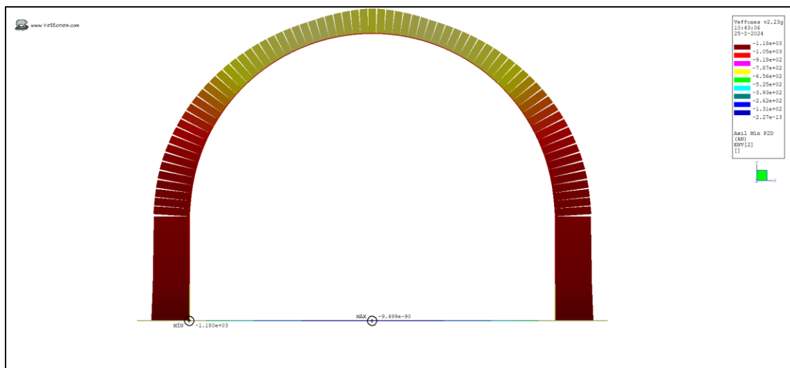
Ilustración 40. Axil Min (kN)
