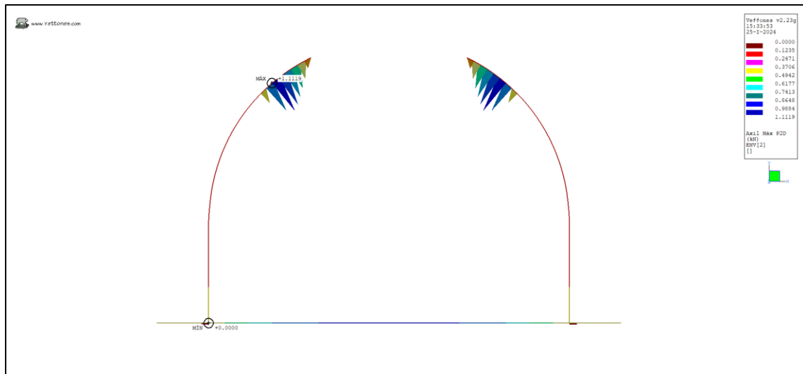
Ilustración 35. Axil Max (kN)
