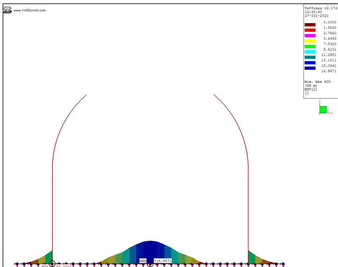
Ilustración 28. Envoltura ELU, K30 = 800 \text{ kgf/cm}^3 . Sección Pico Flauta. Momento máximo.
