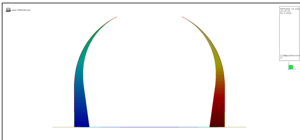
Ilustración 6. Acción – 1 Empuje de tierras K_0
