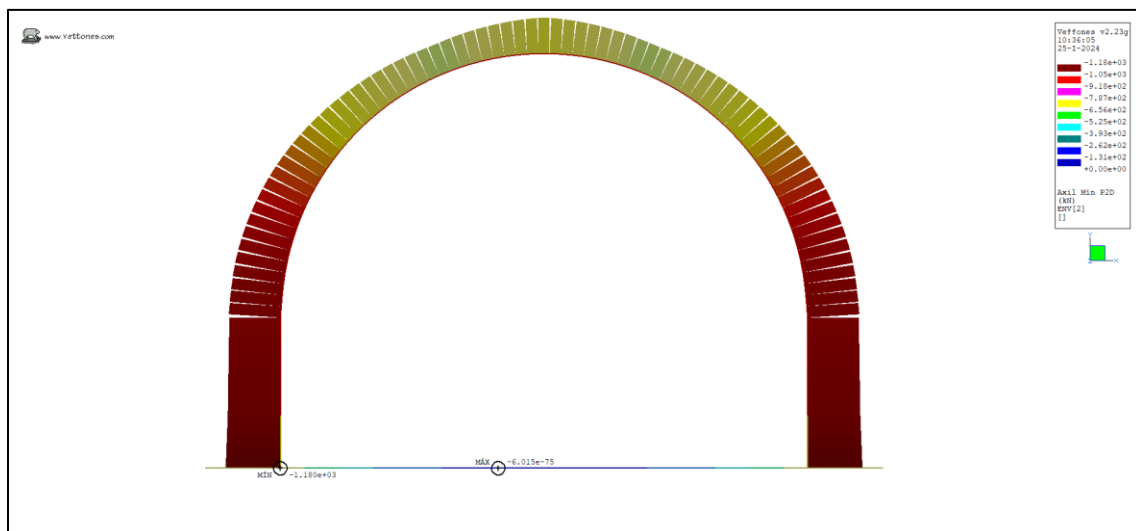
Ilustración 28. Axil Min (kN)
