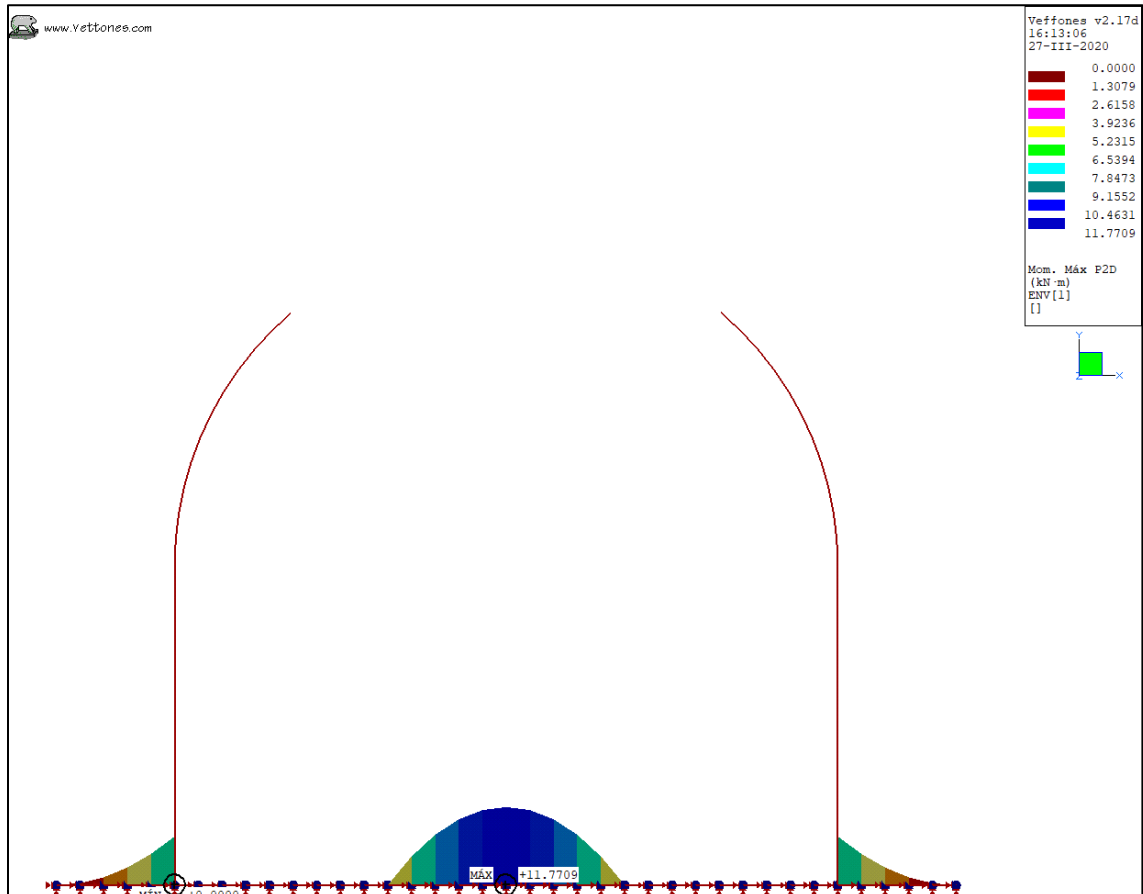
Ilustración 10. Envoltura ELS, K30 = 100 kgf/cm3. Sección Pico Flauta. Momento máximo.
