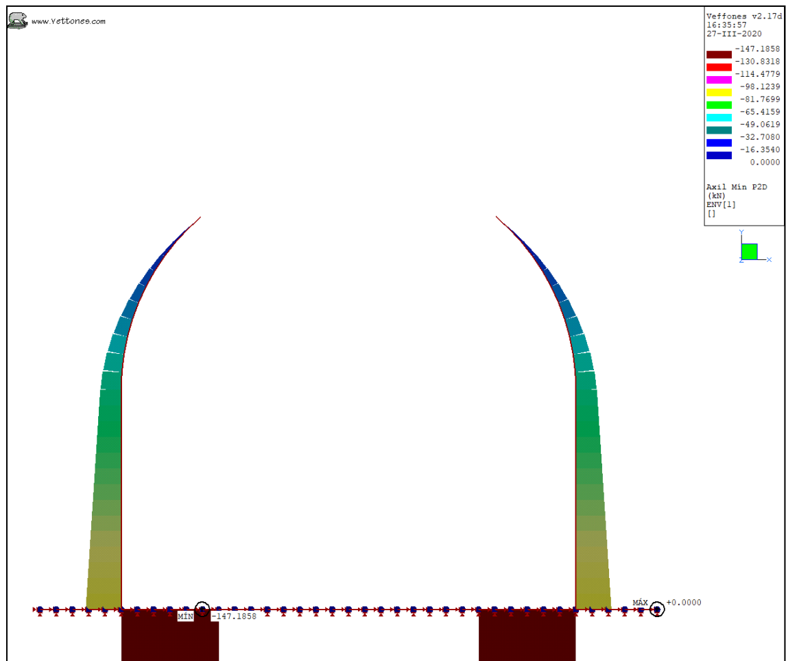
Ilustración 27. Envolvente ELS, K30 = 800 kgf/cm 3 . Sección Pico Flauta. Normal mínimo.
