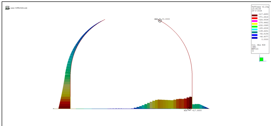
Ilustración 37. Cortante Min (kN)
