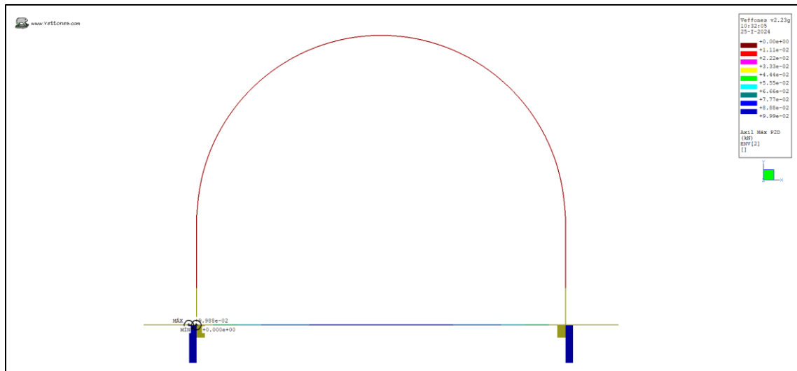
Ilustración 25. Axil Max (kN)
