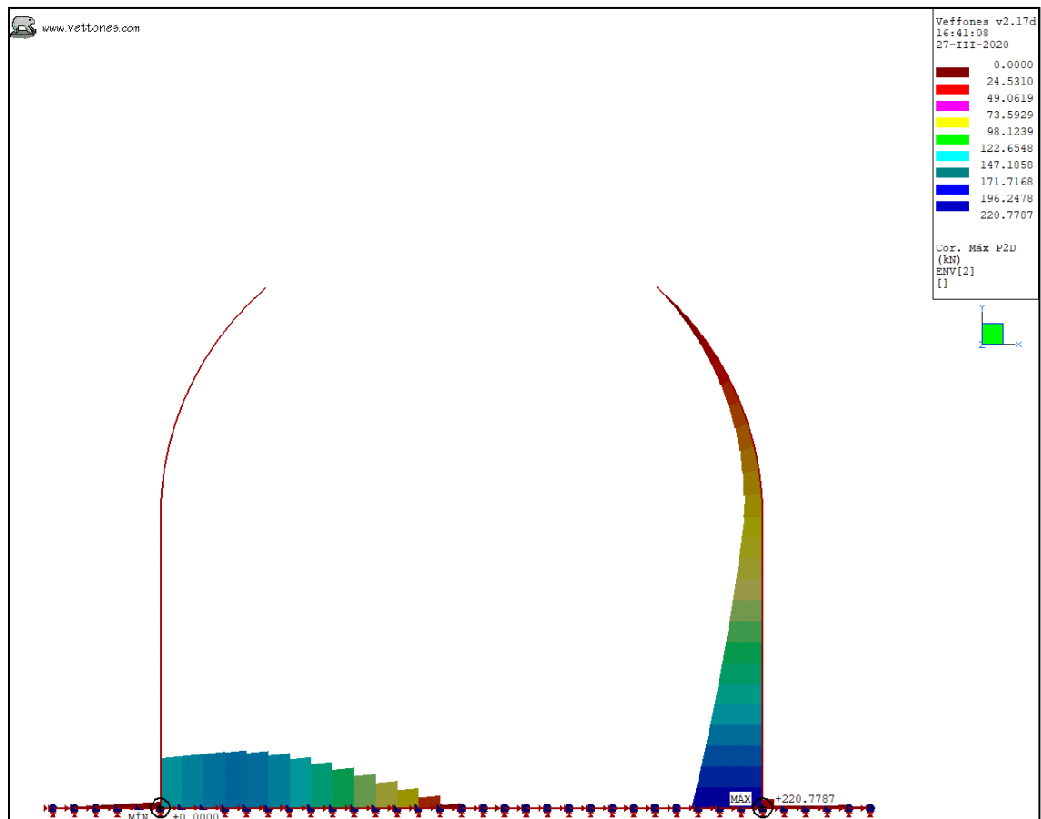
Ilustración 17. Envoltente ELU, K30 = 100 kgf/cm 3 . Sección Pico Flauta. Cortante máximo
