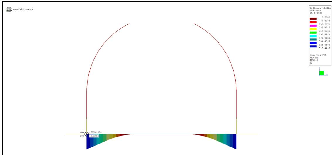
Ilustración 27. Momento Max (kN*m)
