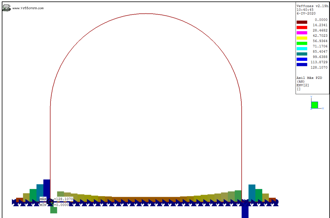
Ilustración 32. Envolvente ELU, k30 = 800 kgf/cm3. Normal máximo.
