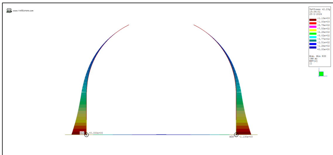
Ilustración 36. Momento Min (kN*m)
