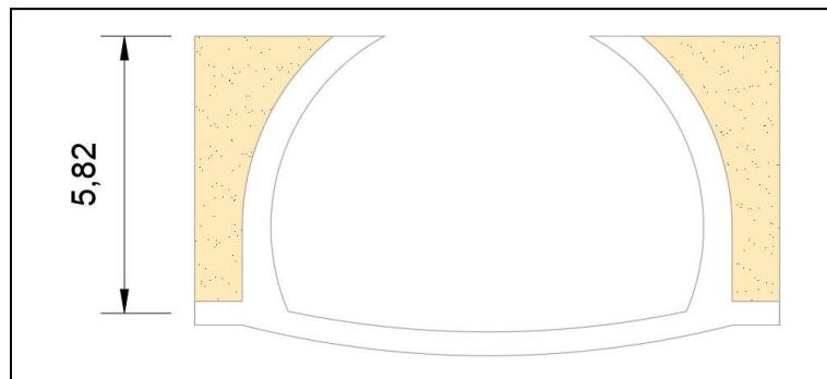
Ilustración 3. Esquema – Área del peso de tierras
