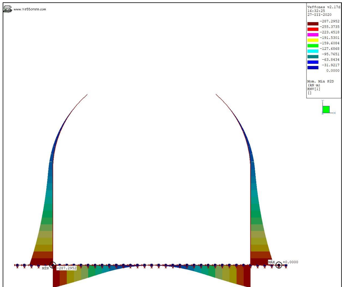
Ilustración 25. Envolvente ELS, K30 = 800 kgf/cm3. Sección Pico Flauta. Momento mínimo
