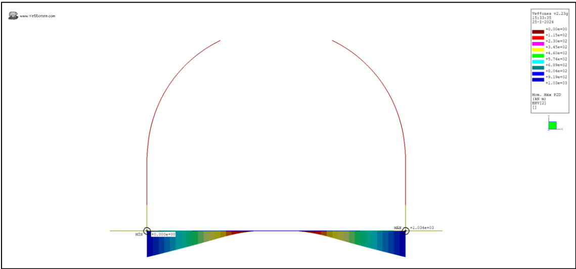
Ilustración 33. Momento Max (kN*m)
