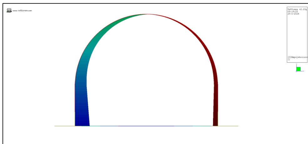
Ilustración 10. Acción – 3 Empuje de tierras K_0 y K_a/2
