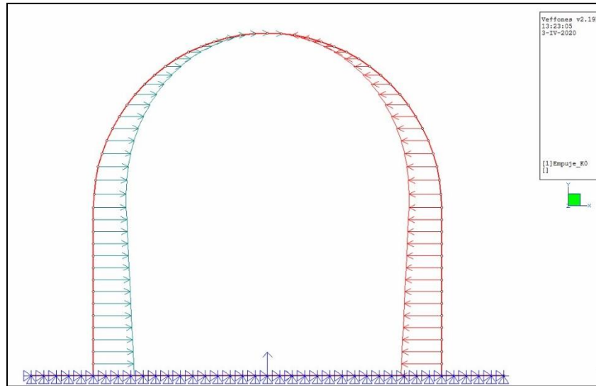
Ilustración 4. Empuje de tierras – Reposo
