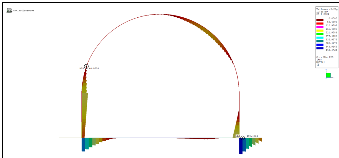
Ilustración 30. Cortante Max (kN)
