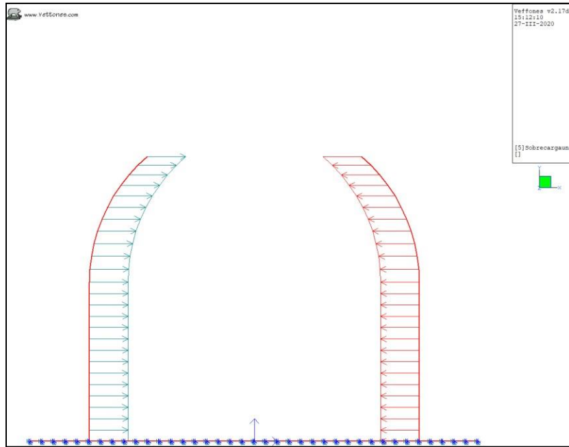
Ilustración 9 Sobrecarga uniforme en superficie (SCU). Efectos horizontales.
