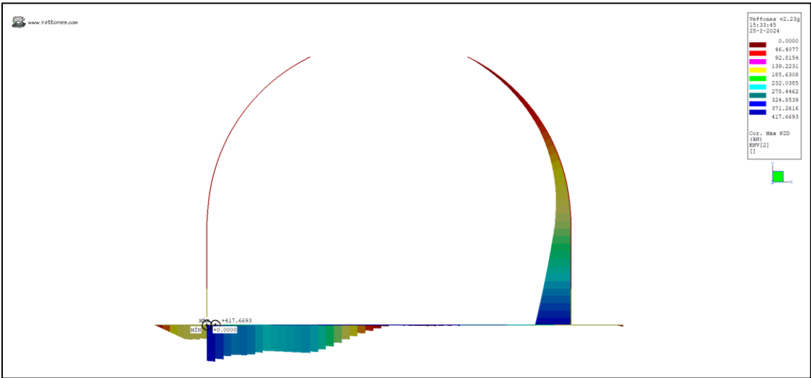
Ilustración 34. Cortante Max (kN)
