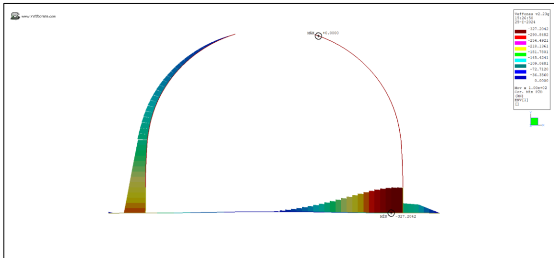
Ilustración 19. Cortante Min (kN)
