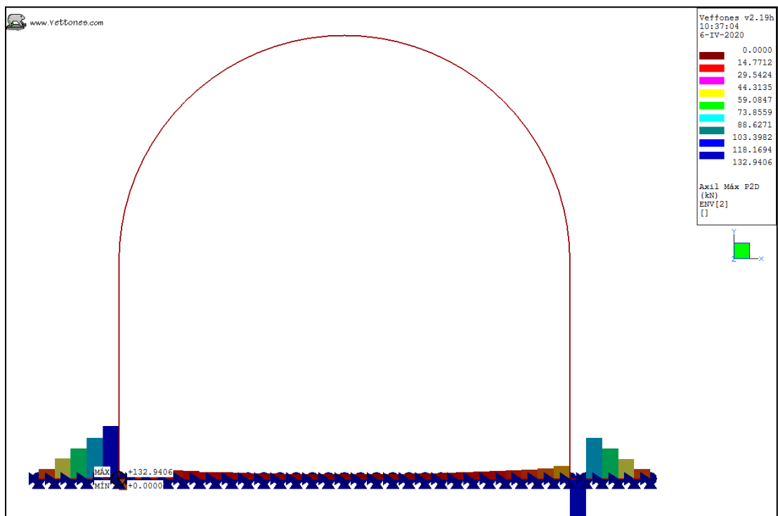
Ilustración 20. Envolvente ELU, K30 =100 kgf/cm 3 . Normal máximo.
