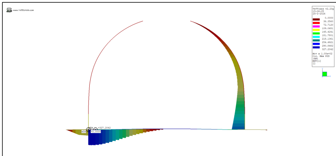
Ilustración 16. Cortante Max (kN)
