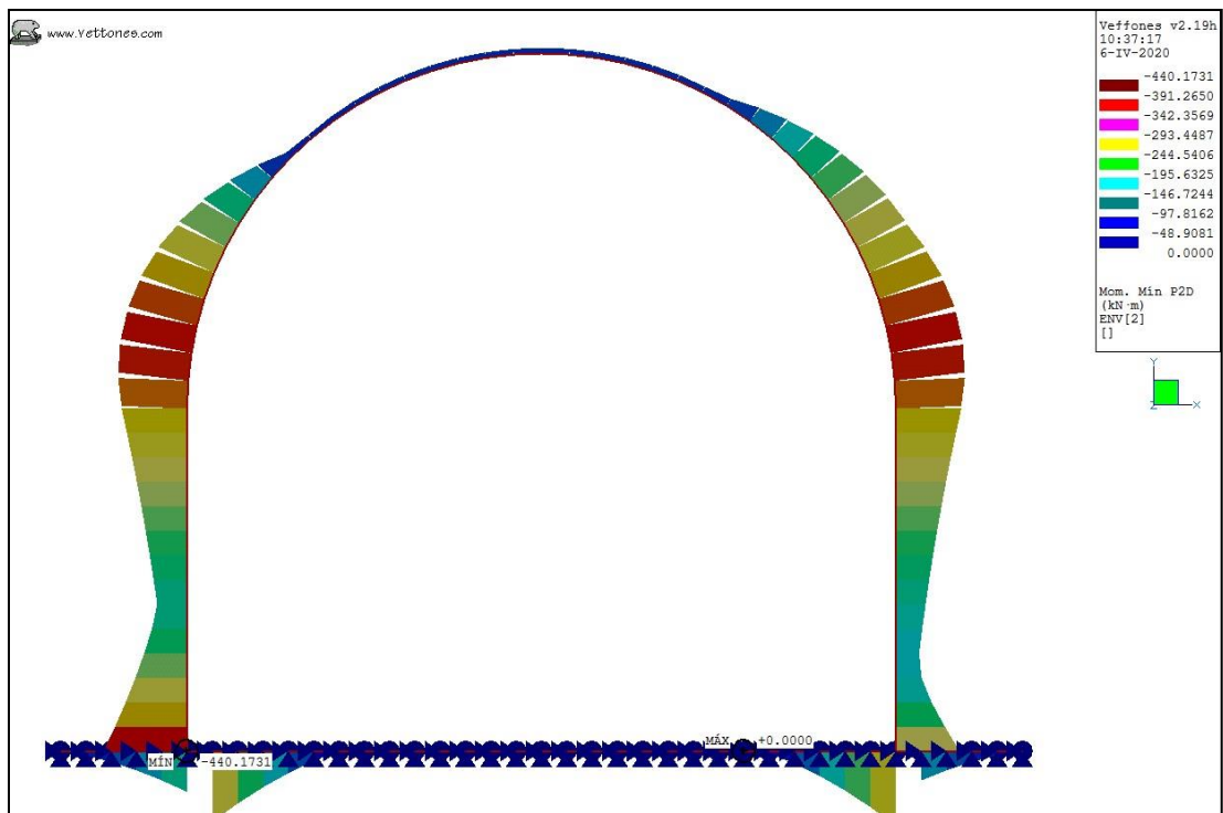
Ilustración 21. Envolvente ELU, K30 = 100 kgf/cm3. Momento mínimo.
