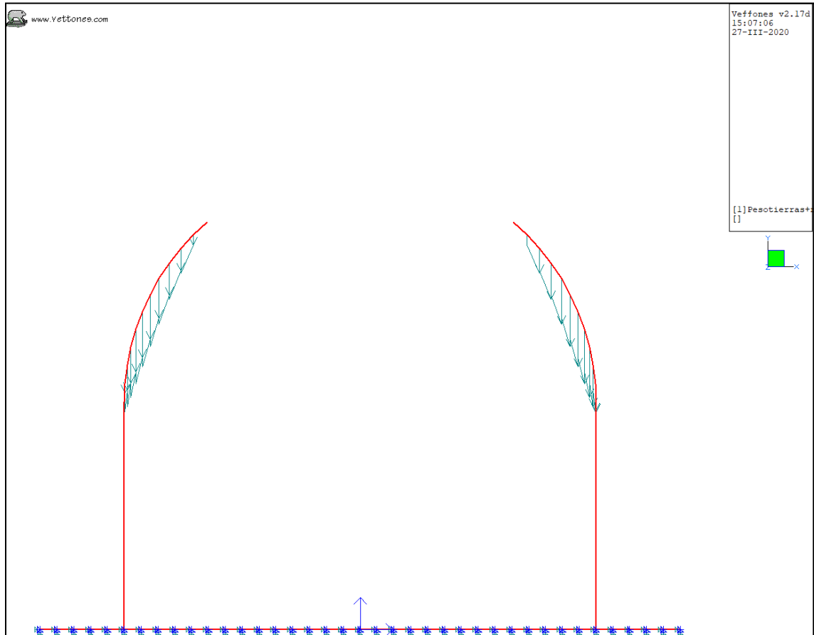
Ilustración 6 Carga vertical de tierras
