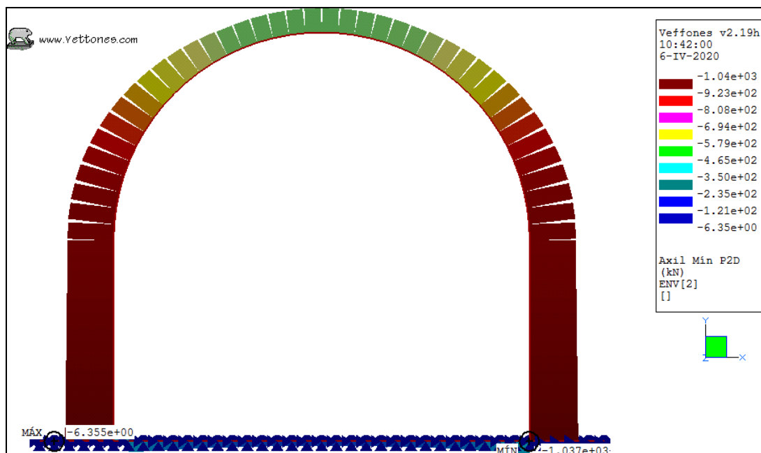
Ilustración 35. Envolvente ELU, K30 = 800 kgf/cm 3 . Normal mínimo.
