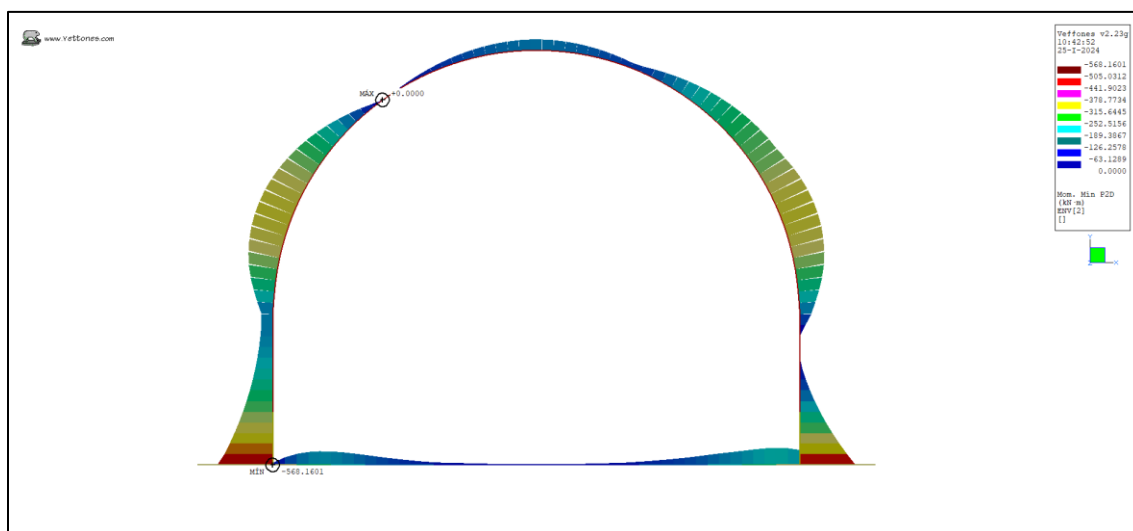
Ilustración 38. Momento Min (kN*m)
