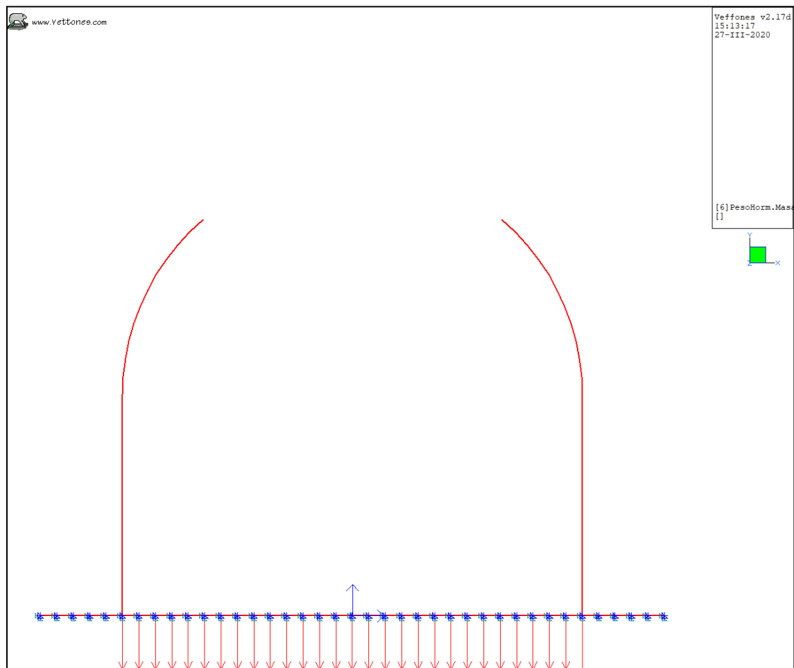
Ilustración 7. Peso de la losa de hormigón en masa
