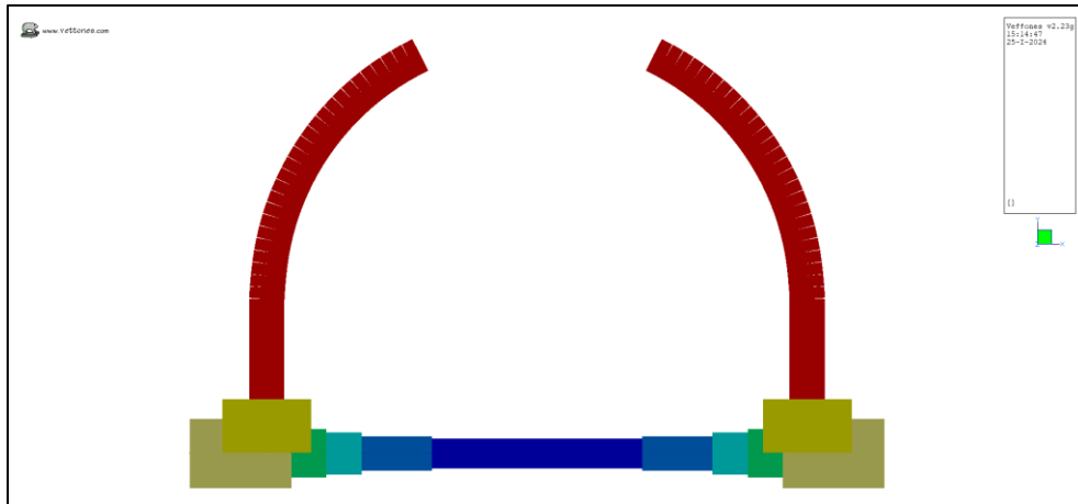
Ilustración 5. Acción – 0 Peso propio
