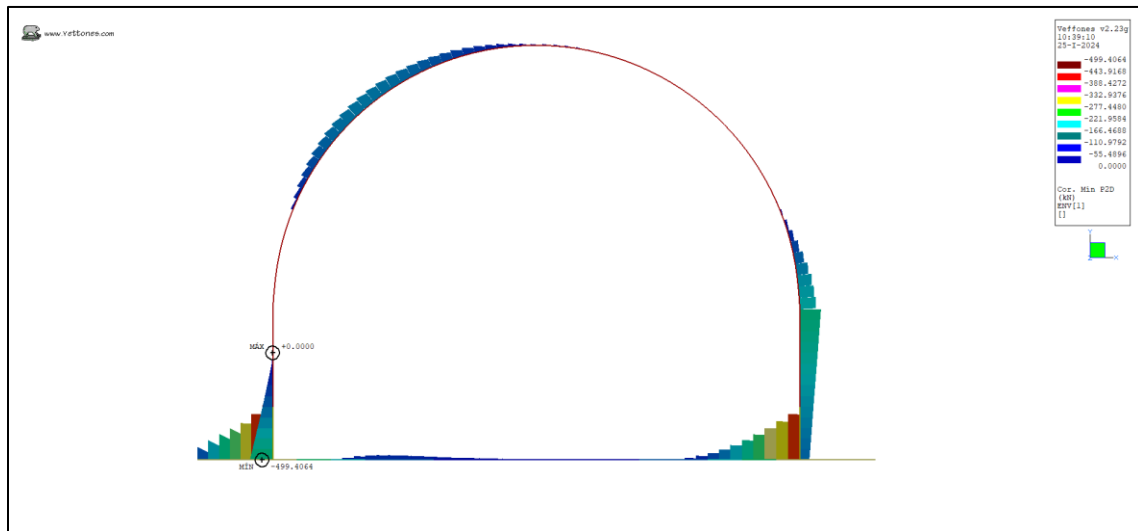
Ilustración 33. Cortante Min (kN)
