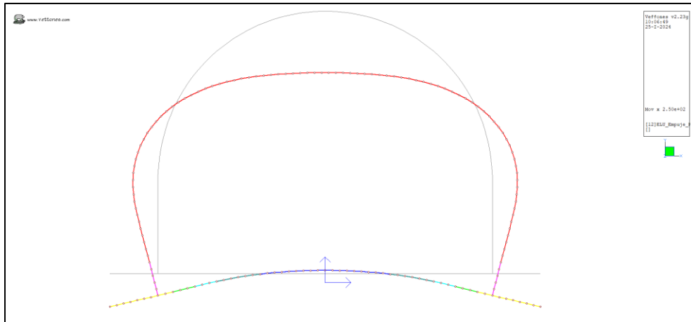
Ilustración 16. Segunda condición de análisis.
