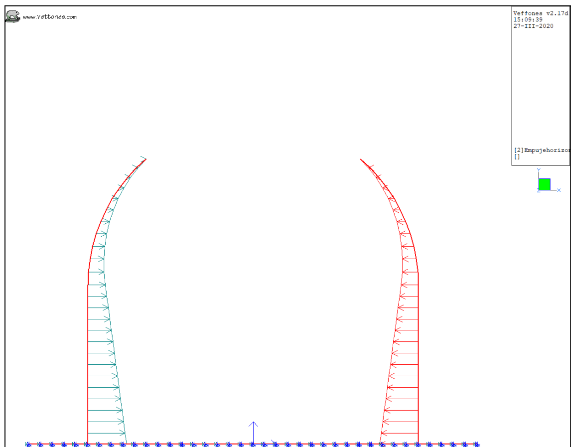
Ilustración 4. Empuje de tierras – Reposo
