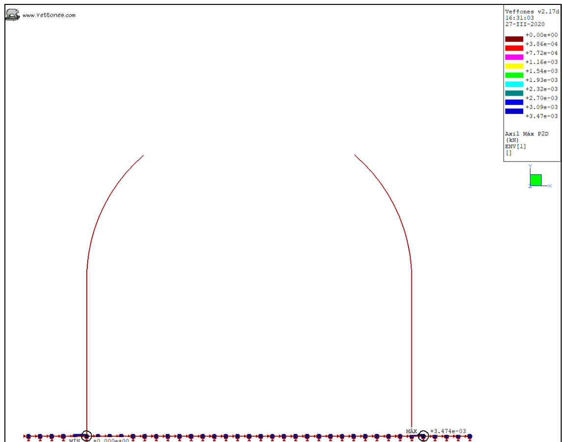
Ilustración 24 Envolvente ELS, K30 = 800 kgf/cm 3 . Sección Pico Flauta. Normal máximo
