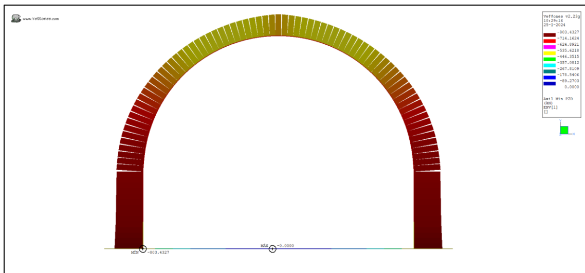
Ilustración 22. Axil Min (kN)
