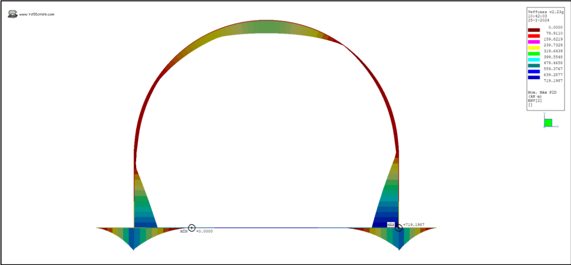
Ilustración 35. Momento Max (kN*m)
