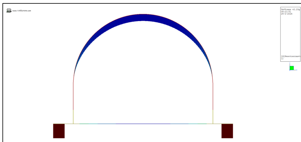
Ilustración 11. Acción – 4 Peso de tierras más rozamiento negativo
