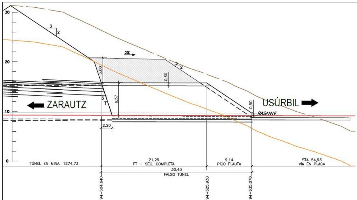
Ilustración 1 Falso túnel de galería. Perfil longitudinal
