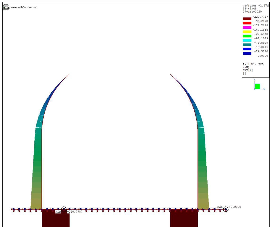
Ilustración 21. Envoltorio ELU, K30 = 100 kgf/cm3. Sección pico Flauta. Normal mínimo
