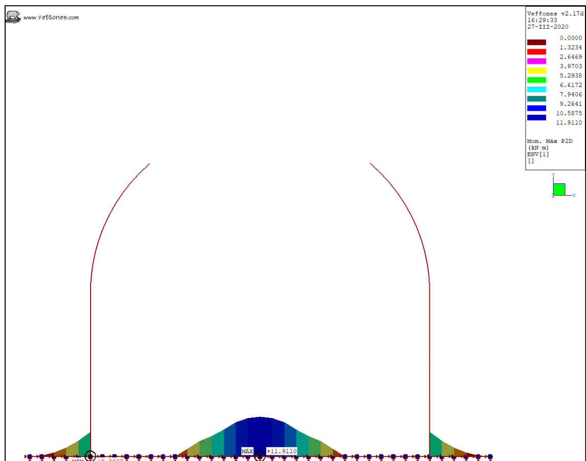
Ilustración 22. Envolvente ELS, K30 = 800 kgf/cm 3 . Sección Pico de Flauta. Momento máximo
