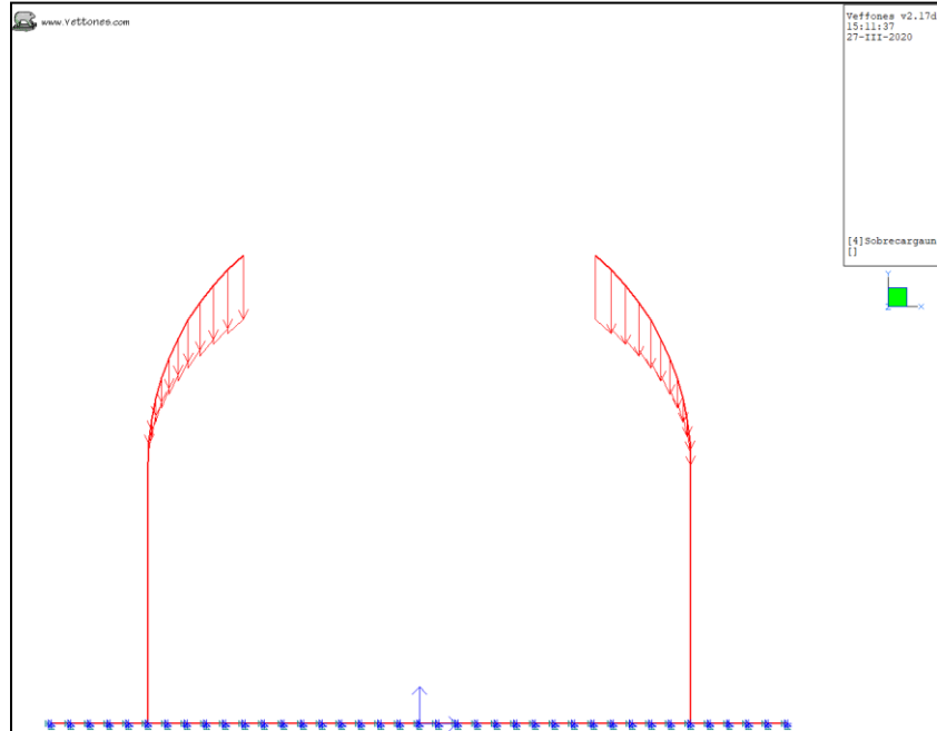
Ilustración 8. Sobrecarga uniforme en superficie (SCU). Efectos verticales.
