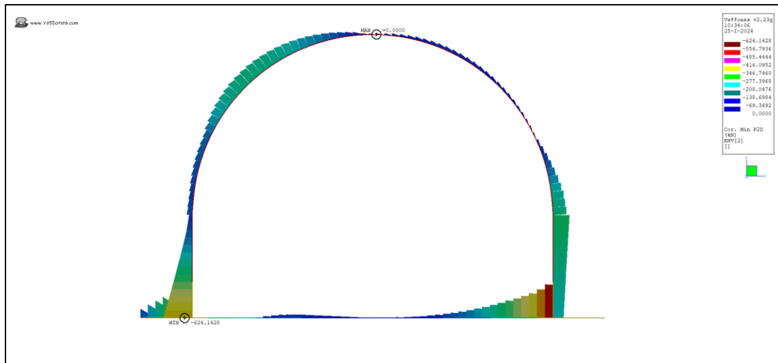
Ilustración 27. Cortante Min (kN)
