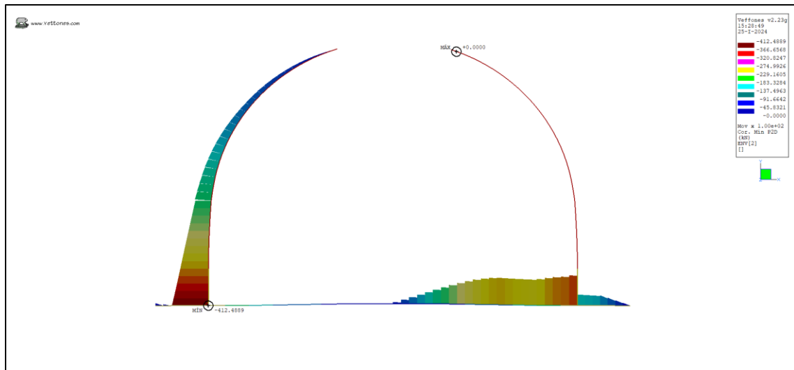
Ilustración 25. Cortante Min (kN)
