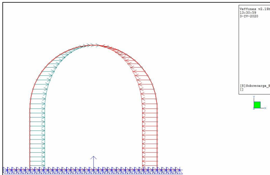
Ilustración 9 Sobrecarga uniforme en superficie (SCU). Efectos horizontales.
