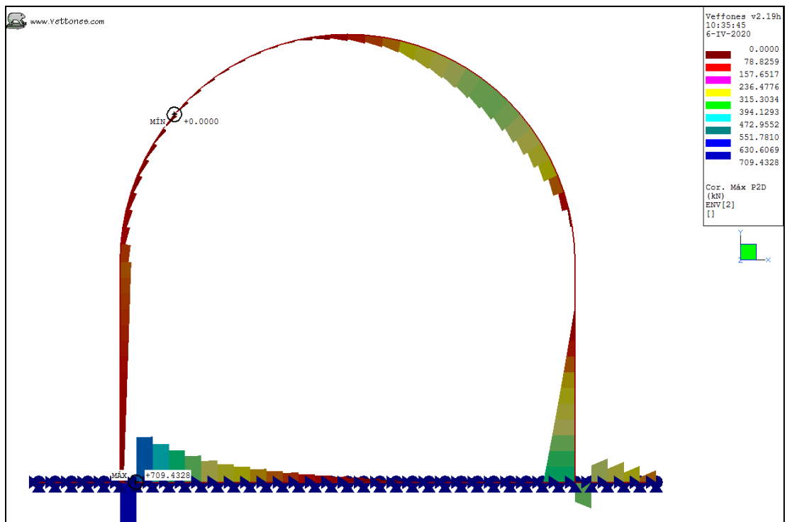
Ilustración 19. Envolvente ELU, K30 = 100 kgf/cm 3 . Cortante máximo.
