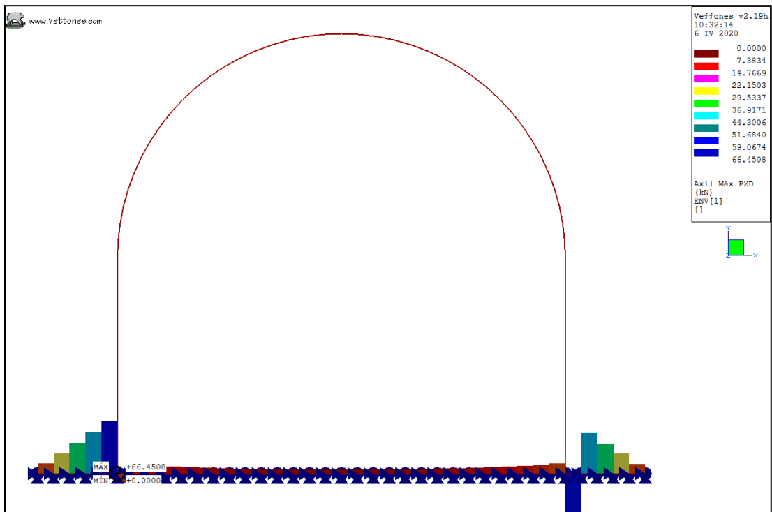
Ilustración 26 Envolverte ELS, K30 = 800 kgf/cm 3 . Normal máximo
