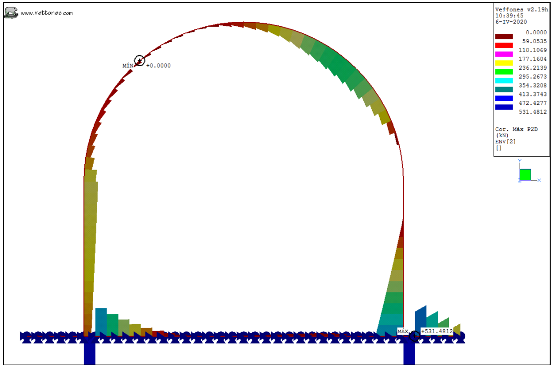
Ilustración 31. Envolvente ELU, K30 = 800 kgf/cm3. Cortante máximo
