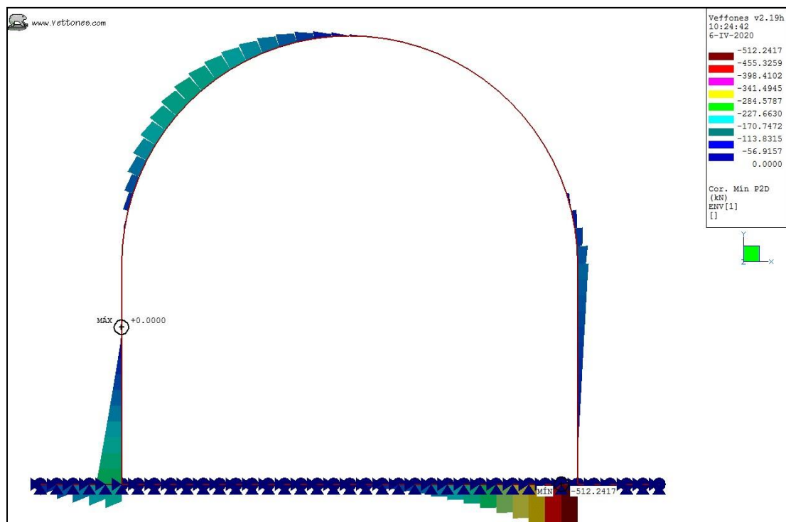
Ilustración 16. Envolvente ELS, K30 = 100 kgf/cm 3 . Cortante mínimo.
