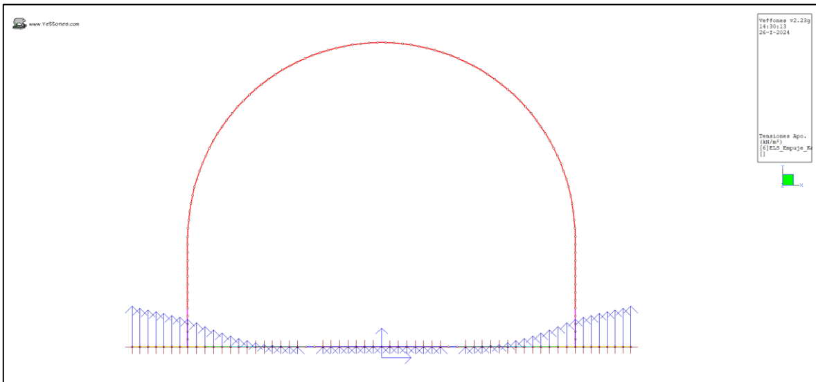
Ilustración 41. Reacción del suelo de cimentación.
