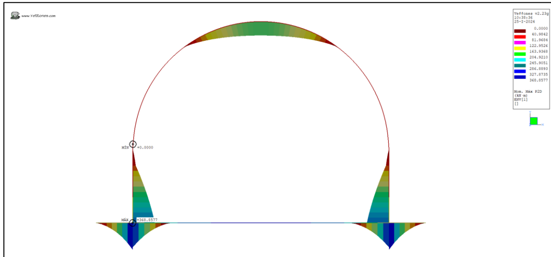
Ilustración 29. Momento Max (kN*m)
