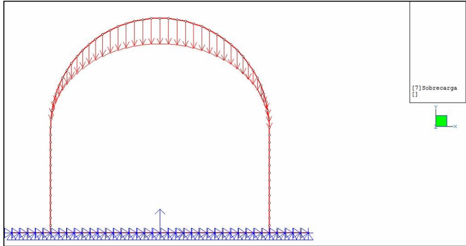
Ilustración 8. Sobrecarga uniforme en superficie (SCU). Efectos verticales.
