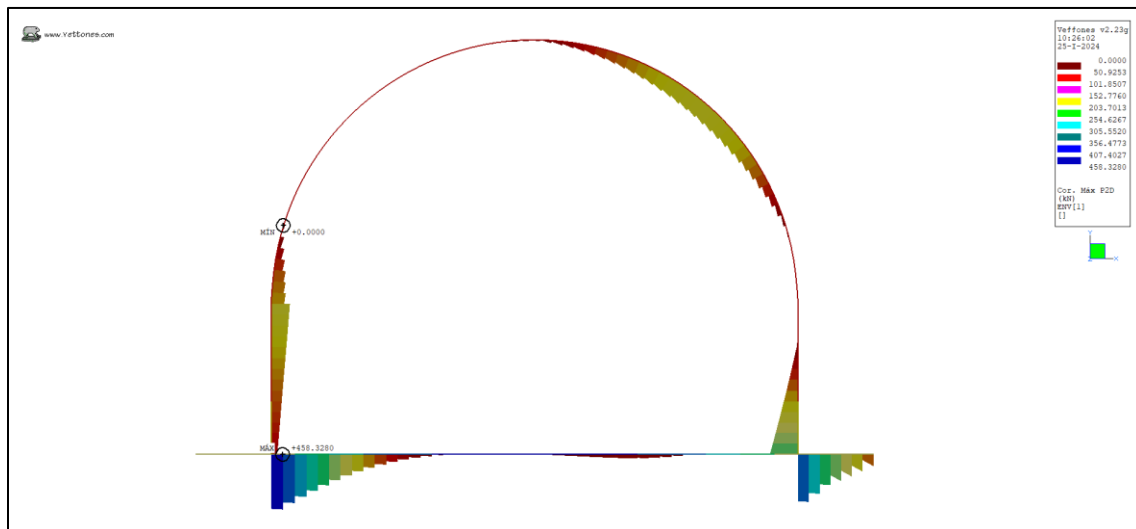
Ilustración 18. Cortante Max (kN)
