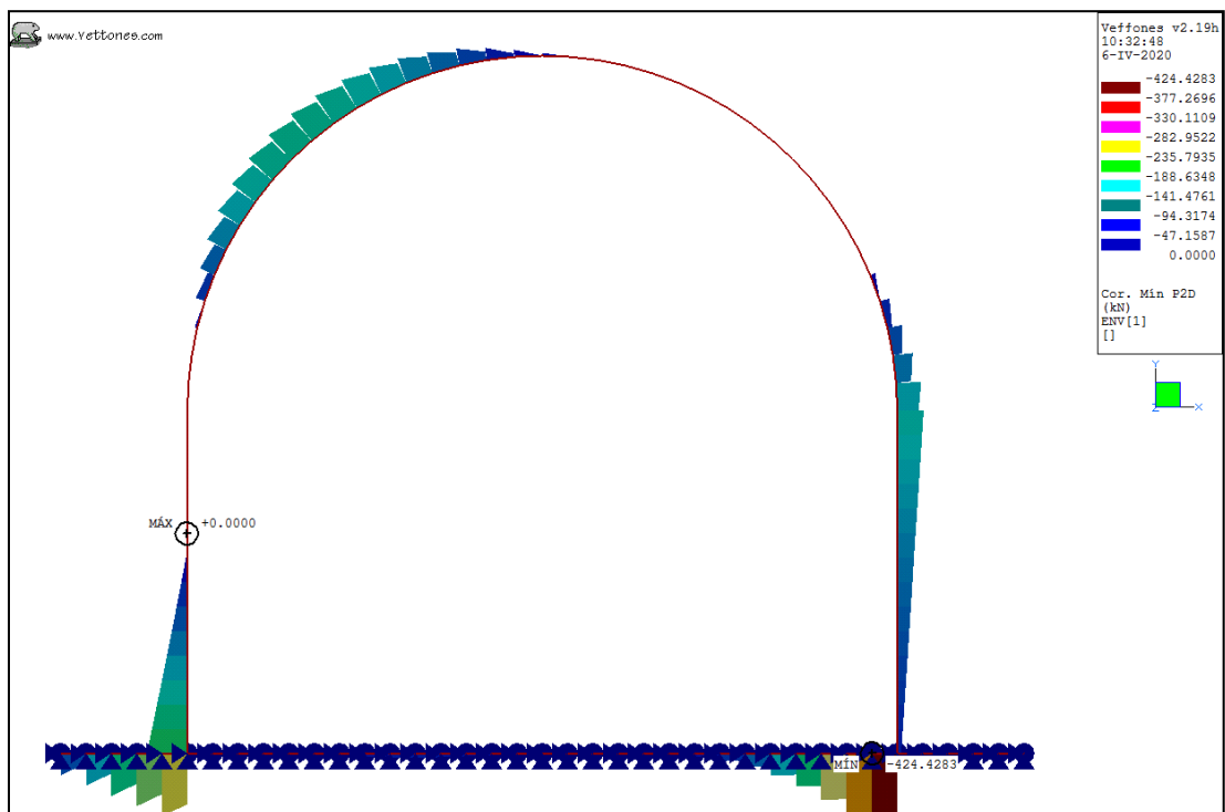
Ilustración 28. Envolvente ELS, K30 = 800 kgf/cm3. Cortante mínimo.
