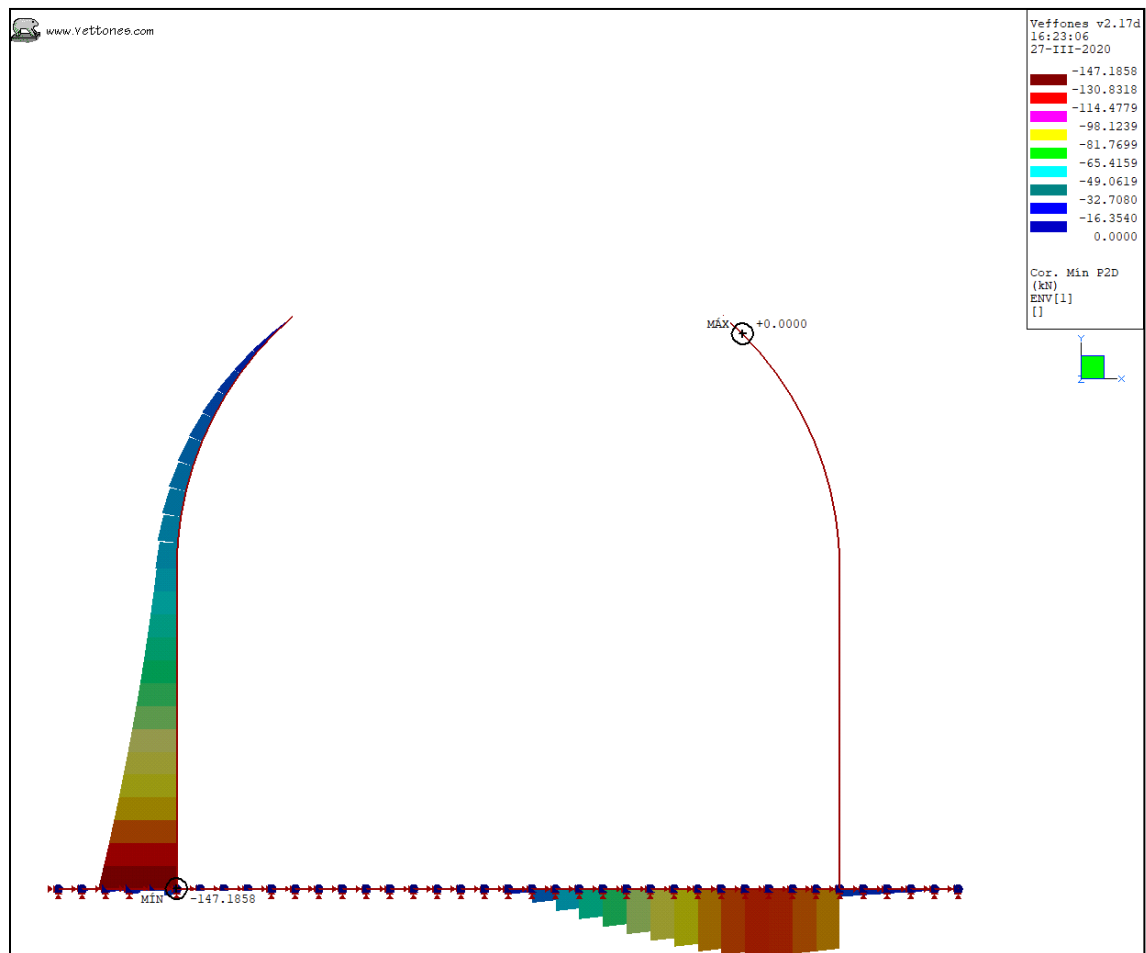
Ilustración 14. Envolvente ELS, K30 = 100 kgf/cm 3 . Sección Pico Flauta. Cortante mínimo.
