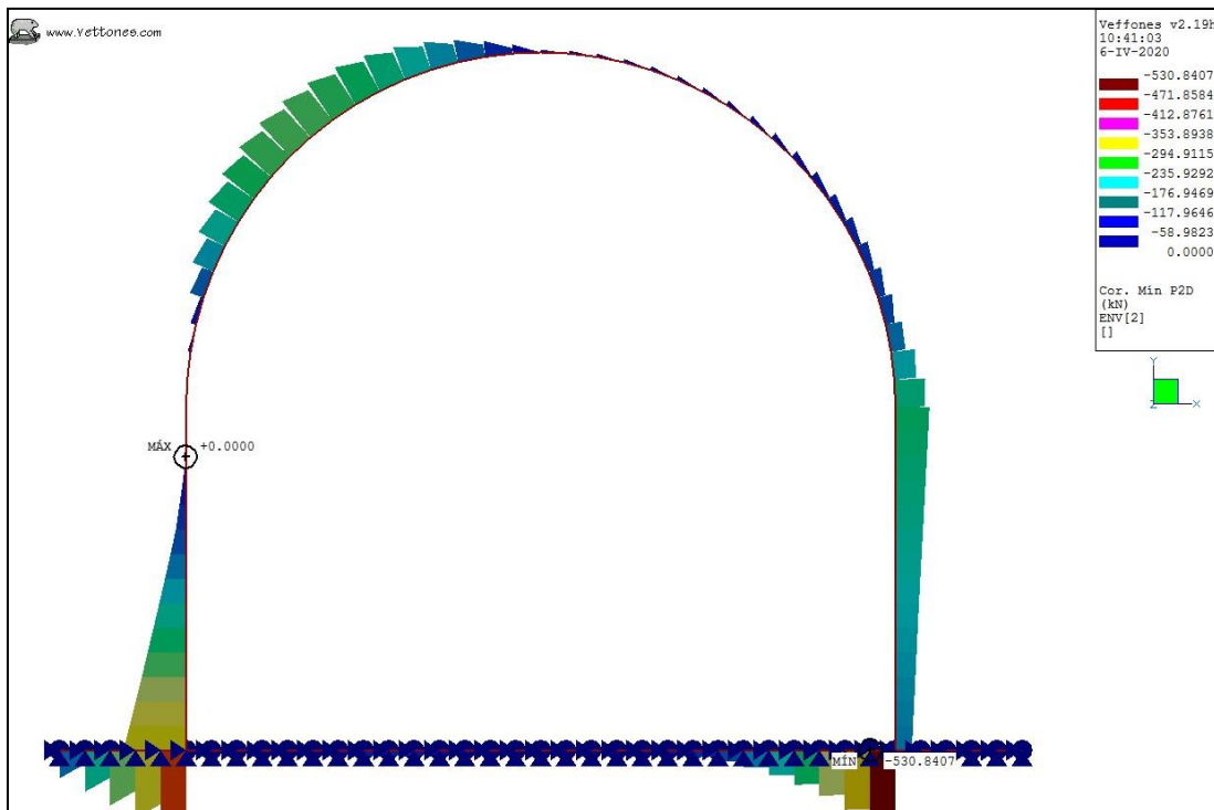
Ilustración 34. Envolvente ELU, K30 = 800 kgf/cm3. Cortante mínimo.
