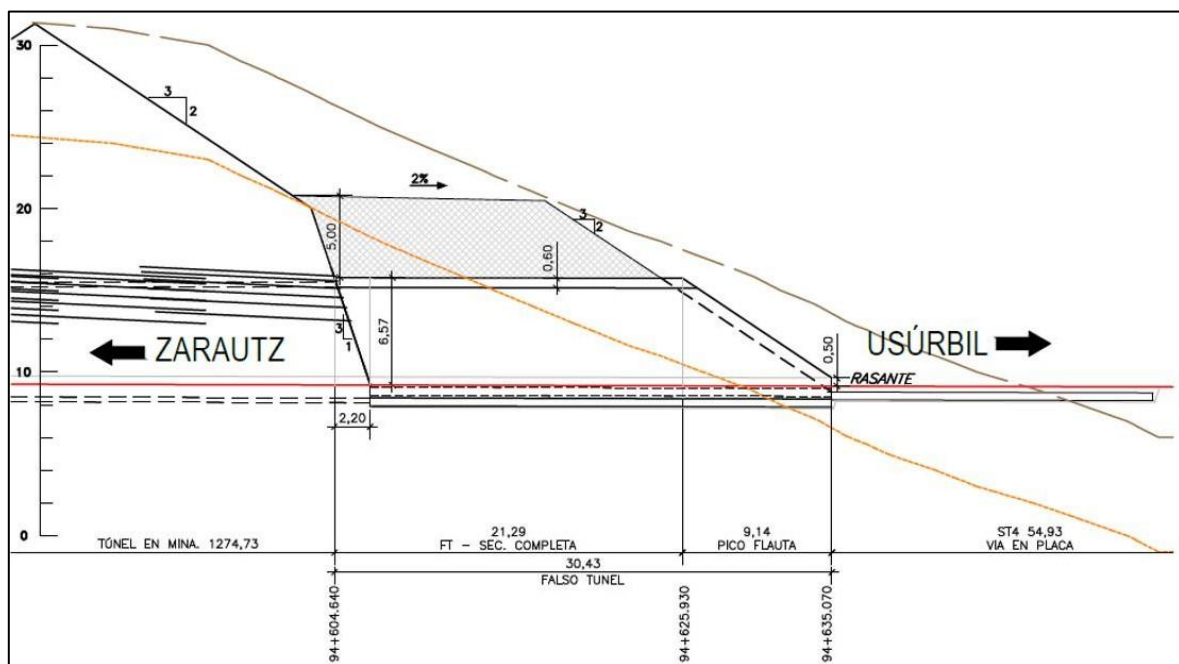
Ilustración 1 Pico de flauta
