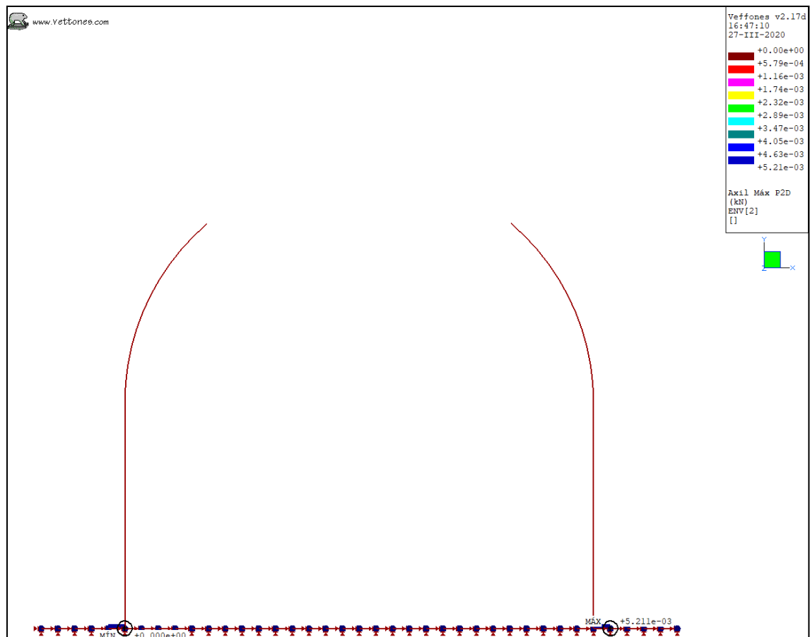
Ilustración 30. Envolvente ELU, k_{30} = 800 \text{ kgf/cm}^3 . Sección Pico Flauta. Normal máximo.
