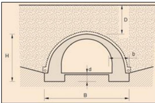
Ilustración 3. Geometría tipo de la sección
