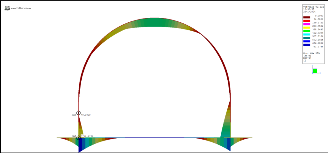
Ilustración 23. Momento Max (kN*m)
