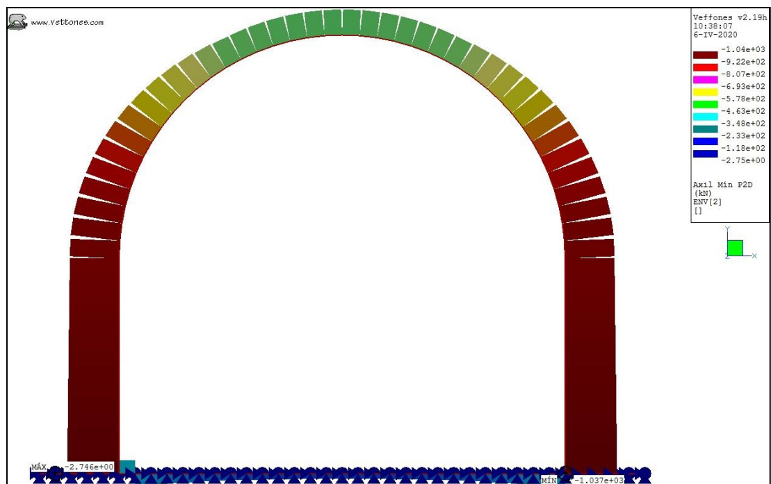
Ilustración 23. Envoltente ELU, K30 = 100 kgf/cm3. Sección completa de galería. Normal mínimo
