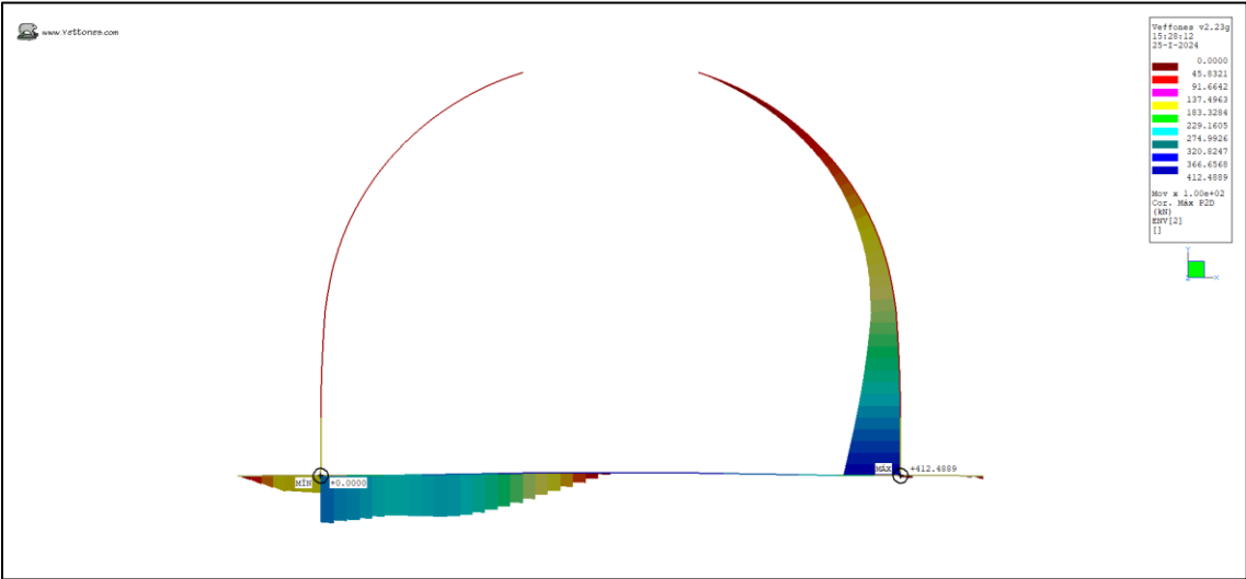
Ilustración 22. Cortante Max (kN)
