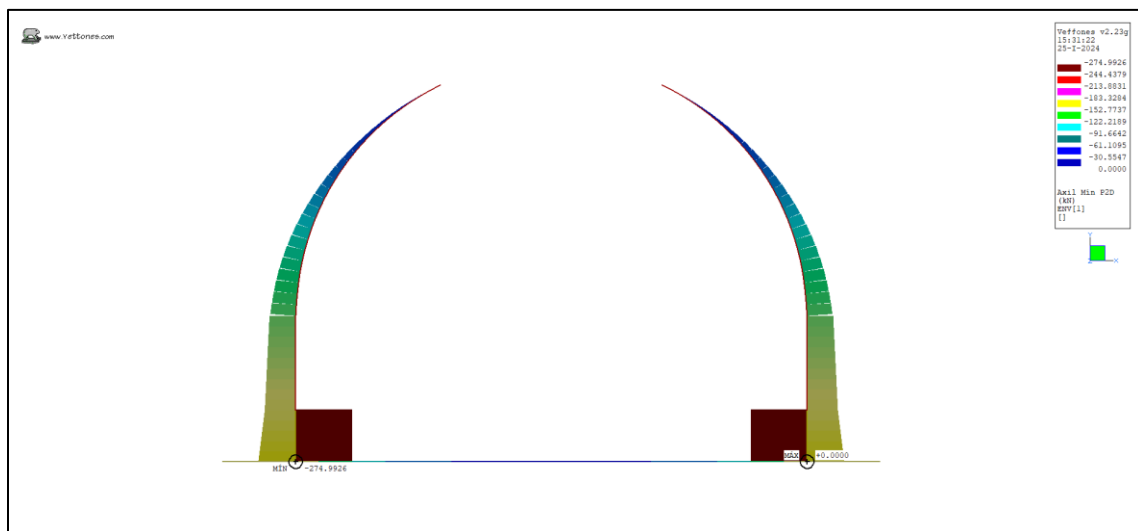
Ilustración 32. Axil Min (kN)
