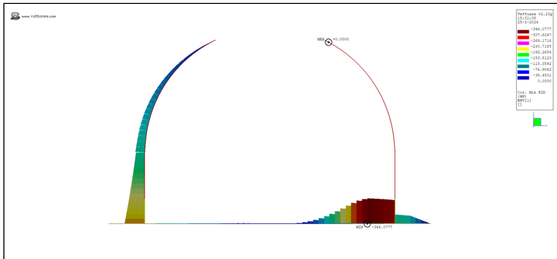
Ilustración 31. Cortante Min (kN)
