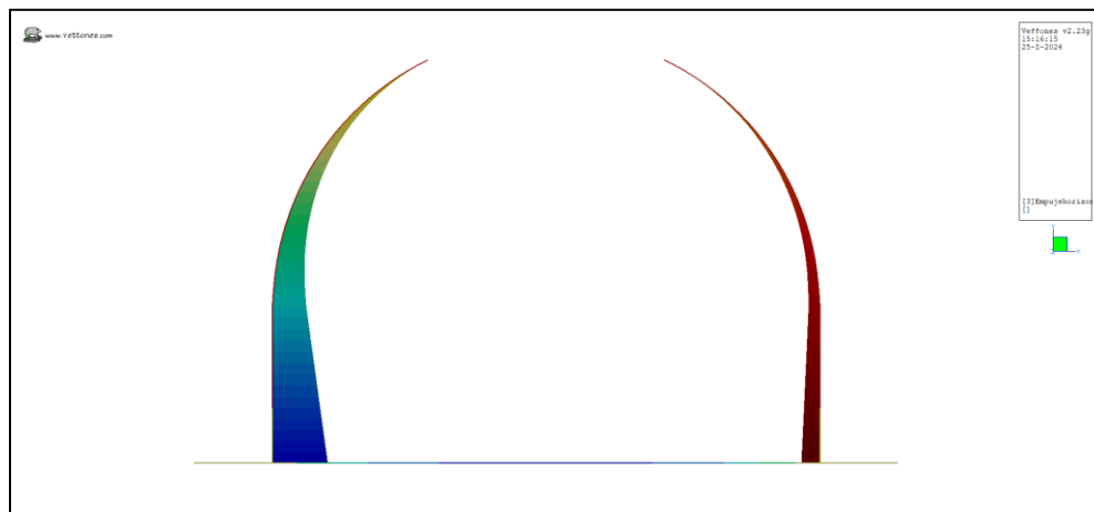
Ilustración 8. Acción – 3 Empuje de tierras Ko y Ka/2
