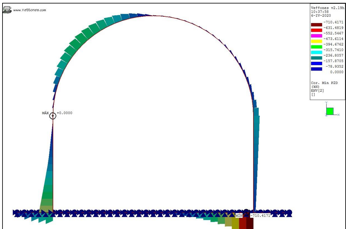
Ilustración 22. Envolvente ELU, K30 = 100 kgf/cm3. Cortante mínimo.
