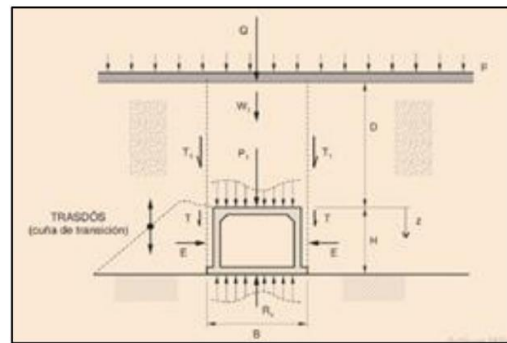
Ilustración 4. Fuerzas del sistema
