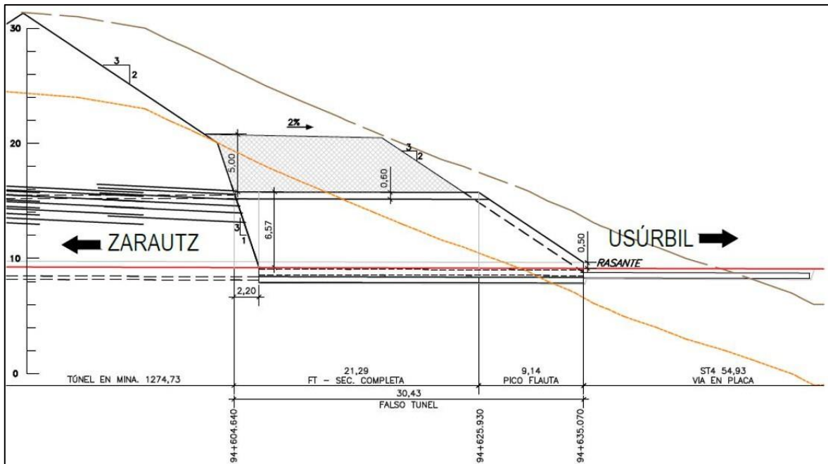
Ilustración 1 Falso túnel de galería. Perfil longitudinal
