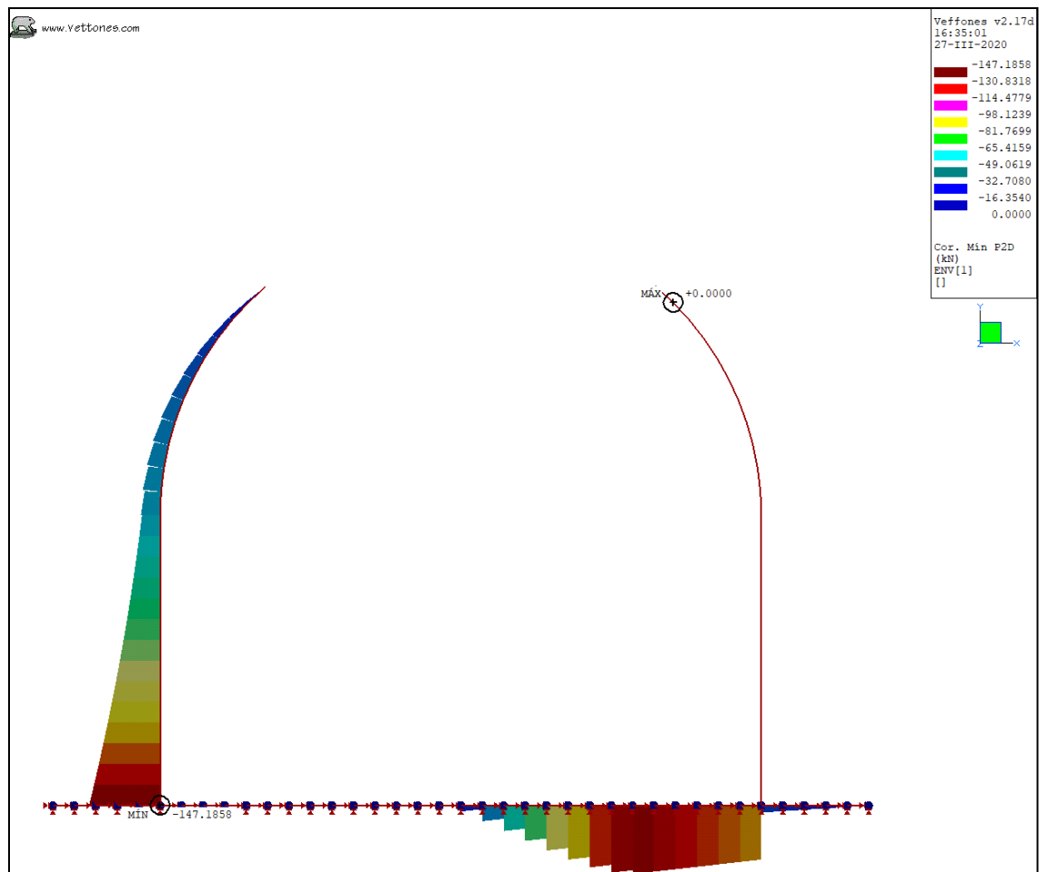
Ilustración 26. Envolverte ELS, K30 = 800 kgf/cm3. Sección Pico Flauta. Cortante mínimo.
