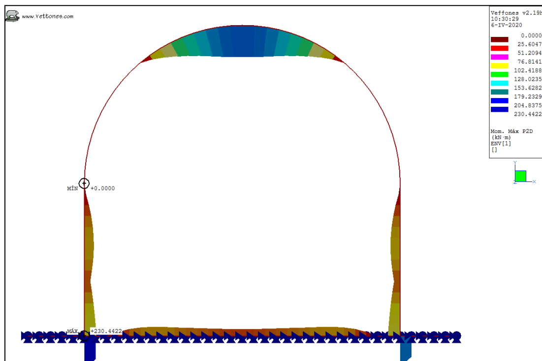
Ilustración 24. Envolvente ELS, K30 = 800 kgf/cm 3 . Momento máximo
