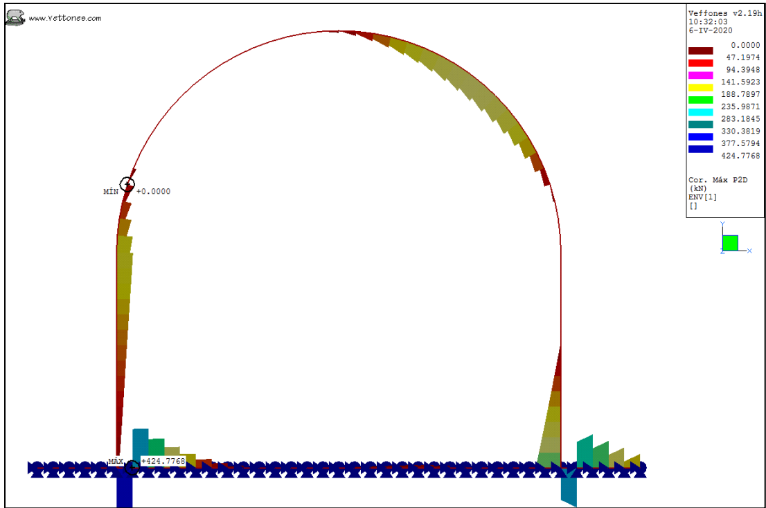
Ilustración 25. Envolverte ELS, K30 = 800 kgf/cm 3 . Cortante máximo
