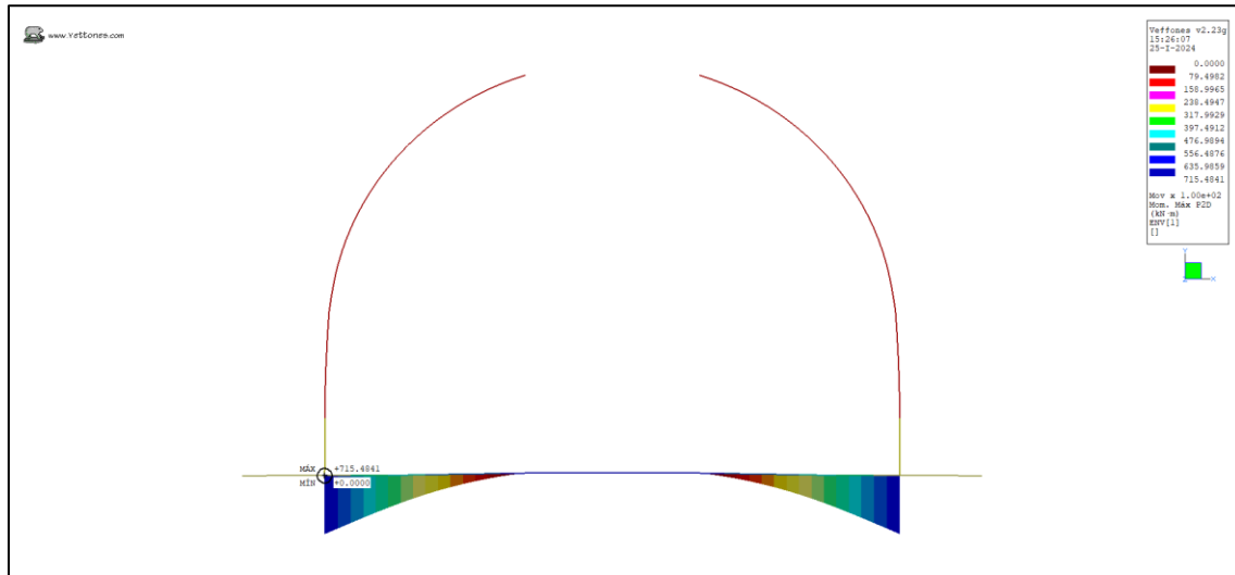
Ilustración 15. Momento Max (kN*m)
