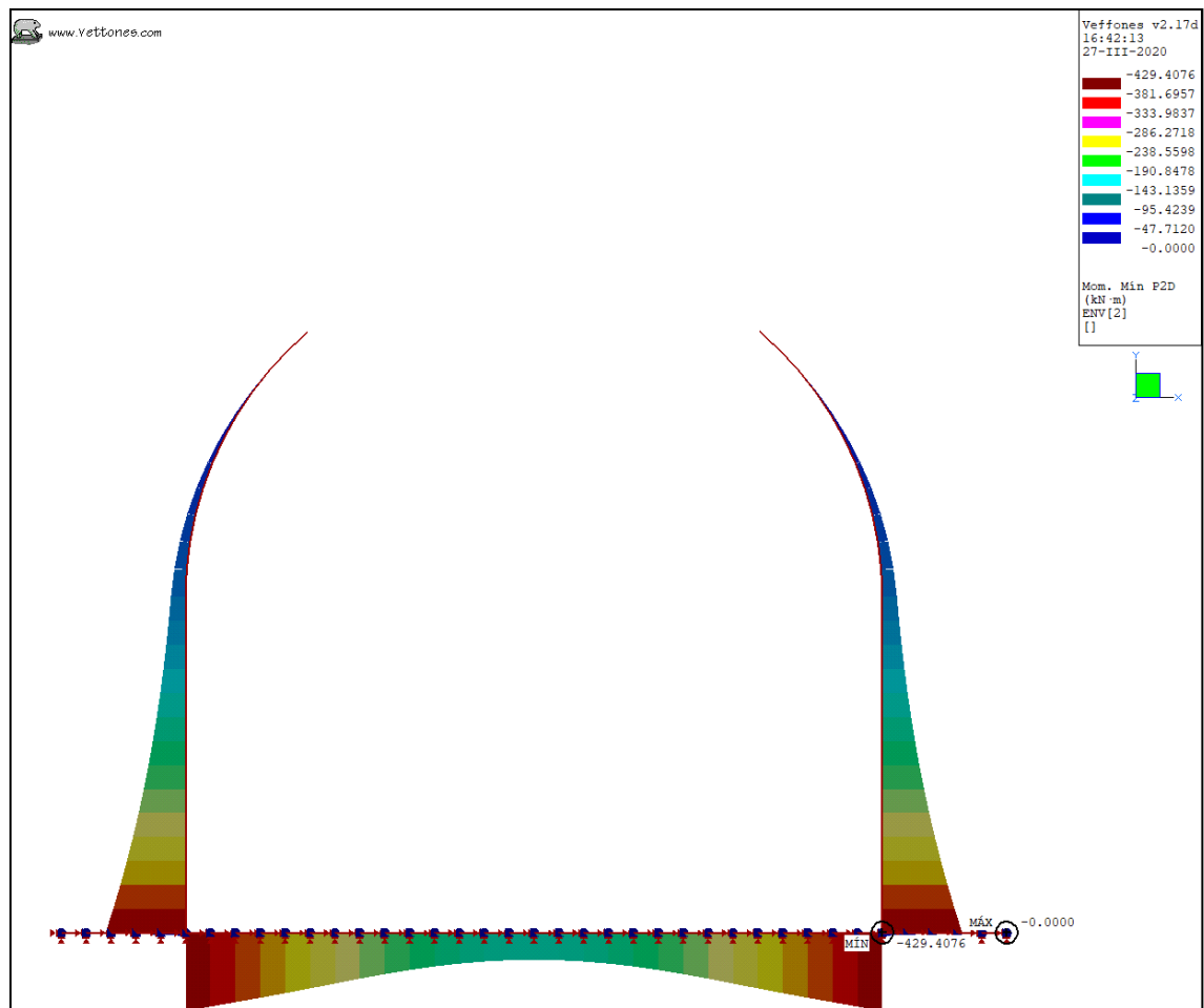
Ilustración 19. Envolvente ELU, K30 = 100 kgf/cm 3 . Sección Pico Flauta. Momento mínimo.
