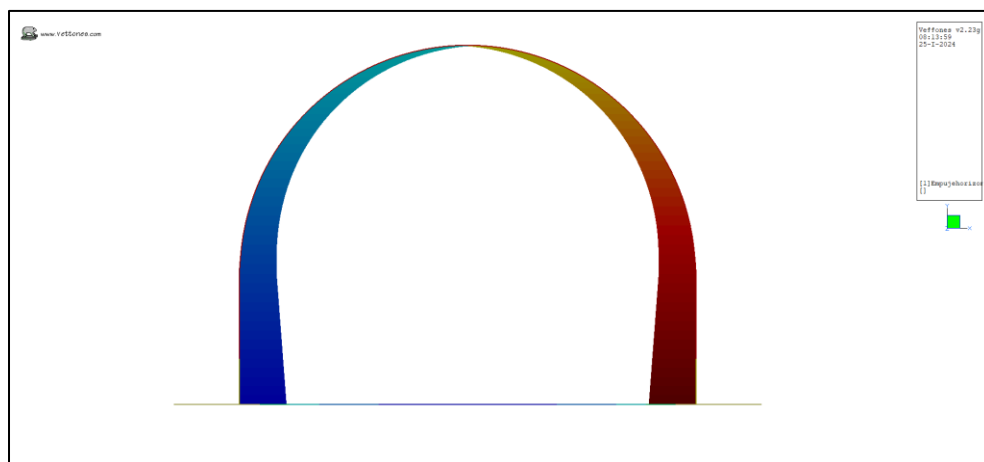
Ilustración 8. Acción – 1 Empuje de tierras K_o
