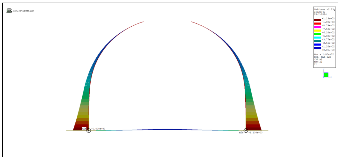
Ilustración 24. Momento Min (kN*m)
