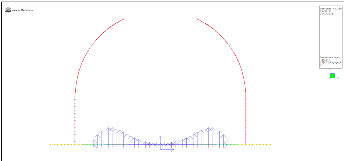
Ilustración 39. Reacción del suelo de cimentación.
