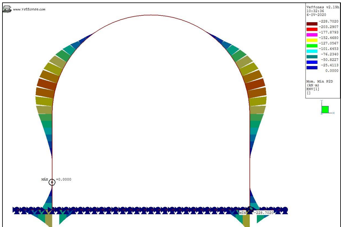
Ilustración 27. Envolvente ELS, K30 = 800 kgf/cm3. Momento mínimo
