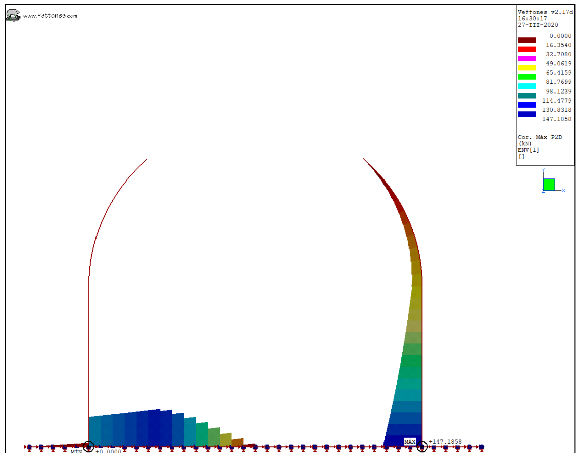
Ilustración 23. Envoltente ELS, K30 = 800 kgf/cm3. Cortante máximo
