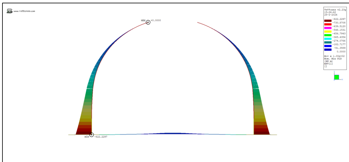
Ilustración 18. Momento Min (kN*m)
