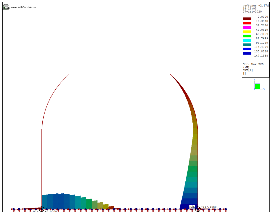
Ilustración 11. Envoltente ELS, K30 = 100 \text{ kgf/cm}^3 . Sección Pico Flauta. Cortante máximo.
