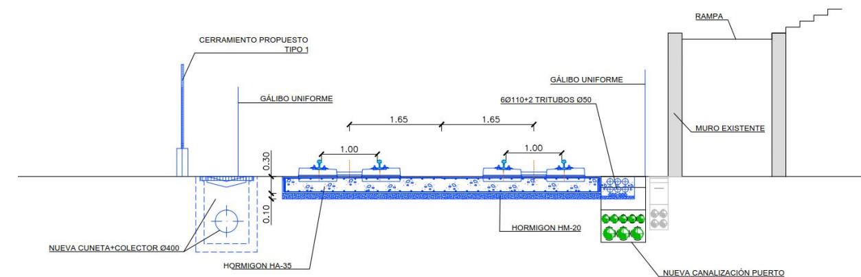
FIGURA 2. SISTEMA DE DRENAJE CUNETA+COLECTOR EN MARGEN IZQUIERDA
