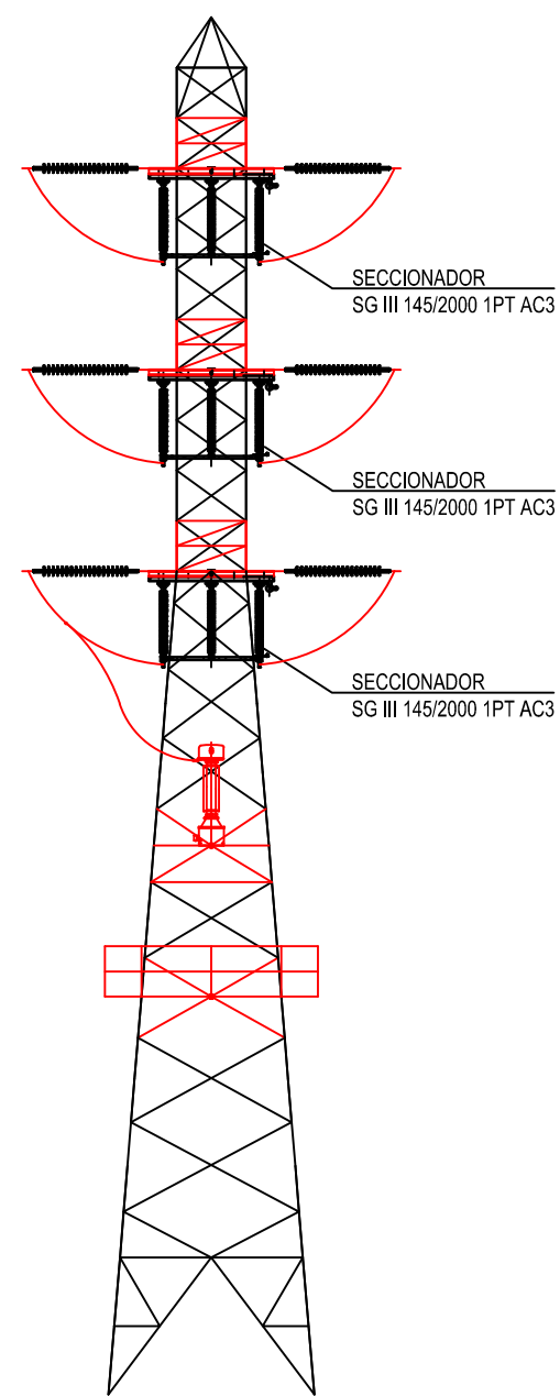
VISTA LATERAL
