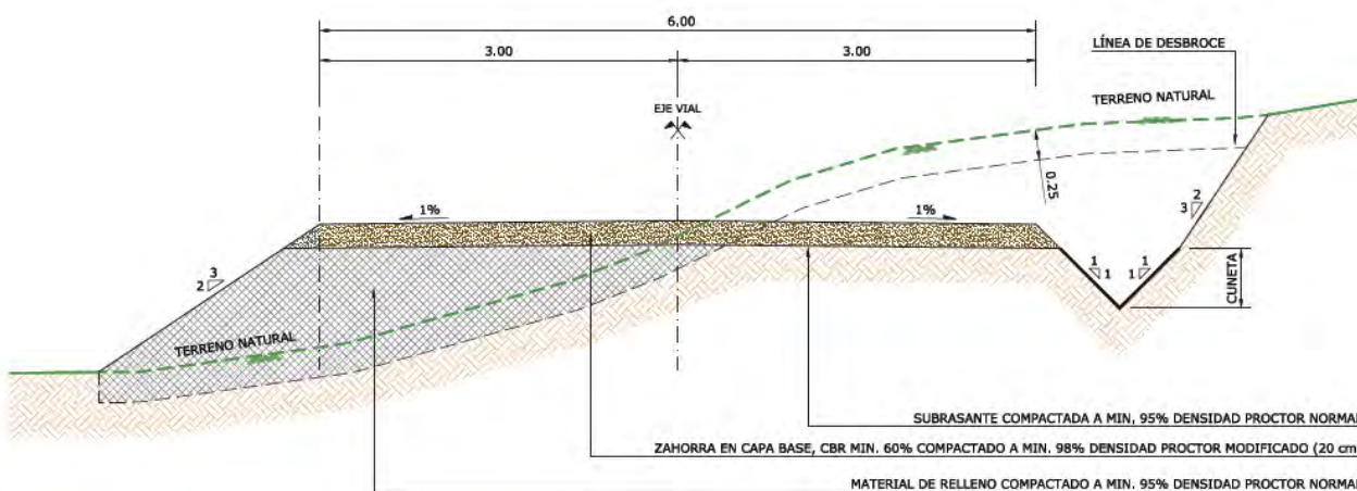
Figura 1. Sección tipo vial de material granular
