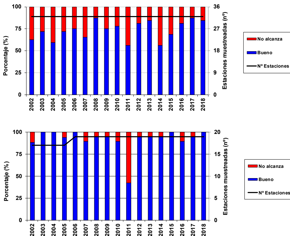
Figura 14 Evolución del estado químico en los estuarios (arriba) y litoral-plataforma (abajo) de la Comunidad Autónoma del País Vasco (Azul: Bueno y Rojo: No alcanza), junto con el número de estaciones muestreadas anualmente (línea negra).
