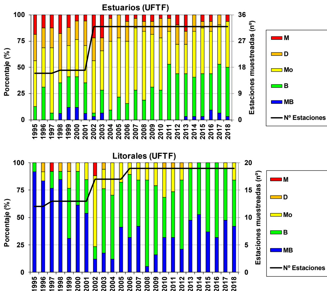
Figura 13 Evolución del estado ecológico, calculado con el principio ‘ uno fuera, todos fuera ’ (UFTF) en los estuarios (arriba) y litoral-plataforma (abajo) de la Comunidad Autónoma del País Vasco (Azul: Muy Bueno; Verde: Bueno; Amarillo: Moderado; Naranja: Deficiente y Rojo: Malo), junto con el número de estaciones muestreadas anualmente (línea negra).
