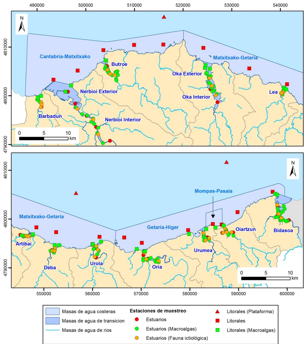
Figura 2 Mapa que muestra la ubicación de las estaciones de control de la Red de seguimiento del estado ecológico de las aguas de transición y costeras de la CAPV.
