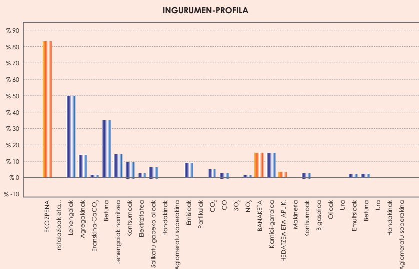
Asfaltoaren ingurumen-alderdiak
