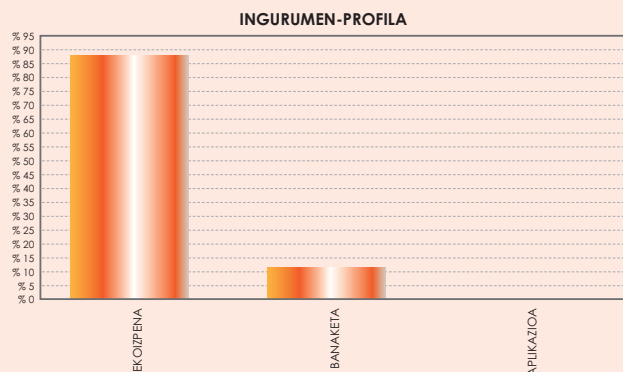
Enkofratu-olioaren ingurumen-profila
