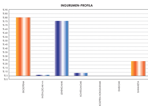
Hormigoiaren ingurumen-profila
