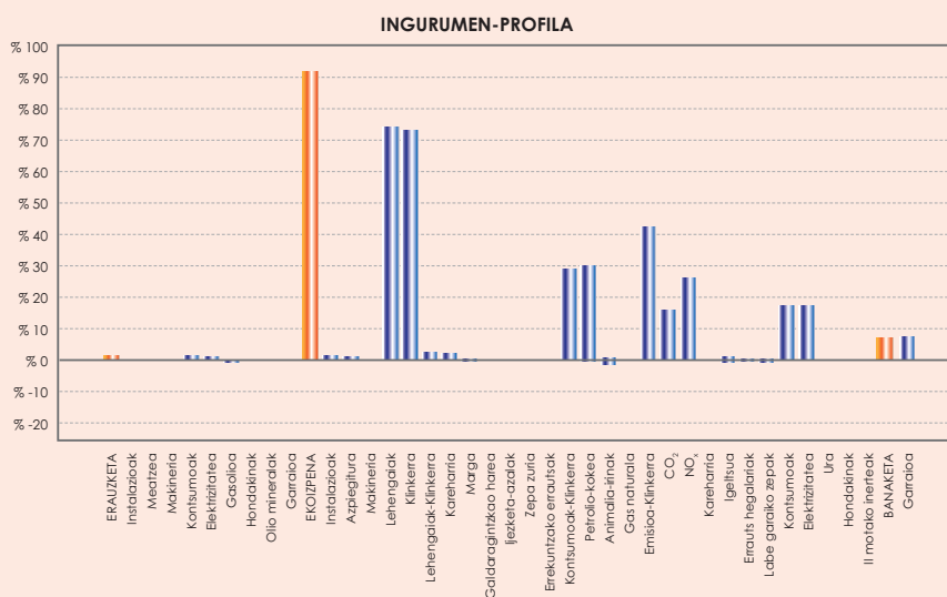
Zementuaren ingurumen-alderdiak
