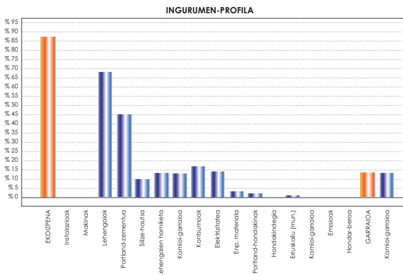
Zementuaren ingurumen-alderdiak
