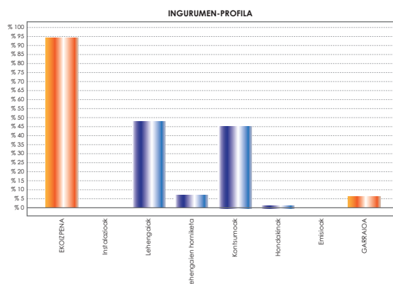
Asfaltoaren ingurumen-profila
