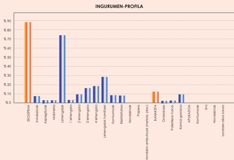
Enkofratu-olioaren ingurumen-alderdiak
