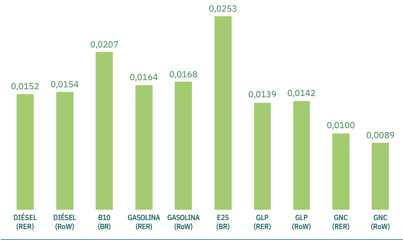
Gráfica 163 – Comparativa de impacto en puntuación única ReCiPe para producir 1kWh de energía para combustión (Pt)
