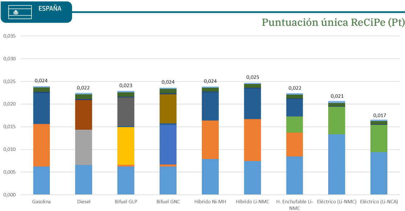
Figura 10 – Comparativa de impacto en cambio climático (kg CO 2 eq.) y puntuación única ReCiPe (impacto ambiental agregado) (Pt.) de un vehículo de tamaño medio, realizando un recorrido mixto de 100 km (15 km urbano, 85 km interurbano) por cada uno de los países del estudio: España, Reino Unido, Estados Unidos, Brasil y México. La escala del eje de ordenadas se ha igualado en todas las gráficas para facilitar su comparación. (continúa)
