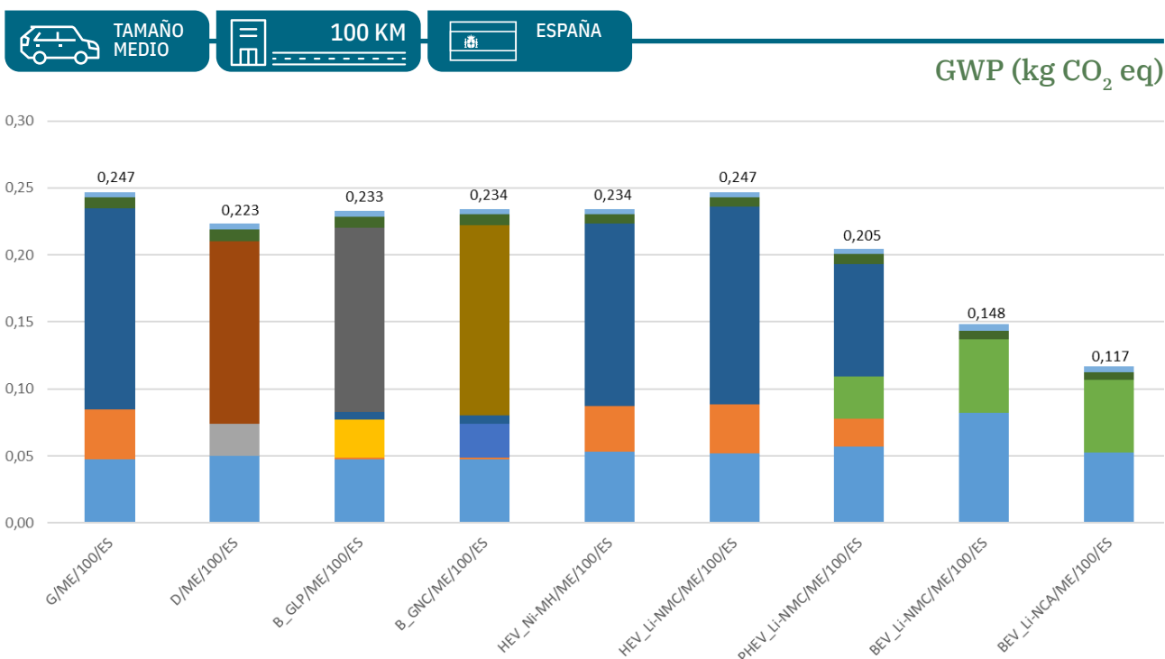
Gráfica 14 – Comparativa del impacto en cambio climático de las 9 tecnologías contempladas para un vehículo de tamaño medio (ME) realizando el recorrido mixto de 100 km, que circula por España (ES) (kg CO 2 eq.)
