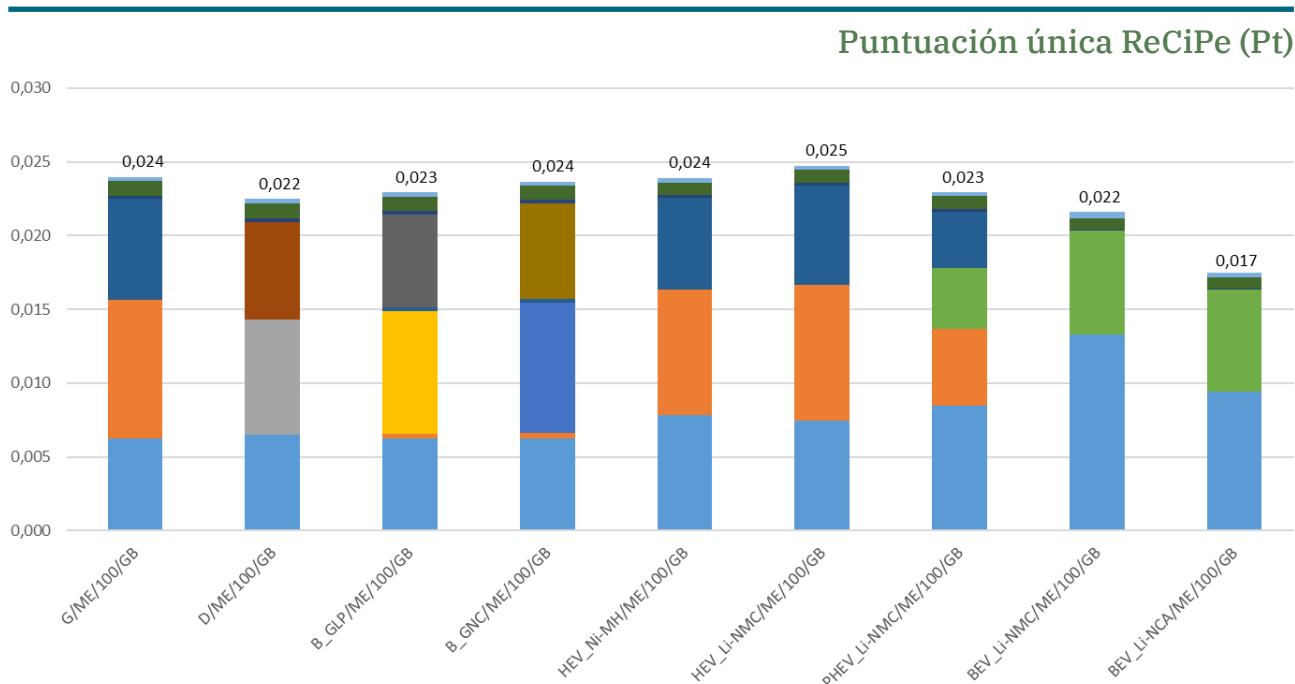
Gráfica 35 – Comparativa del impacto en puntuación única ReCiPe de las 9 tecnologías contempladas para un vehículo de tamaño mediano (ME) realizando el recorrido mixto de 100 km, que circula por Reino Unido (GB) (Pt)
