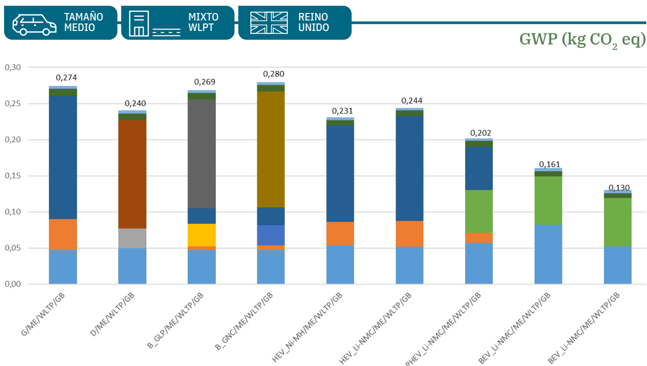
Gráfica 44 – Comparativa del impacto en cambio climático de las 9 tecnologías contempladas para un vehículo de tamaño mediano (ME) realizando el recorrido mixto WLTP, que circula por Reino Unido (GB) (kg CO 2 eq.)
