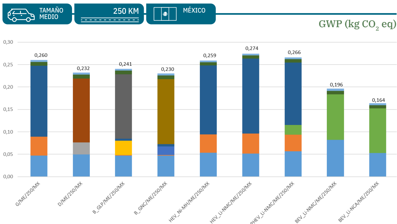
Gráfica 96 – Comparativa del impacto en cambio climático de las 9 tecnologías contempladas para un vehículo de tamaño mediano (ME) realizando el recorrido interurbano de 250 km, que circula por México (MX) (kg CO 2 eq.)
