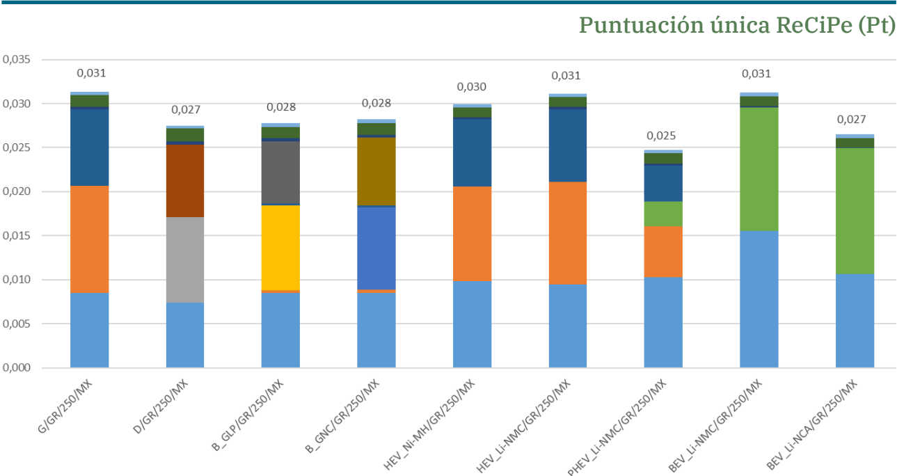
Gráfica 103 – Comparativa del impacto en puntuación única ReCiPe de las 9 tecnologías contempladas para un vehículo de tamaño grande (GR) realizando el recorrido interurbano de 250 km, que circula por México (MX) (Pt)
