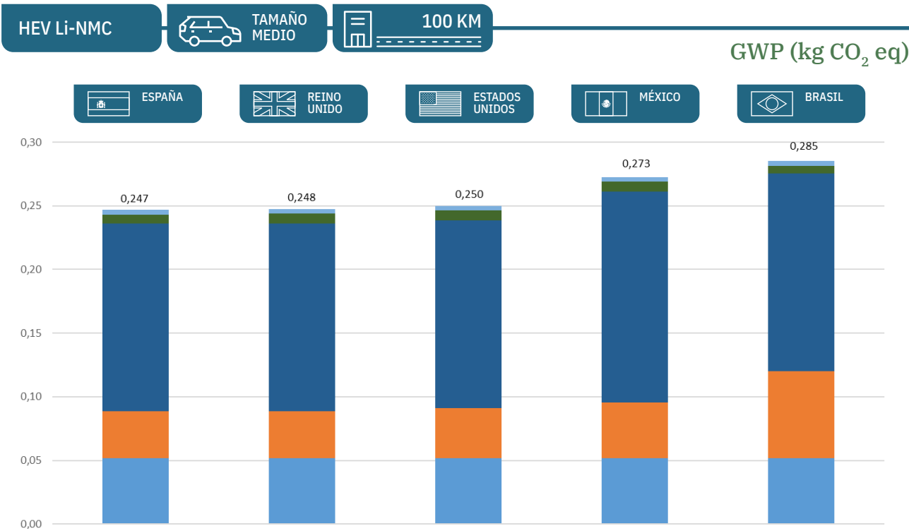
Gráfica 154 – Impacto en cambio climático de la influencia de cada país, para un vehículo híbrido HEV, con batería de ion Litio NMC, de tamaño mediano (ME), que realiza un recorrido mixto de 100 km (kg CO 2 eq.)
