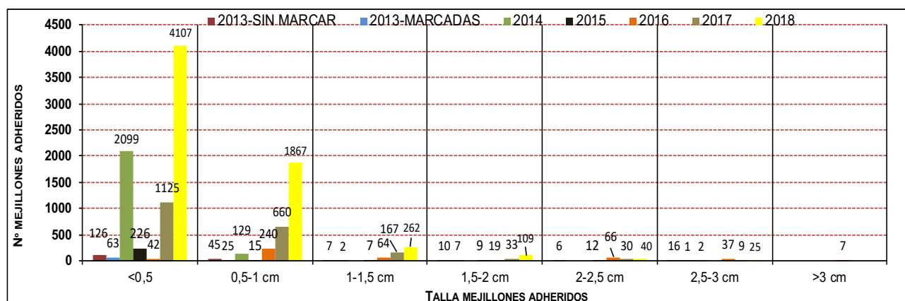
Figura 5 Número de mejillones cebra contabilizados para cada rango de tamaño sobre los 20 ejemplares de Anodonta anatina recapturados en la Zona A, a lo largo de los diferentes años de seguimiento.
