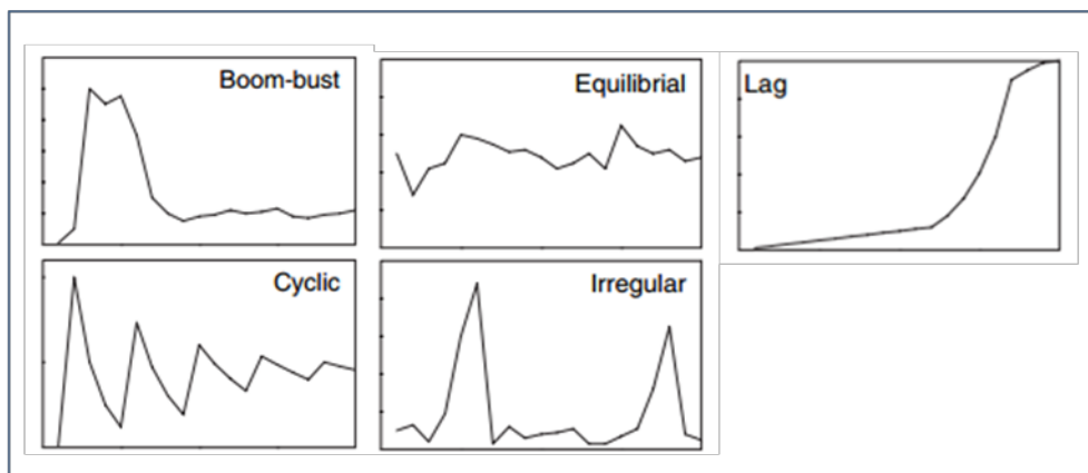
Figura 63 Tendencias a largo plazo que pueden experimentar las poblaciones de mejillón cebra (Strayer y Malcom, 2006).
