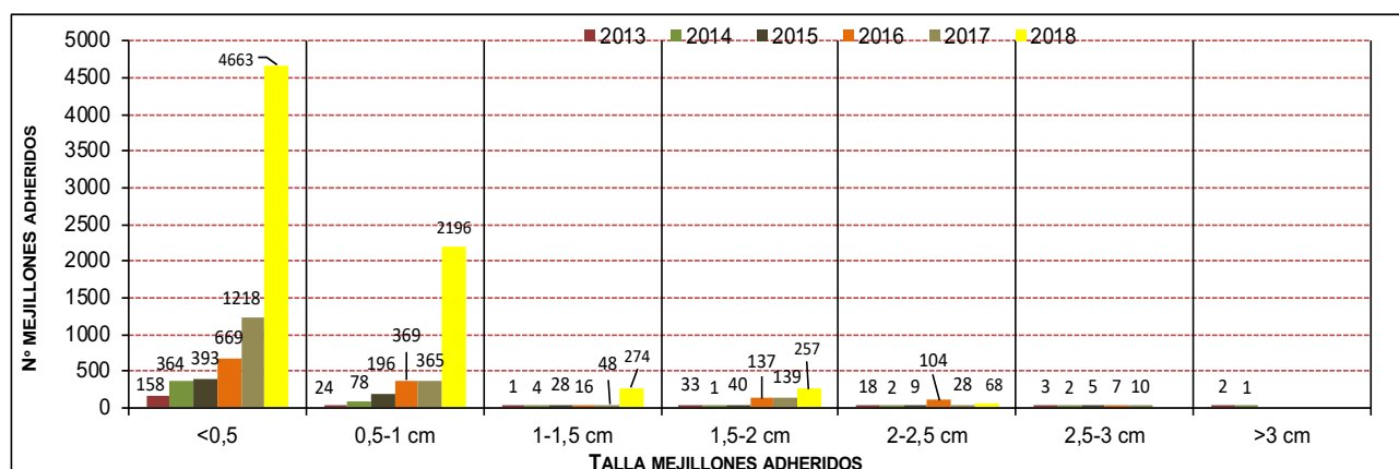
Figura 13 Gráfico. Número de mejillones cebra contabilizados para cada rango de tamaño sobre los 20 ejemplares de Anodonta anatina recapturados en la Zona C, a lo largo de los diferentes años de seguimiento.
