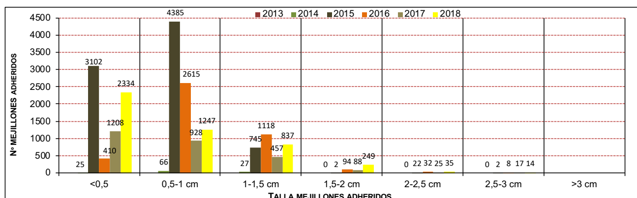
Figura 49 Gráfico. Número de mejillones cebra contabilizados para cada rango de tamaño sobre los 20 ejemplares de Anodonta anatina recapturados en la Zona Q, a lo largo de los diferentes años de seguimiento.
