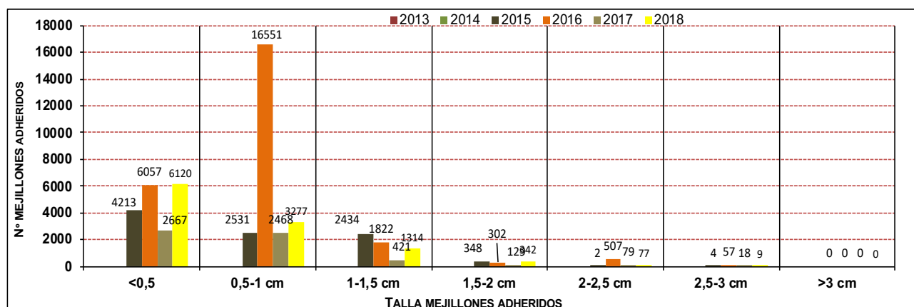
Figura 61 Gráfico. Número de mejillones cebra contabilizados para cada rango de tamaño sobre los 20 ejemplares de Anodonta anatina recapturados en la Zona V, a lo largo de los diferentes años de seguimiento.
