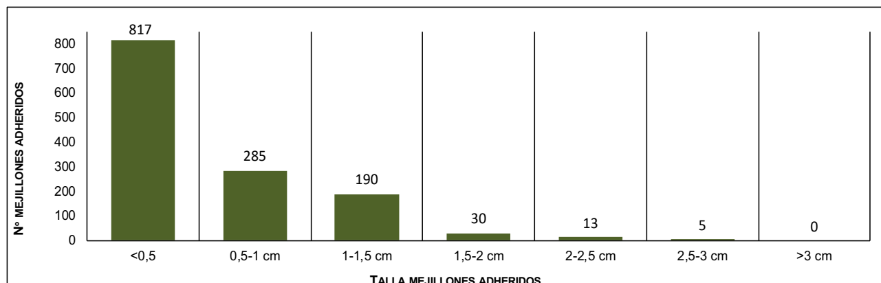
Figura 40 Gráfico. Número de mejillones cebra contabilizados para cada rango de tamaño sobre el total de los 20 ejemplares de Anodonta anatina recapturados en la Zona G. Año 2017.
