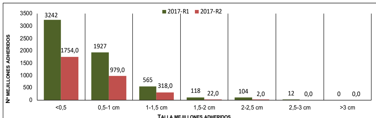
Figura 52 Gráfico. Número de mejillones cebra contabilizados para cada rango de tamaño sobre el total de los ejemplares de Anodonta anatina recapturados en las Zonas R1 y R2. Año 2018.
