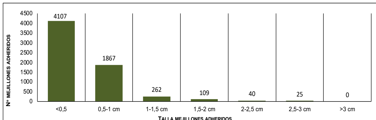
Figura 4 Número de mejillones cebra contabilizados para cada rango de tamaño sobre el total de los 20 ejemplares de Anodonta anatina recapturados en la Zona A. Año 2018.
