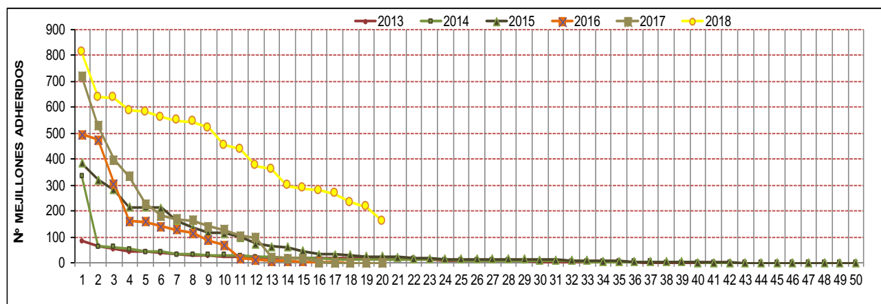
Figura 10 Número total de mejillones cebra contabilizados sobre cada una de las náyades analizadas en la Zona B2, a lo largo de los diferentes años de seguimiento.
