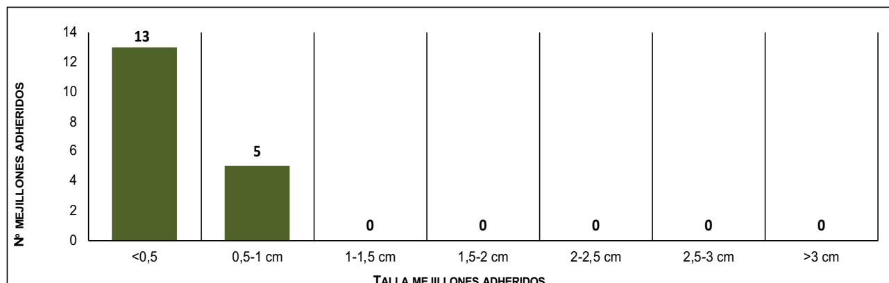
Figura 28 Número de mejillones cebra contabilizados para cada rango de tamaño sobre el total de los 20 ejemplares de Anodonta anatina recapturados en la Zona P. Año 2018.
