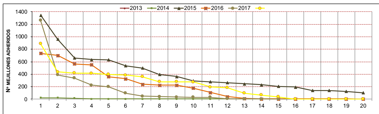
Figura 50 Gráfico. Número total de mejillones cebra contabilizados sobre cada una de las náyades analizadas en la Zona Q, a lo largo de los diferentes años de seguimiento.
