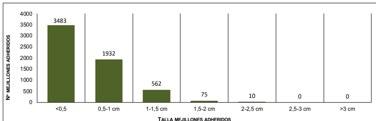
Figura 20 Gráfico. Número de mejillones cebra contabilizados para cada rango de tamaño sobre el total de los 5 ejemplares de Anodonta anatina recapturados en la Zona H. Año 2018.
