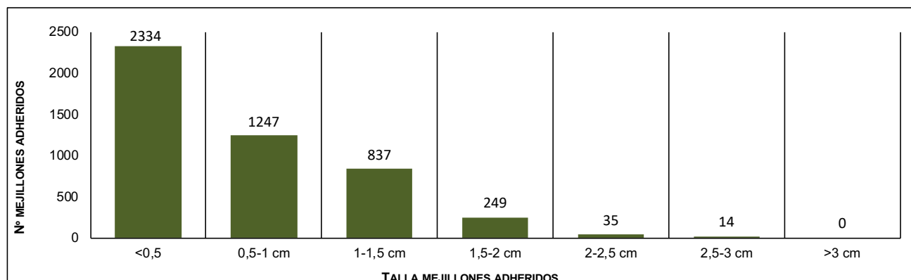
Figura 48 Gráfico. Número de mejillones cebra contabilizados para cada rango de tamaño sobre el total de los 20 ejemplares de Anodonta anatina recapturados en la Zona Q. Año 2018.
