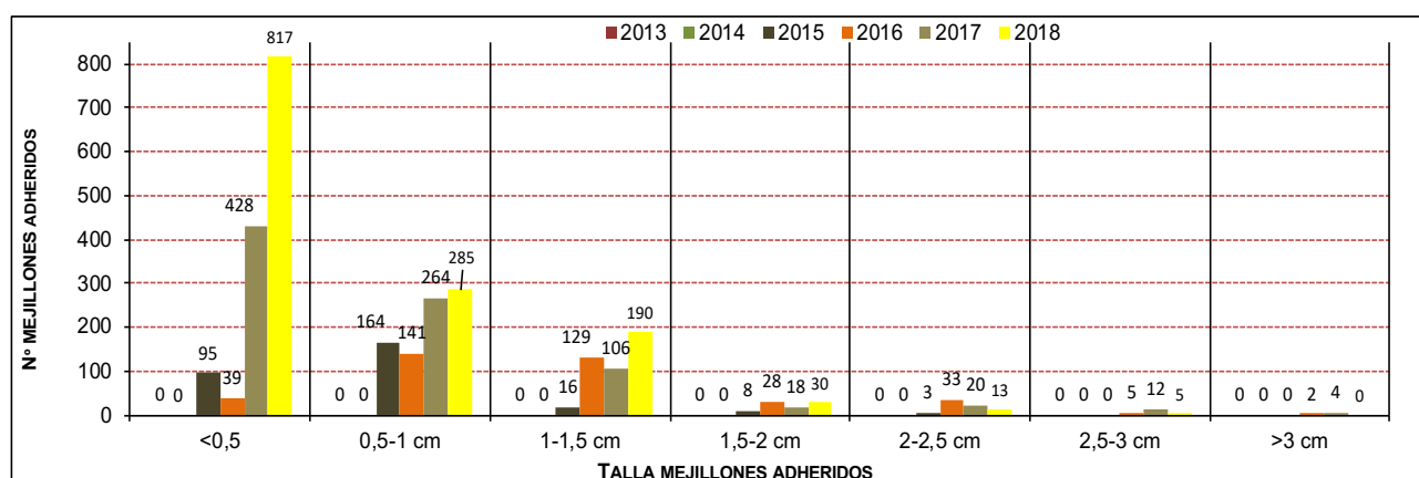
Figura 41 Gráfico. Número de mejillones cebra contabilizados para cada rango de tamaño sobre los 20 ejemplares de Anodonta anatina recapturados en la Zona G, a lo largo de los diferentes años de seguimiento.
