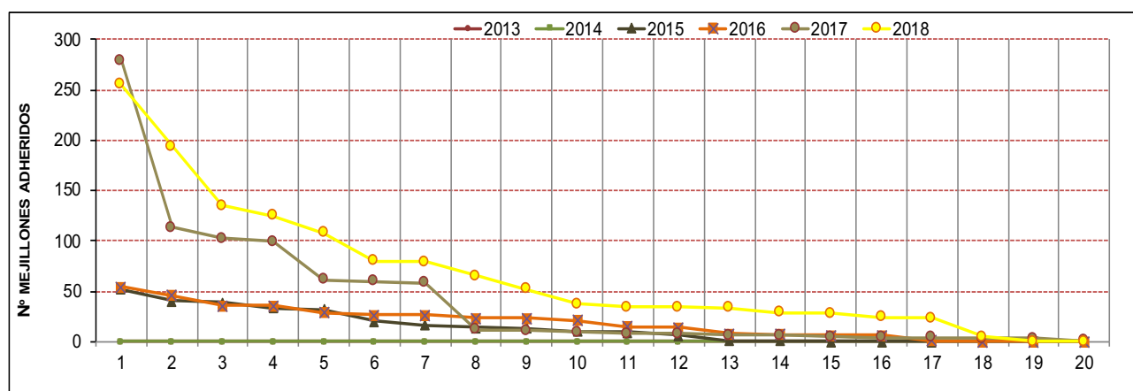
Figura 42 Gráfico. Número total de mejillones cebra contabilizados sobre cada una de las náyades analizadas en la Zona G, a lo largo de los diferentes años de seguimiento.
