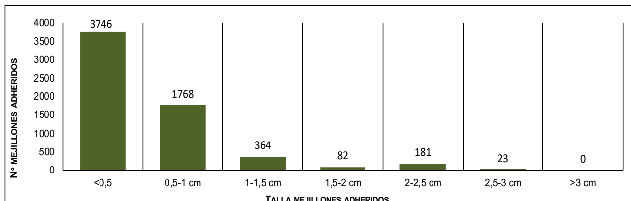
Figura 32 Gráfico. Número de mejillones cebra contabilizados para cada rango de tamaño sobre el total de los 20 ejemplares de Anodonta anatina recapturados en la Zona Q. Año 2018.
