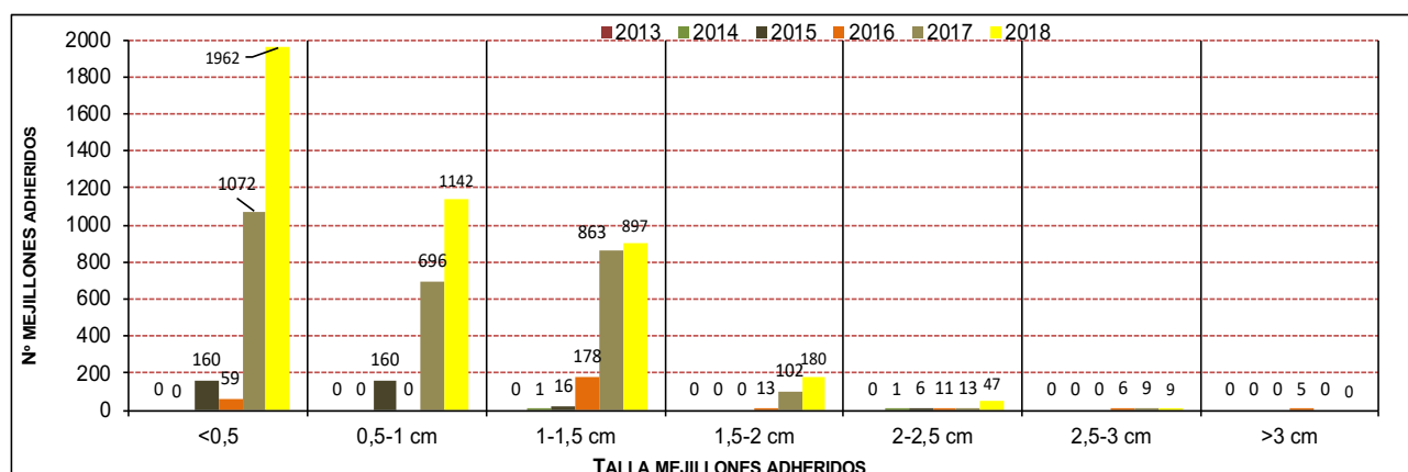
Figura 45 Gráfico. Número de mejillones cebra contabilizados para cada rango de tamaño sobre los 20 ejemplares de Anodonta anatina recapturados en la Zona G, a lo largo de los diferentes años de seguimiento.
