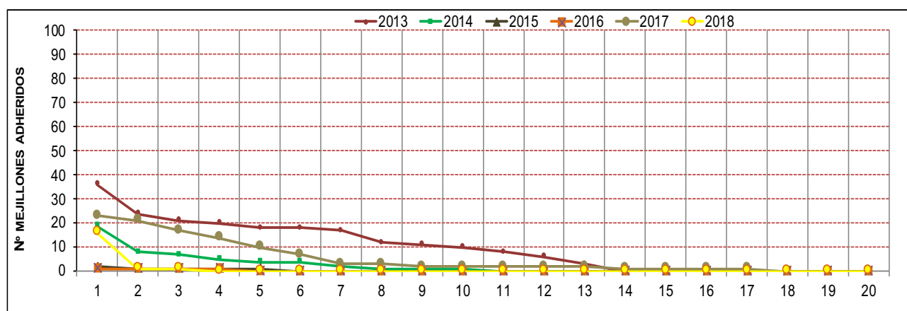
Figura 30 Número total de mejillones cebra contabilizados sobre cada una de las náyades analizadas en la Zona P, a lo largo de los diferentes años de seguimiento.
