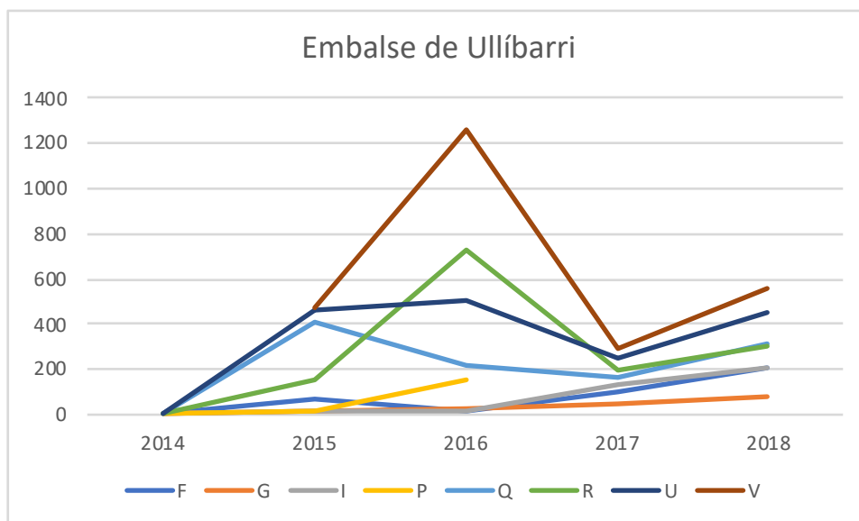
Figura 64 Tendencia que parece experimentar en el tiempo la población de mejillón cebra del embalse de Ullívarri, en base a los índices medios de fijación en cada una de las zonas de seguimiento.
