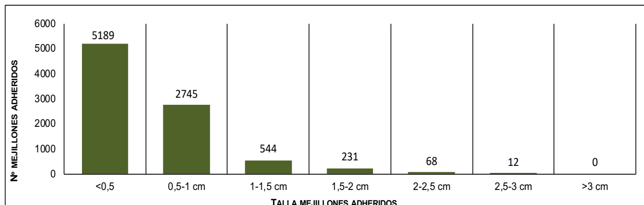
Figura 8 Gráfico. Número de mejillones cebra contabilizados para cada rango de tamaño sobre el total de los 20 ejemplares de Anodonta anatina recapturados en la Zona B2. Año 2018.
