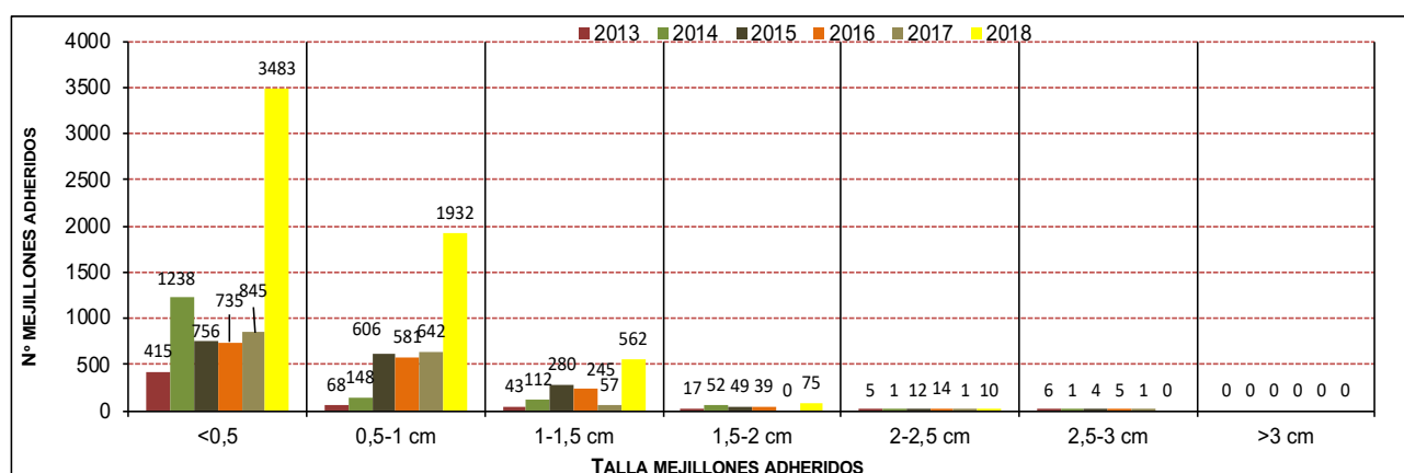
Figura 21 Gráfico. Número de mejillones cebra contabilizados para cada rango de tamaño sobre los 5 ejemplares de Anodonta anatina recapturados en la Zona H, a lo largo de los diferentes años de seguimiento.
