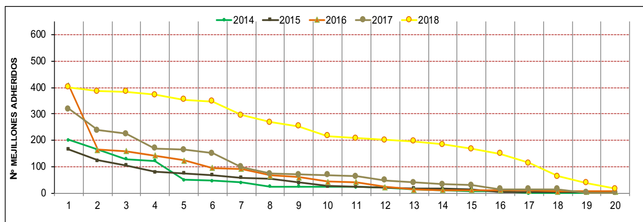
Figura 26 Gráfico. Número total de mejillones cebra contabilizados sobre cada una de las náyades analizadas en la Zona L, a lo largo de los diferentes años de seguimiento.
