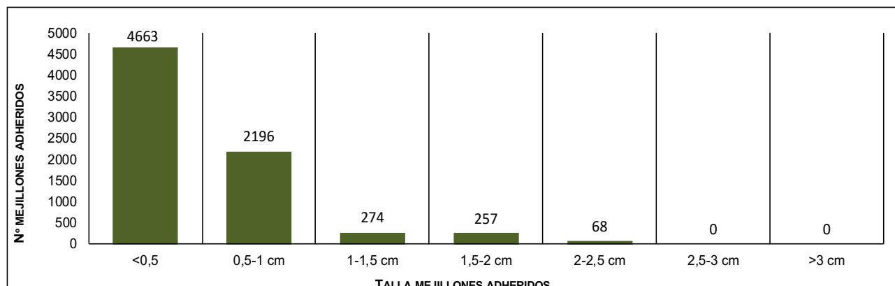
Figura 12 Gráfico. Número de mejillones cebra contabilizados para cada rango de tamaño sobre el total de los 20 ejemplares de Anodonta anatina recapturados en la Zona C. Año 2018.
