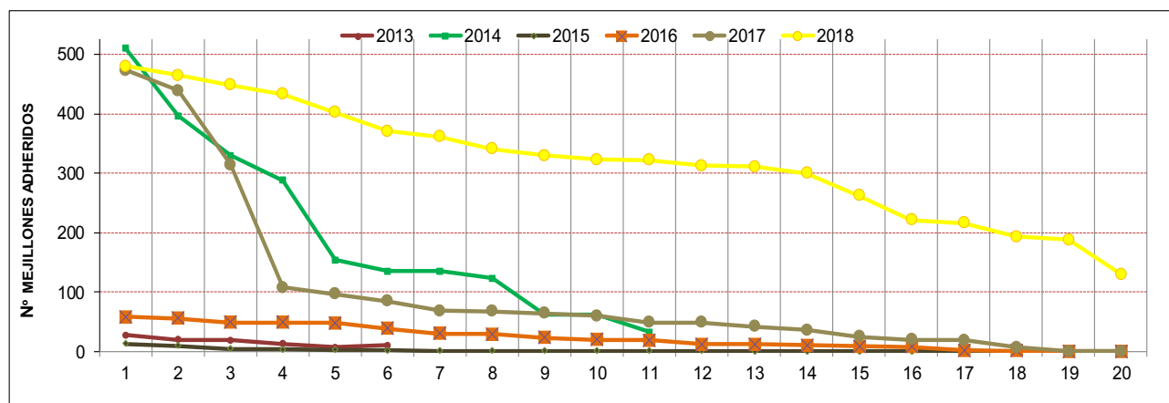
Figura 6 Número total de mejillones cebra contabilizados sobre cada una de las náyades analizadas en la Zona A, a lo largo de los diferentes años de seguimiento.
