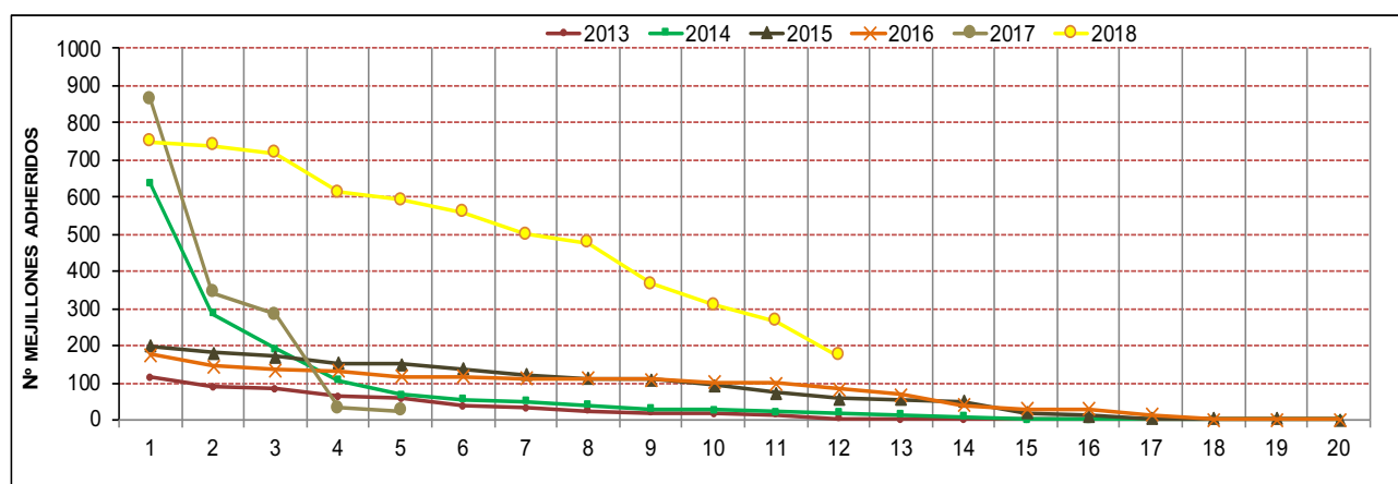
Figura 22 Gráfico. Número total de mejillones cebra contabilizados sobre cada una de las náyades analizadas en la Zona H, a lo largo de los diferentes años de seguimiento.
