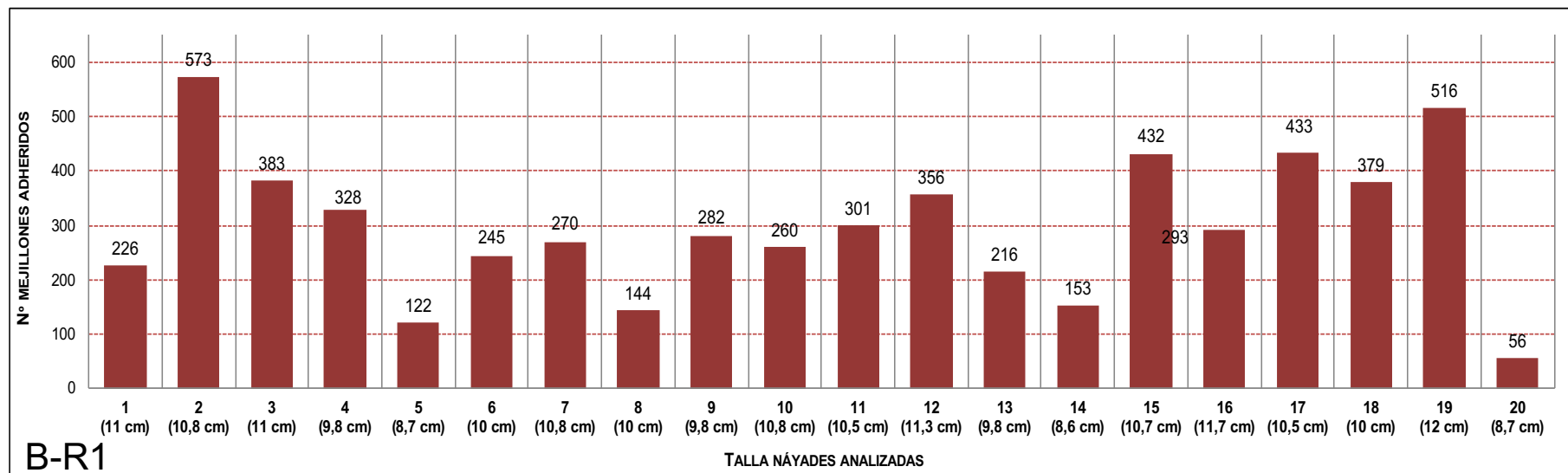
Figura 51. B Gráfico B: Número total de mejillones cebra contabilizados sobre cada uno de los 20 ejemplares de Anodonta anatina recapturados en las Zonas R1 y R2. Año 2018.
