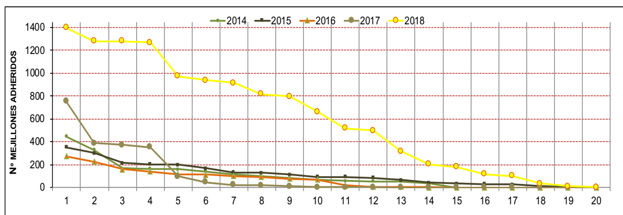
Figura 18 Gráfico. Número total de mejillones cebra contabilizados sobre cada una de las náyades analizadas en la Zona E, a lo largo de los diferentes años de seguimiento.
