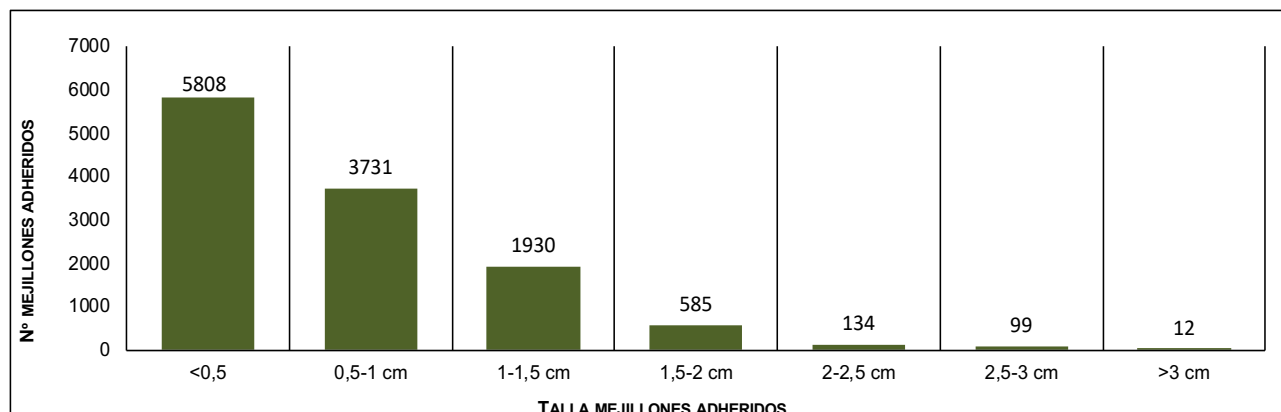
Figura 16 Gráfico. Número de mejillones cebra contabilizados para cada rango de tamaño sobre el total de los 15 ejemplares de Anodonta anatina recapturados en la Zona E. Año 2018.
