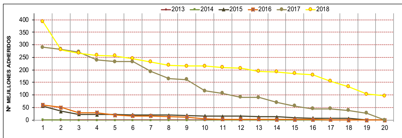
Figura 46 Gráfico. Número total de mejillones cebra contabilizados sobre cada una de las náyades analizadas en la Zona G, a lo largo de los diferentes años de seguimiento.
