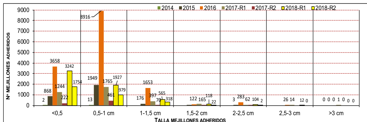
Figura 53 Gráfico. Número de mejillones cebra contabilizados para cada rango de tamaño sobre los ejemplares de Anodonta anatina recapturados en las Zonas R1 y R2, a lo largo de los diferentes años de seguimiento.
