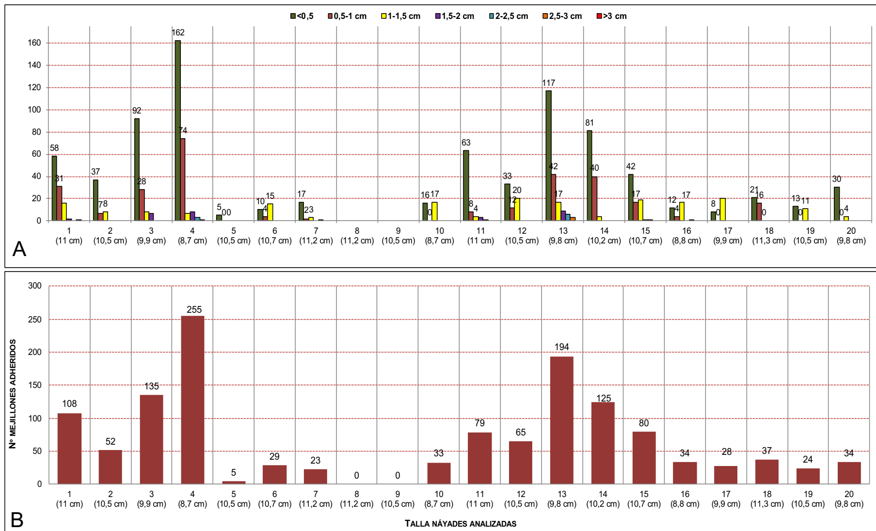
Figura 39 Gráfico A: Número de ejemplares de Dreissena polymorpha adheridos por clase de tamaño a cada uno de los 20 ejemplares de Anodonta anatina recapturados en la Zona G. Gráfico B: Número total de mejillones cebra contabilizados sobre cada uno de los 20 ejemplares de Anodonta anatina recapturados. Año 2018.
