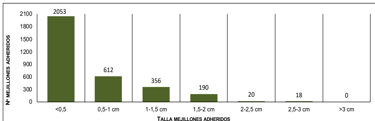
Figura 36 Gráfico. Número de mejillones cebra contabilizados para cada rango de tamaño sobre el total de los 20 ejemplares de Anodonta anatina recapturados en la Zona F. Año 2018.
