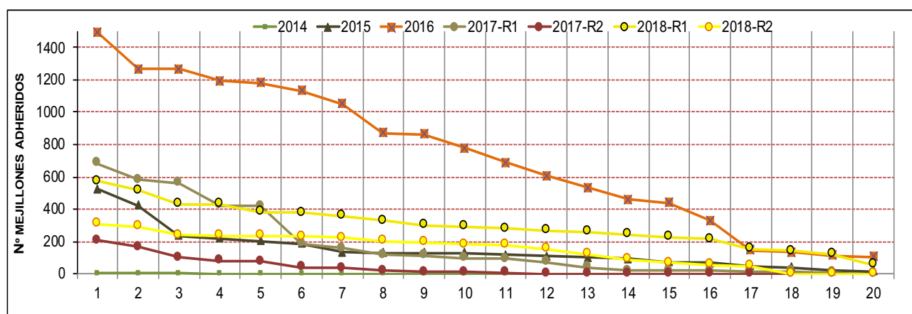
Figura 54 Gráfico. Número total de mejillones cebra contabilizados sobre cada una de las náyades analizadas en las Zonas R1 y R2, a lo largo de los diferentes años de seguimiento.
