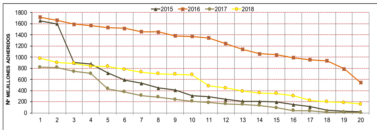
Figura 62 Gráfico. Número total de mejillones cebra contabilizados sobre cada una de las náyades analizadas en la Zona V, a lo largo de los diferentes años de seguimiento.
