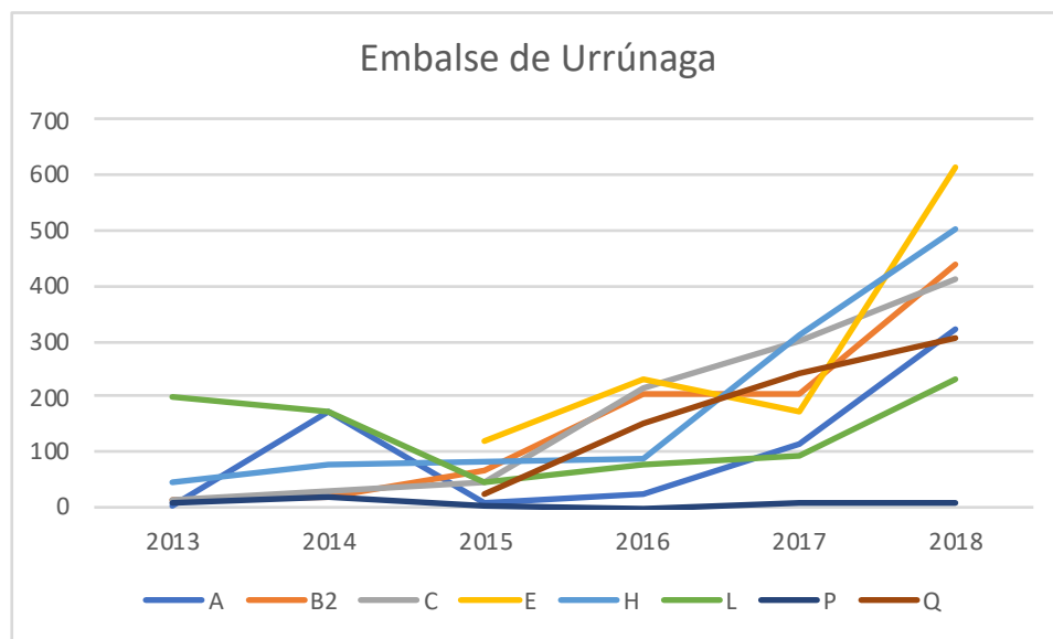
Figura 65 Tendencia que parece experimentar en el tiempo la población de mejillón cebra del embalse de Urrúnaga, en base a los índices medios de fijación en cada una de las zonas de seguimiento.
