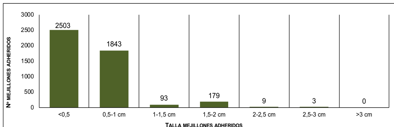
Figura 24 Gráfico. Número de mejillones cebra contabilizados para cada rango de tamaño sobre el total de los 20 ejemplares de Anodonta anatina recapturados en la Zona L. Año 2018.
