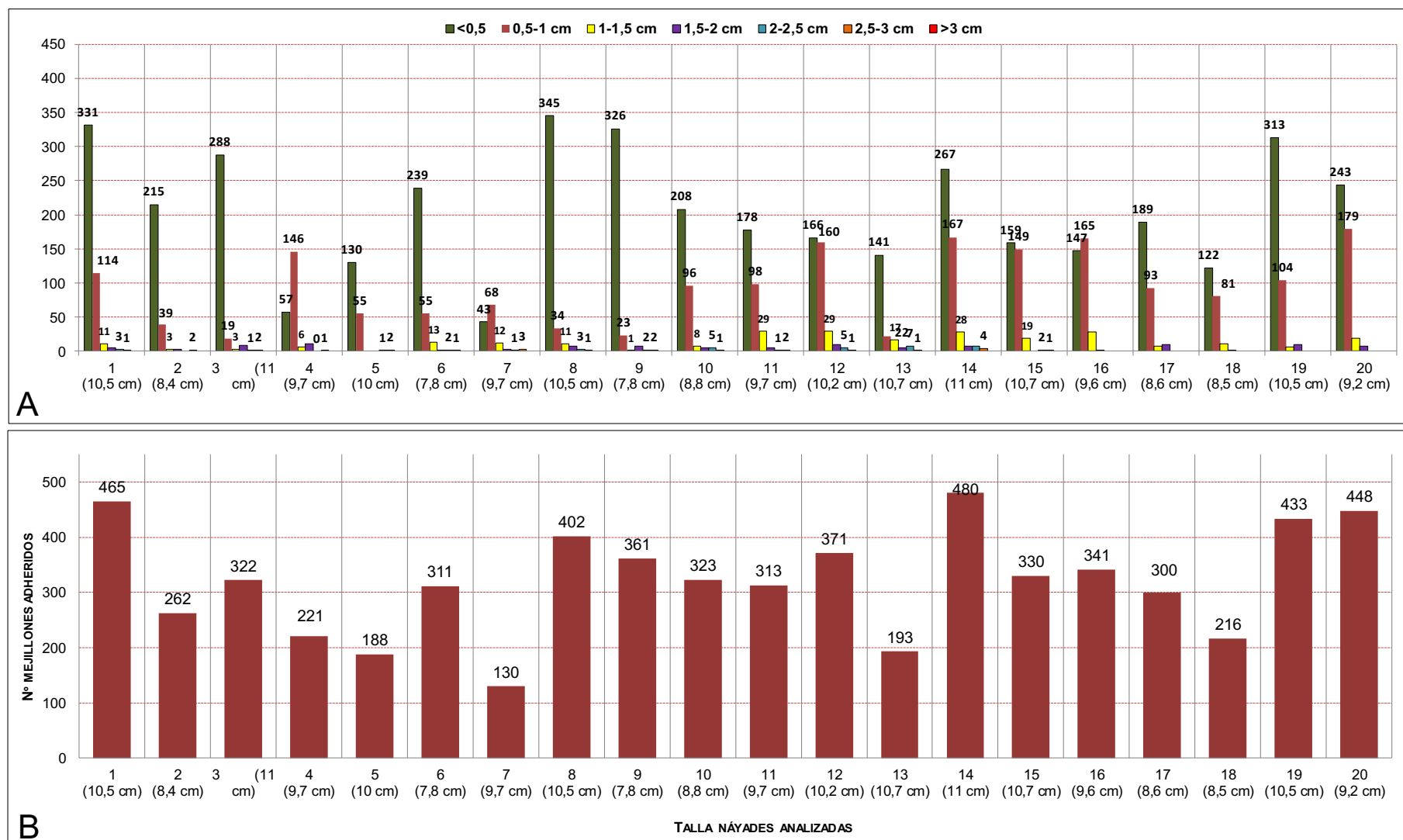
Figura 3 Gráfico A: Número de ejemplares de Dreissena polymorpha adheridos por clase de tamaño a cada uno de los 20 ejemplares de Anodonta anatina recapturados en la Zona A. Gráfico B: Número total de mejillones cebra contabilizados sobre cada uno de los 20 ejemplares de Anodonta anatina recapturados. Año 2018.
