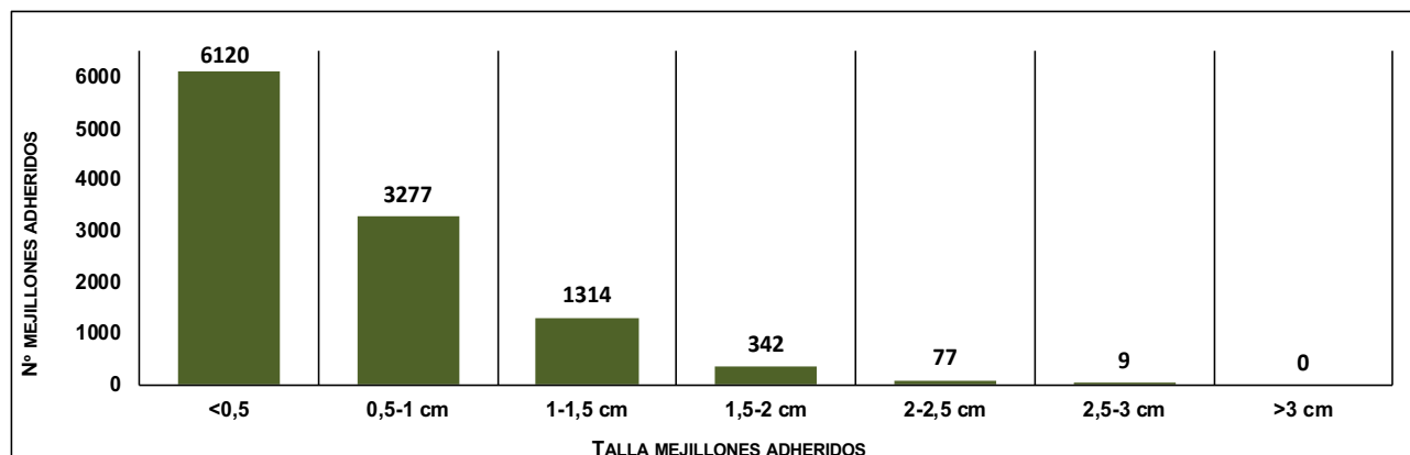
Figura 60 Gráfico. Número de mejillones cebra contabilizados para cada rango de tamaño sobre el total de los 20 ejemplares de Anodonta anatina recapturados en la Zona V. Año 2018.
