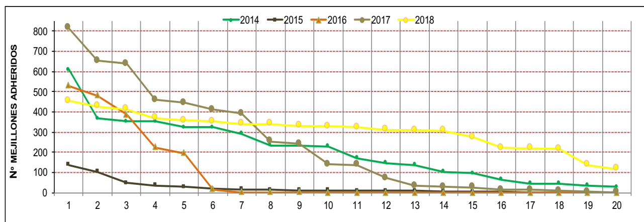
Figura 34 Gráfico. Número total de mejillones cebra contabilizados sobre cada una de las náyades analizadas en la Zona Q, a lo largo de los diferentes años de seguimiento.
