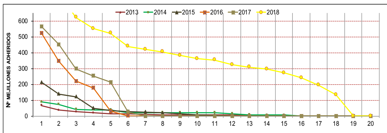
Figura 14 . Número total de mejillones cebra contabilizados sobre cada una de las náyades analizadas en la Zona C, a lo largo de los diferentes años de seguimiento.
