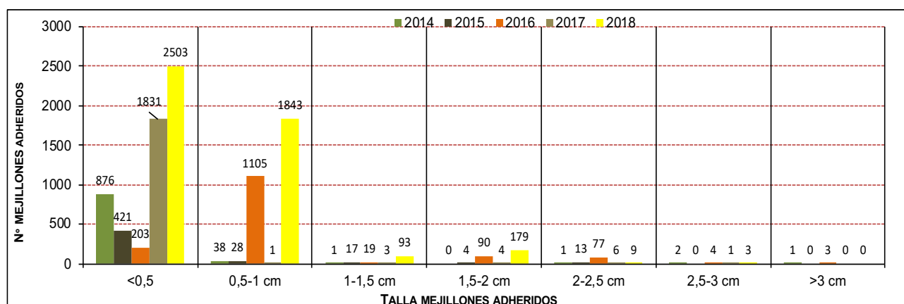
Figura 25 Gráfico. Número de mejillones cebra contabilizados para cada rango de tamaño sobre los 20 ejemplares de Anodonta anatina recapturados en la Zona L, a lo largo de los diferentes años de seguimiento.
