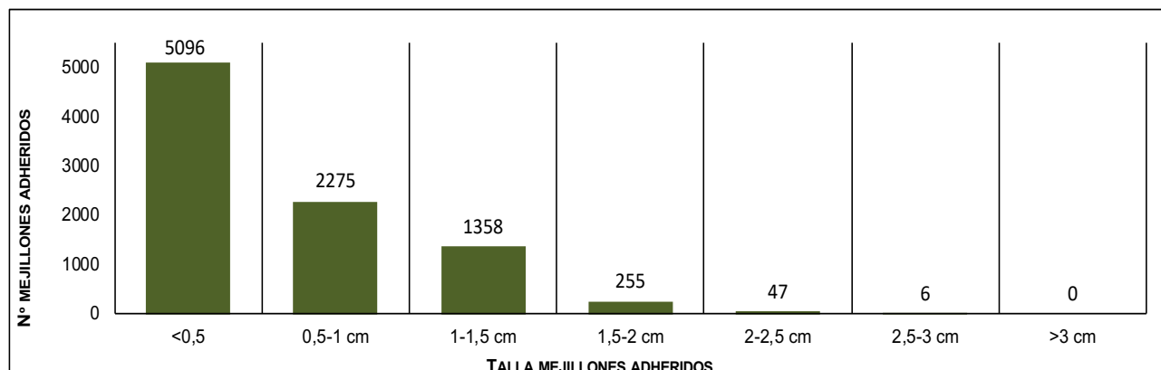
Figura 56 Gráfico. Número de mejillones cebra contabilizados para cada rango de tamaño sobre el total de los 20 ejemplares de Anodonta anatina recapturados en la Zona U. Año 2018.
