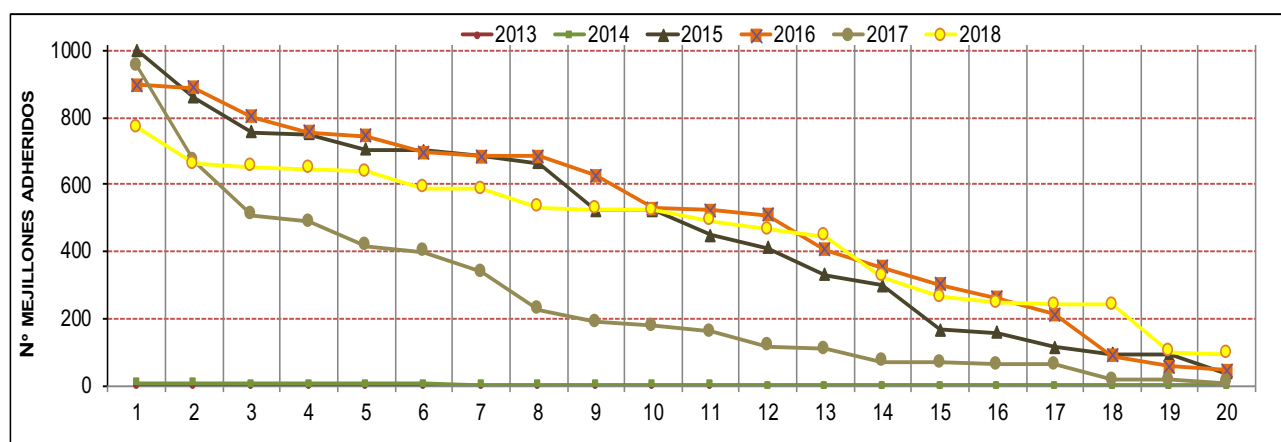
Figura 58 Gráfico. Número total de mejillones cebra contabilizados sobre cada una de las náyades analizadas en la Zona U, a lo largo de los diferentes años de seguimiento.
