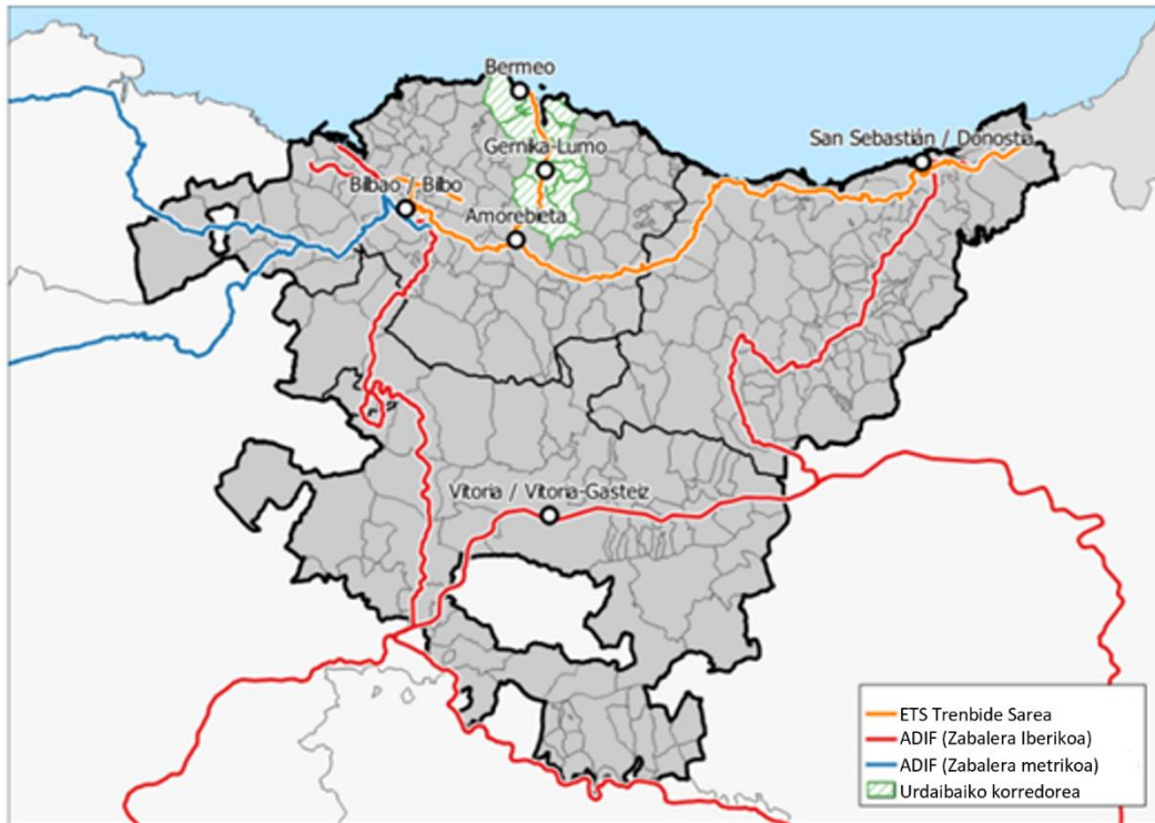
86. irudia. EAEko Trenbide sarea Iturria: Berezko lanketa
