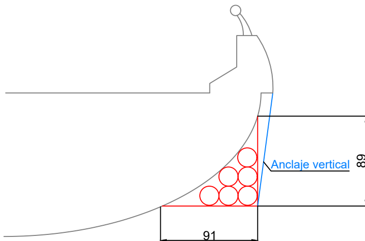
CANALIZACIÓN ADOSADA A PUENTE (6 TUBOS 200MM Ø) COTAS EN CM
