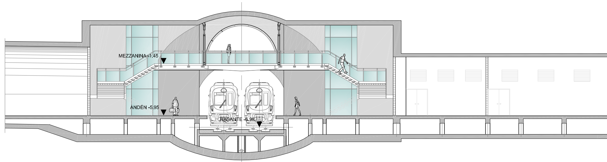
SECCIÓN A-A E(A1): 1/100
