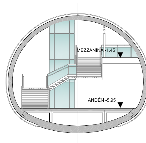
SECCIÓN B-B E(A1): 1/100
