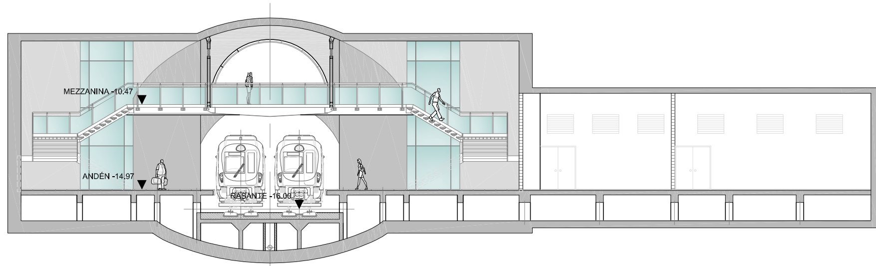
SECCIÓN A-A E(A1): 1/100
