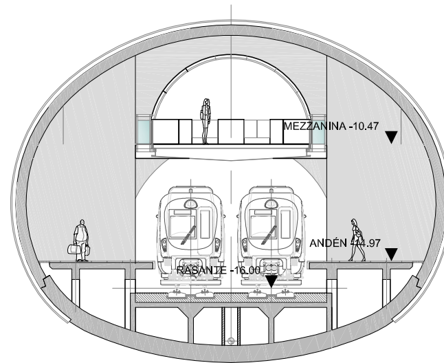
SECCIÓN C-C E(A1): 1/100
