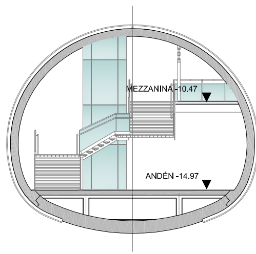
SECCIÓN B-B E(A1): 1/100
