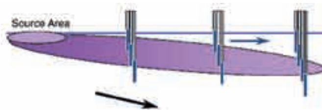
Figura 4.6. Planteamiento de una red de control multinivel.
