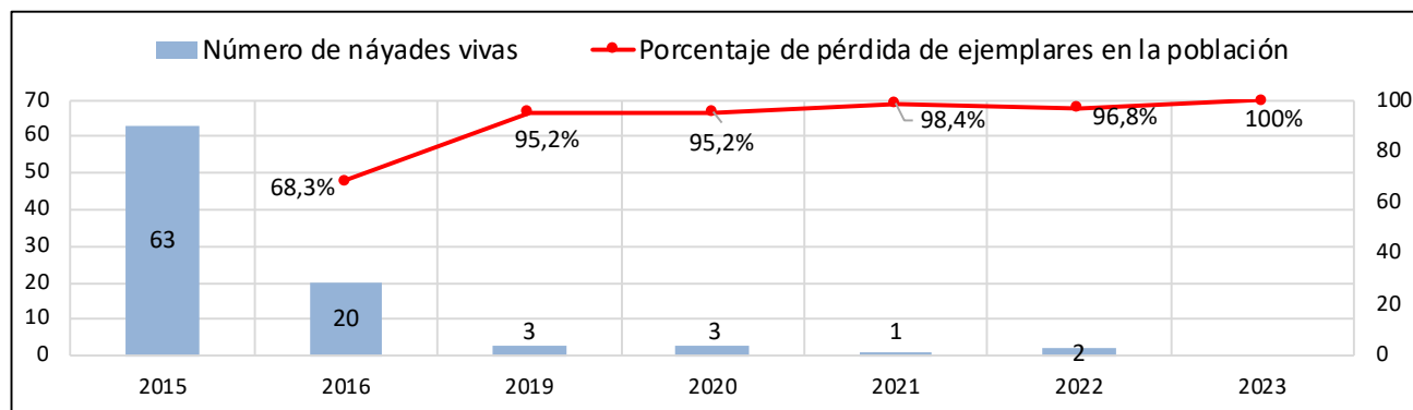
Figura 61 Número de náyades detectadas en la Zona V en los muestreos realizados durante los diferentes años de seguimiento y porcentaje estimado de pérdida de individuos en esta población a lo largo de este tiempo
