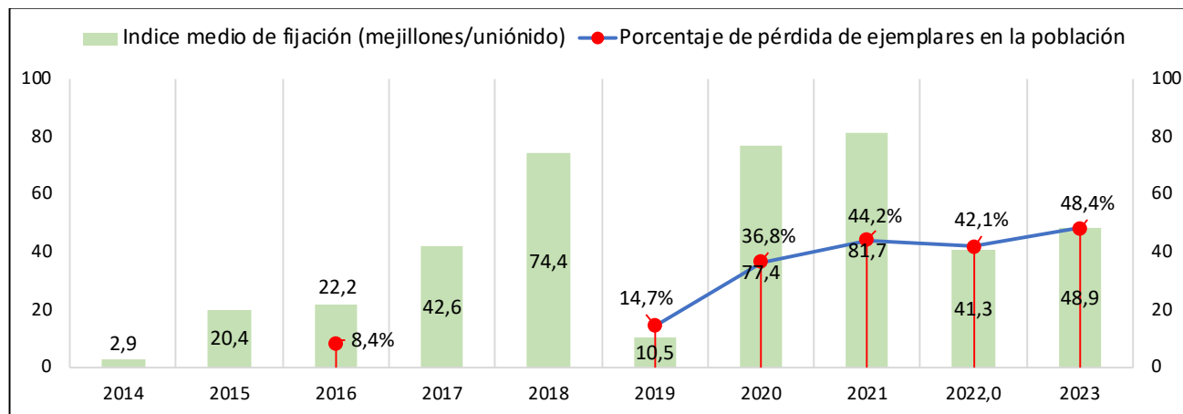
Figura 40 Índice medio de fijación (mejillones/uniónido) estimado en los muestreos realizados durante los años 2014-2023 en la Zona G, y porcentaje estimado de pérdida de individuos en esta población durante los muestreos realizados en 2016, 2019, 2020, 2021, 2022 y 2023
