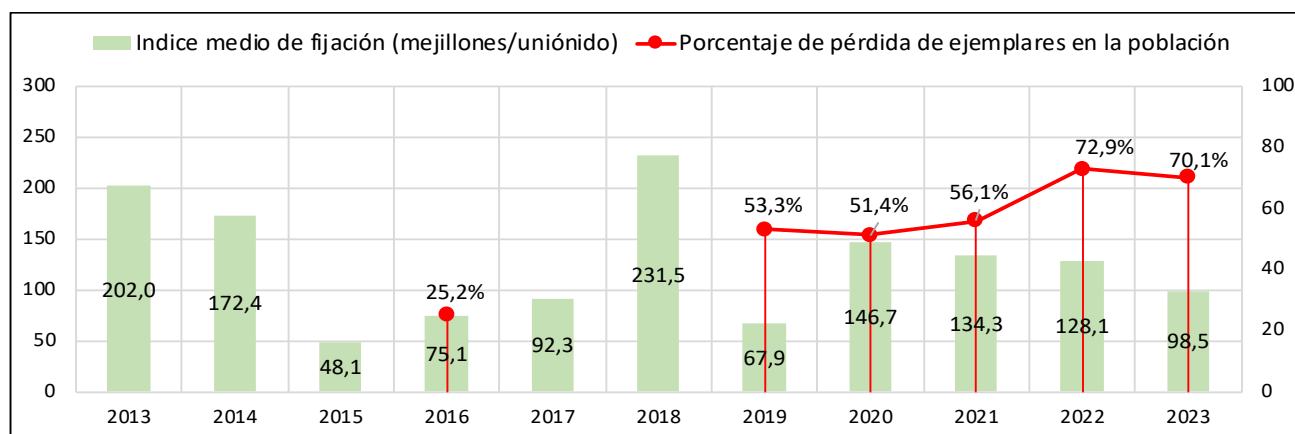
Figura 20 Índice medio de fijación (mejillones/uniónido) estimado en los muestreos realizados durante los años 2013-2023 en la Zona L, y porcentaje estimado de pérdida de individuos en esta población durante los muestreos realizados en 2016, 2019, 2020, 2021, 2022 y 2023
