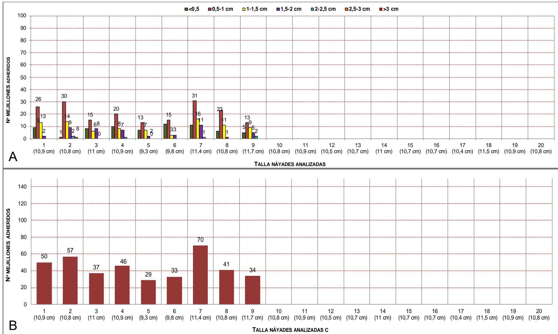
Figura 57 Gráfico A: Número de ejemplares de Dreissena polymorpha adheridos por clase de tamaño a cada uno de los 20 ejemplares de Anodonta anatina recapturados en la Zona R2. Gráfico B: Número total de mejillones cebra contabilizados sobre cada uno de los 20 ejemplares de Anodonta anatina recapturados. Año 2023.
