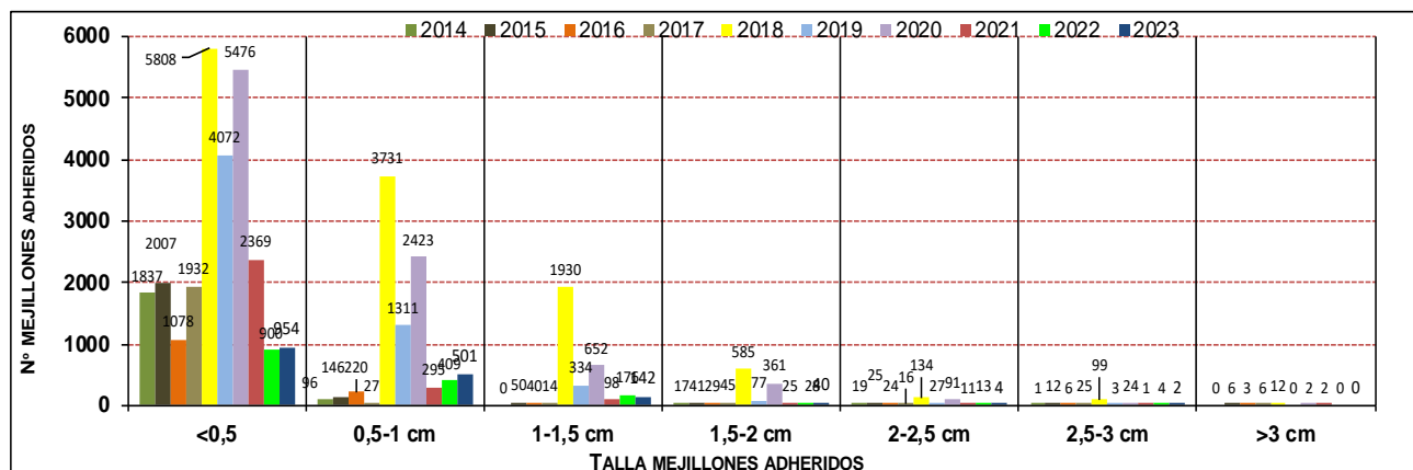
Figura 17 Gráfico. Número de mejillones cebra contabilizados para cada rango de tamaño sobre los 15 ejemplares de Anodonta anatina recapturados en la Zona E a lo largo de los diferentes años de seguimiento.
