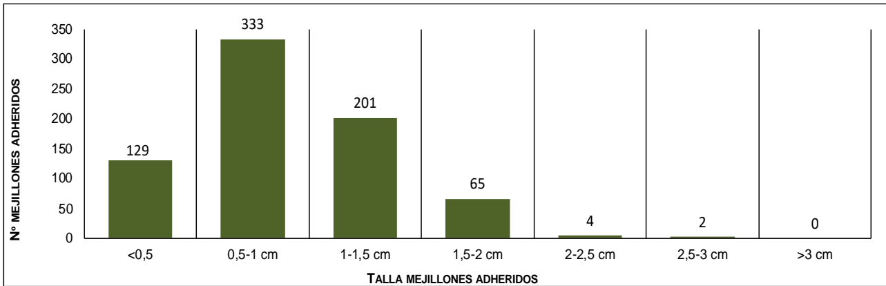
Figura 42 Gráfico. Número de mejillones cebra contabilizados para cada rango de tamaño sobre el total de los 20 ejemplares de Anodonta anatina recapturados en la Zona G. Año 2023.
