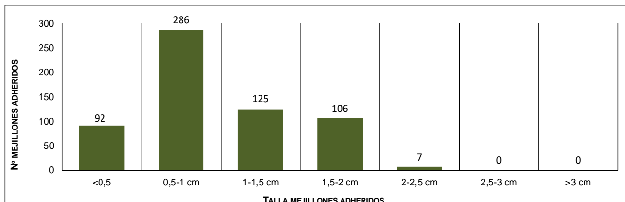
Figura 48 Gráfico. Número de mejillones cebra contabilizados para cada rango de tamaño sobre el total de los 20 ejemplares de Anodonta anatina recapturados en la Zona I. Año 2023.
