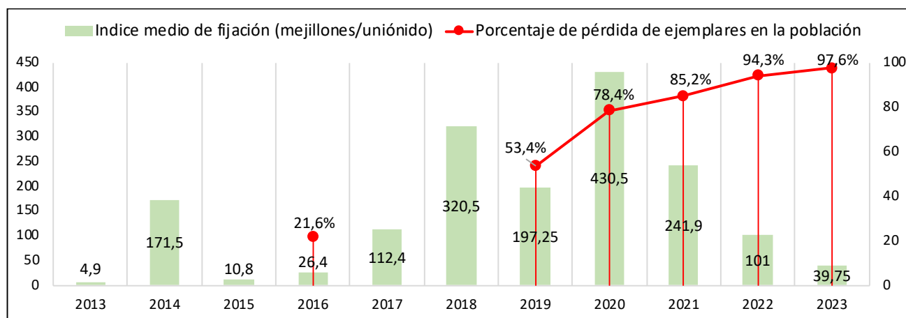
Figura 2 Índice medio de fijación (mejillones/uniónimo) estimado en los muestreos realizados durante los años 2013-2023 en la Zona A, y porcentaje estimado de pérdida de individuos en esta población durante los muestreos realizados en 2016, 2019, 2020, 2021, 2022 y 2023.
