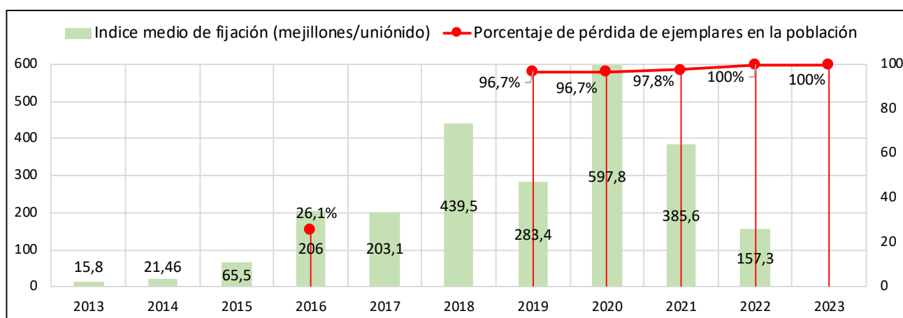
Figura 10 Índice medio de fijación (mejillones/uniónido) estimado en los muestreos realizados durante los años 2013-2022 en la Zona B2, y porcentaje estimado de pérdida de individuos en esta población durante los muestreos realizados en 2016, 2019, 2020, 2021, 2022 y 2023
