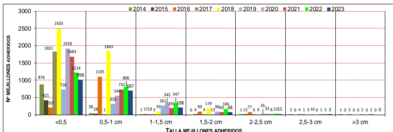
Figura 23 Gráfico. Número de mejillones cebra contabilizados para cada rango de tamaño sobre los 20 ejemplares de Anodonta anatina recapturados en la Zona L a lo largo de los diferentes años de seguimiento.
