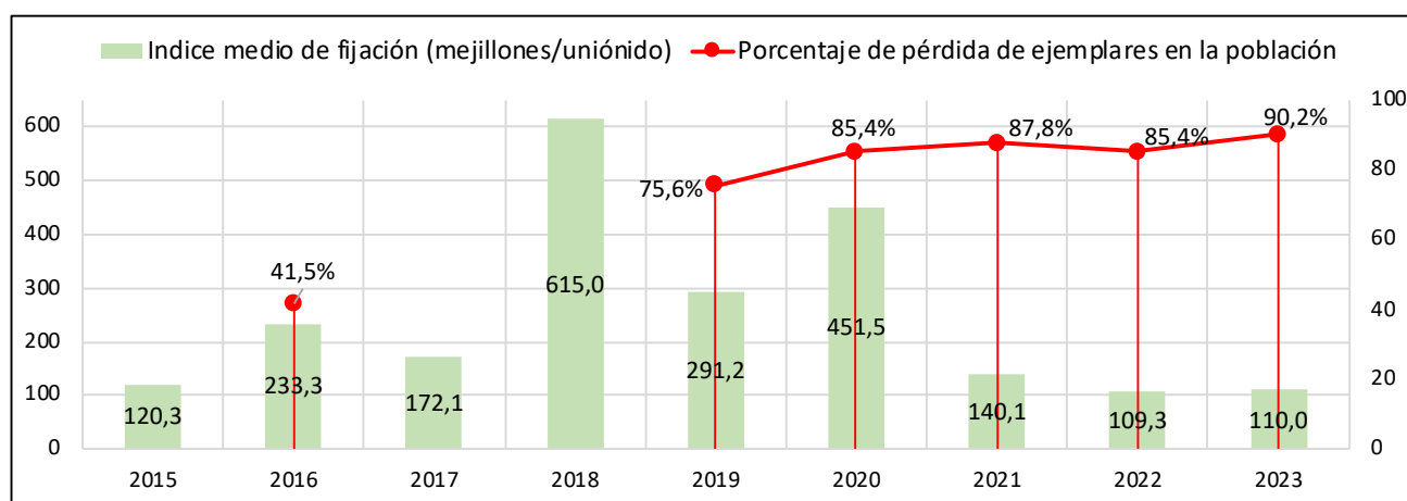
Figura 14 Índice medio de fijación (mejillones/uniónido) estimado en los muestreos realizados durante los años 2015-2023 en la Zona E, y porcentaje estimado de pérdida de individuos en esta población durante los muestreos realizados en 2016, 2019, 2020, 2021, 2022 y 2023
