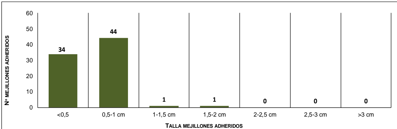
Figura 26 Número de mejillones cebra contabilizados para cada rango de tamaño sobre el total de los 20 ejemplares de Anodonta anatina recapturados en la Zona P. Año 2023.
