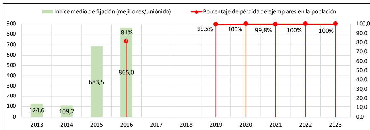
Figura 8 Índice medio de fijación (mejillones/uniónido) estimado en los muestreos realizados durante los años 2013-2016 en la Zona B1, y porcentaje estimado de pérdida de individuos en esta población durante los muestreos realizados en 2016, 2019, 2020, 2021, 2022 y 2023
