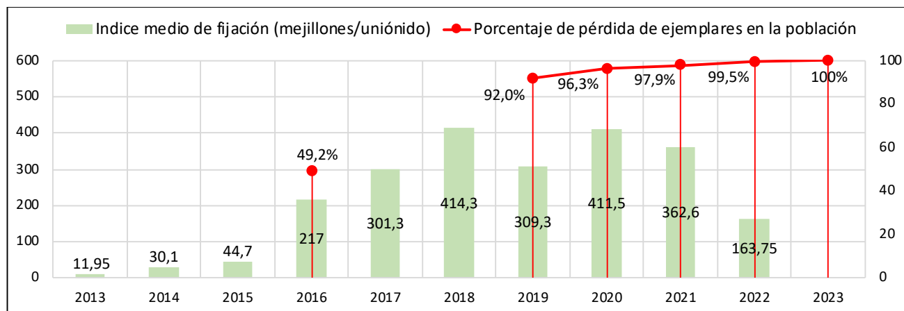
Figura 12 Índice medio de fijación (mejillones/uniónido) estimado en los muestreos realizados durante los años 2013-2022 en la Zona C, y porcentaje estimado de pérdida de individuos en esta población durante los muestreos realizados en 2016, 2019, 2020, 2021, 2022 y 2023
