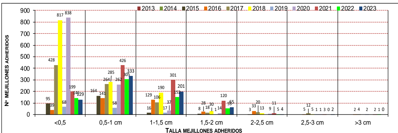
Figura 43 Gráfico. Número de mejillones cebra contabilizados para cada rango de tamaño sobre los 20 ejemplares de Anodonta anatina recapturados en la Zona G a lo largo de los diferentes años de seguimiento.
