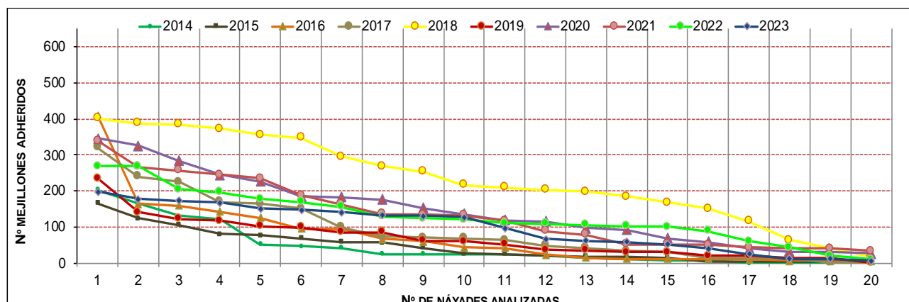
Figura 24 Gráfico. Número total de mejillones cebra contabilizados sobre cada una de las náyades analizadas en la Zona L, a lo largo de los diferentes años de seguimiento.
