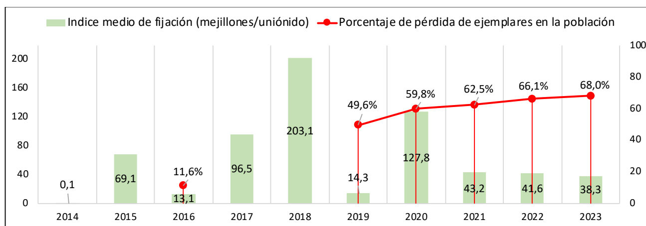
Figura 34 Índice medio de fijación (mejillones/uniónido) estimado en los muestreos realizados durante los años 2014-2023 en la Zona F, y porcentaje estimado de pérdida de individuos en esta población durante los muestreos realizados en 2016, 2019, 2020, 2021, 2022 y 2023
