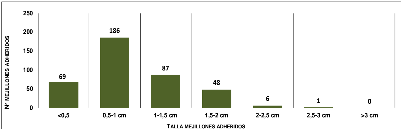
Figura 58 Gráfico. Número de mejillones cebra contabilizados para cada rango de tamaño sobre el total de los ejemplares de Anodonta anatina recapturados en la Zona R2. Año 2023.
