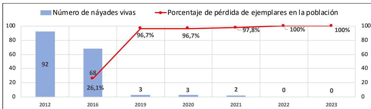
Figura 9 Número de náyades detectadas en la Zona B2 en los muestreos realizados durante los diferentes años de seguimiento y porcentaje estimado de pérdida de individuos en esta población a lo largo de este tiempo
