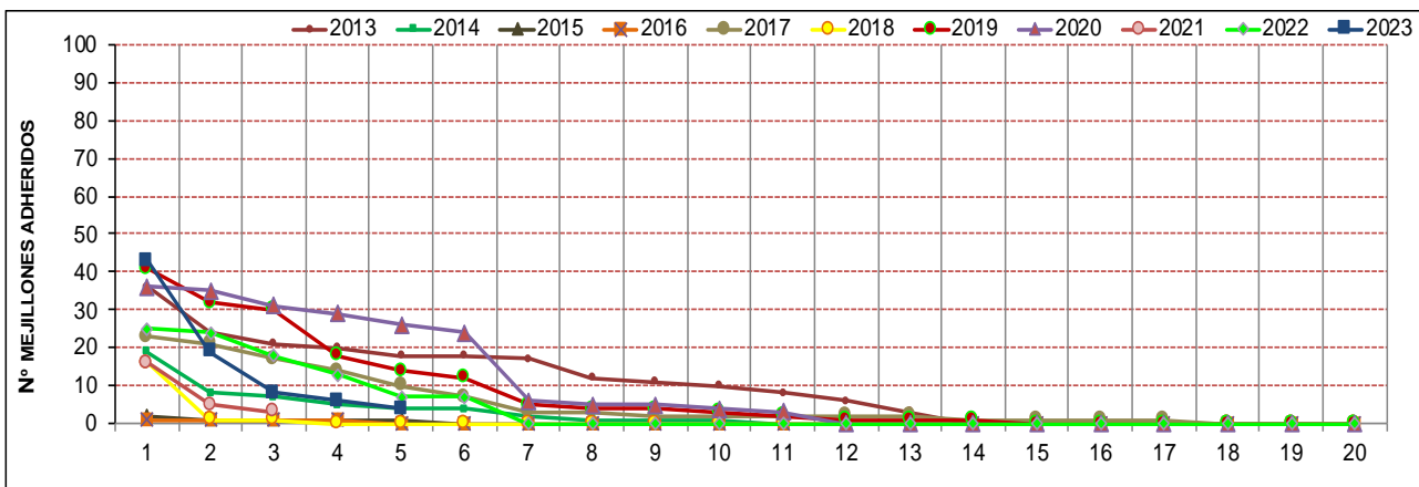
Figura 28 Número total de mejillones cebra contabilizados sobre cada una de las náyades analizadas en la Zona P a lo largo de los diferentes años de seguimiento.
