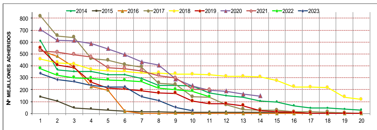
Figura 32 Número total de mejillones cebra contabilizados sobre cada una de las náyades analizadas en la Zona Q a lo largo de los diferentes años de seguimiento.
