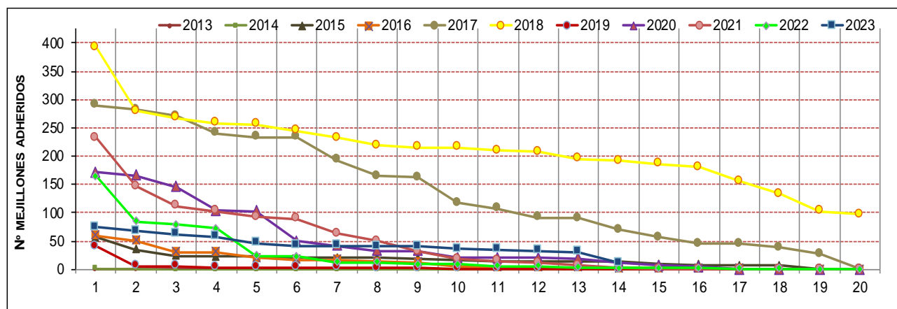
Figura 50 Gráfico. Número total de mejillones cebra contabilizados sobre cada una de las náyades analizadas en la Zona I a lo largo de los diferentes años de seguimiento.
