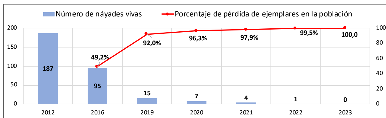
Figura 11 Número de náyades detectadas en la Zona C en los muestreos realizados durante los diferentes años de seguimiento y porcentaje estimado de pérdida de individuos en esta población a lo largo de este tiempo
