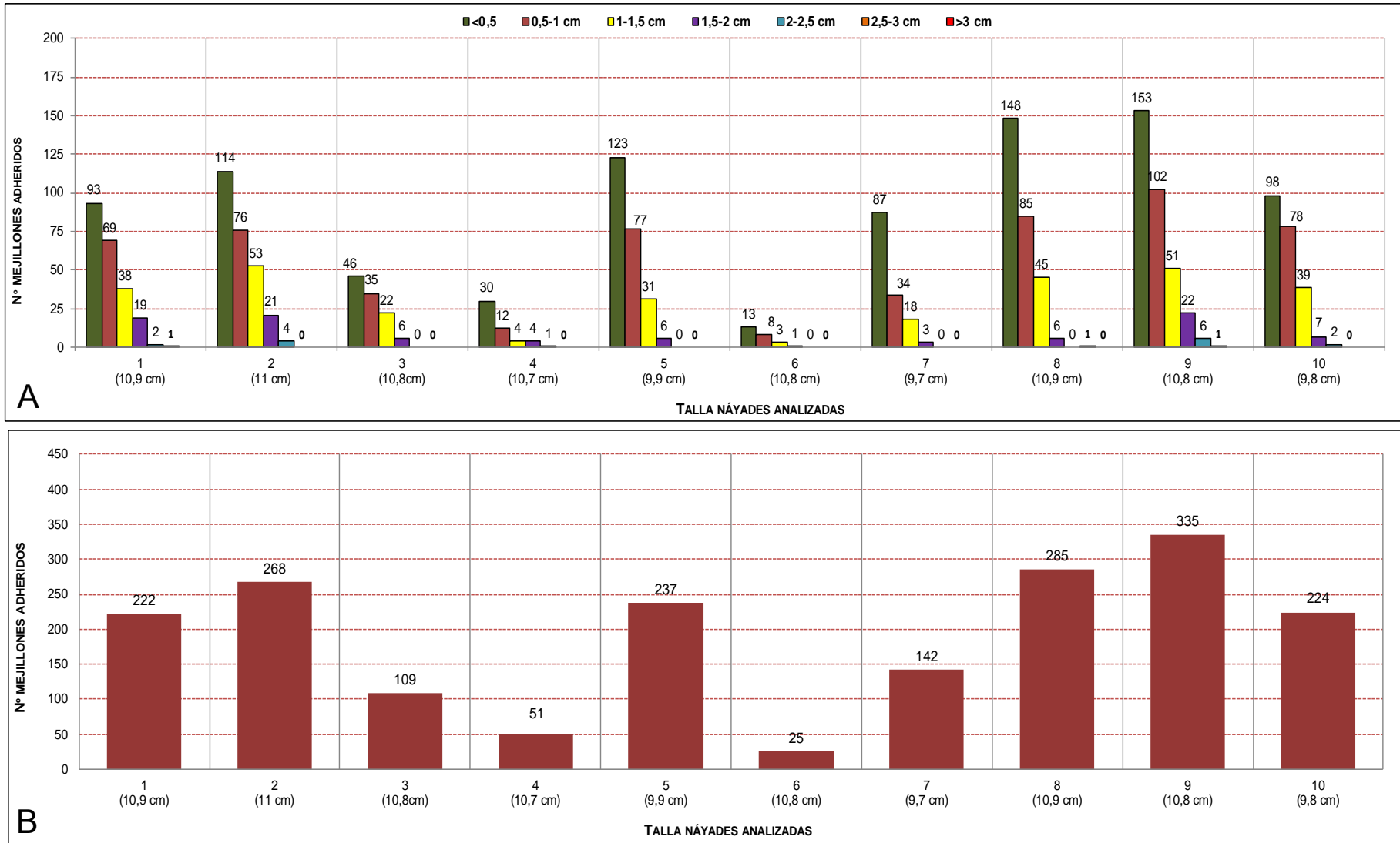
Figura 29 Gráfico A: Número de ejemplares de Dreissena polymorpha adheridos por clase de tamaño a cada uno de los 10 ejemplares de Anodonta anatina recapturados en la Zona Q. Gráfico B: Número total de mejillones cebra contabilizados sobre cada uno de los 11 ejemplares de Anodonta anatina recapturados. Año 2023.
