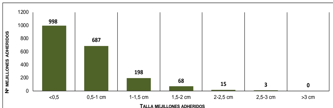
Figura 22 Gráfico. Número de mejillones cebra contabilizados para cada rango de tamaño sobre el total de los 20 ejemplares de Anodonta anatina recapturados en la Zona L. Año 2023.
